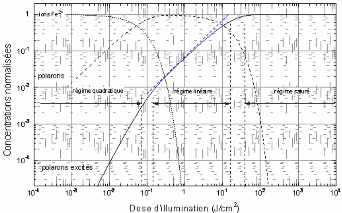
FIG. 4.4: Concentrations normalisées obtenues à la fin de l'impulsion laser, calculées dans le cadre du modèle à deux centres, à 532nm. Sections efficaces : 5 \times 10^{-18} \text{ cm}^2 pour l'ion fer, 5 \times 10^{-20} \text{ cm}^2 pour l'excitation du polron (valeur arbitraire inférieure au majorant donné par l'équation (4.36)).
