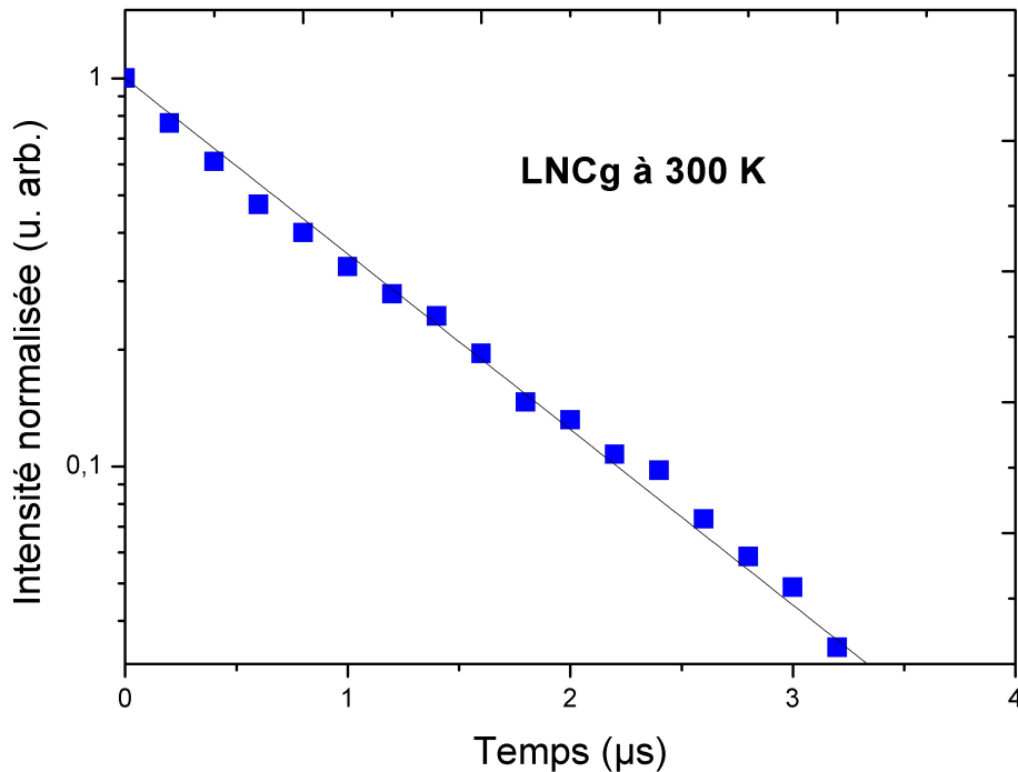
FIG. 3.25: Déclin de temps de vie du polaron dans le LN Cg à la température ambiante à 860\text{ nm} ( \lambda_{excitatrice} = 532\text{ nm} )
