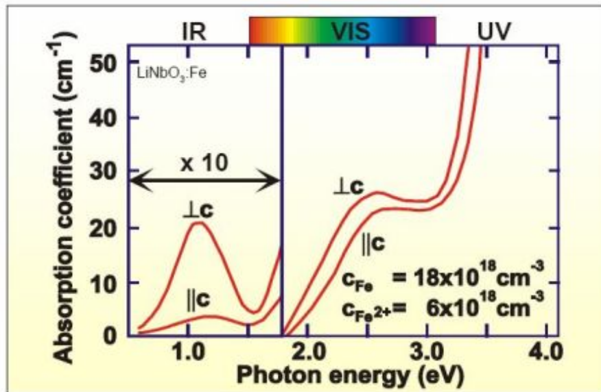
FIG. 1.13: Spectre d'absorption optique pour LN :Fe (342wt.ppm) réduit
