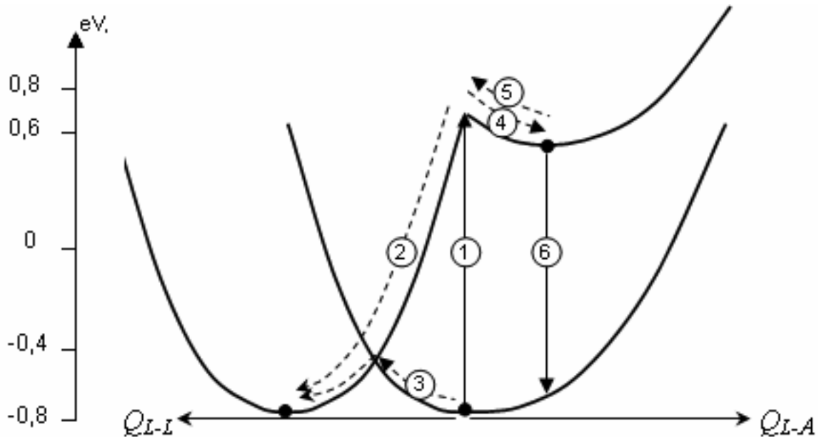
FIG. 4.5: Représentation schématique du diagramme de configuration du polaron lié Nb_{Li}^{4+} . Les flèches en trait plein représentent les transitions optiques, celles en trait interrompu les transitions assistées par les phonons
