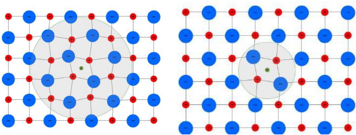
FIG. 2.2: Grand polaron (à gauche) et petit polaron (à droite)
