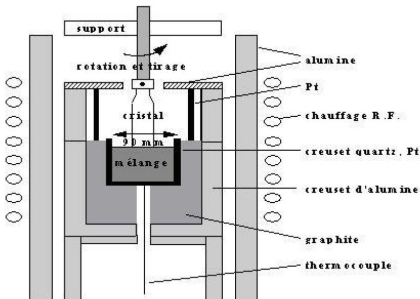
FIG. 1.3: Montage expérimental du tirage Czochralski
