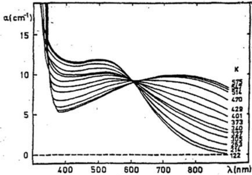
FIG. 2.8: Le changement d'absorption de 2.5eV (500nm) à 1.6eV (760nm), attribué à dissociation thermique du bipolaron dans le LN non dopé chimiquement réduit [2]
