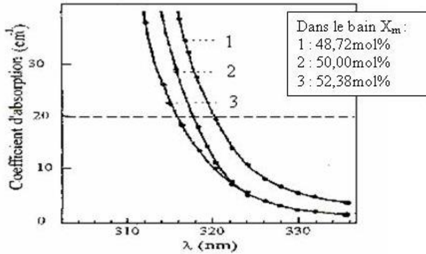
FIG. 1.9: Absorption optique fondamentale des échantillons de compositions différentes d'après Földvari et al. [38] 1 : X_c=48,57\text{mol}\% ; 2 : X_c=48,95\text{mol}\% ; 3 : X_c=49,40\text{mol}\%
