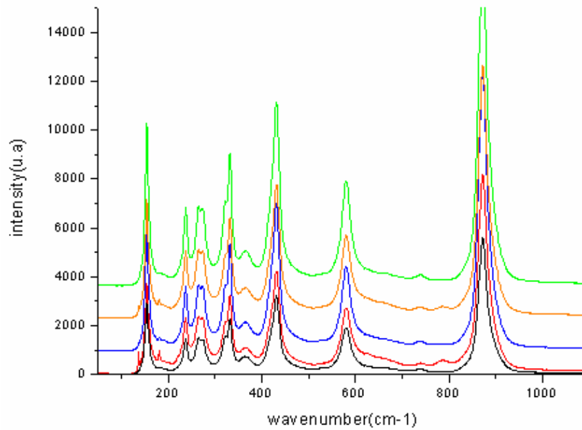
FIG. C.6: Spectres Raman au long d'un guide (à la surface) (Configuration Z(YX)Z, laser \lambda = 633\text{nm} , réseau 1800\text{ tr/mm} , temps d'acquisition 10\text{s} et température ambiante)
