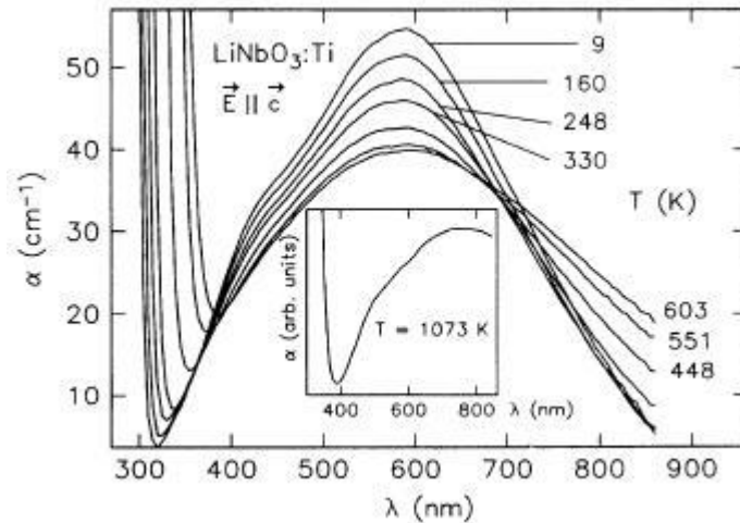
FIG. 1.14: Absorption du LN :Ti en fonction de la température (D'après Thiemann et al. [1]).
