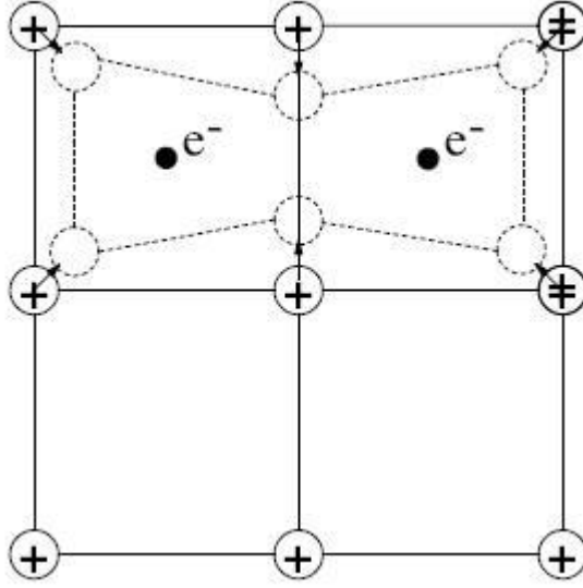
FIG. 2.3: Bipolaron
