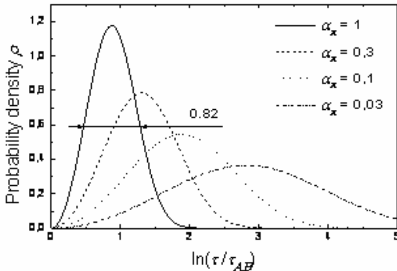
FIG. B.2: Probabilité des densités
