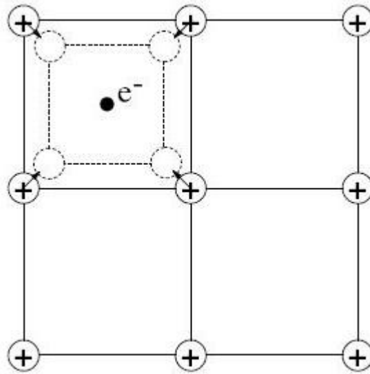
FIG. 2.1: Polaron diélectrique
