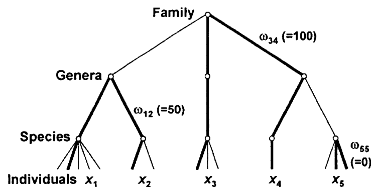
Figure 20 : Schéma théorique illustrant la notion de distance taxonomique ( w_{ij} ) entre les niveaux taxonomiques dans un arbre phylogénique (d'après Clarke et Warwick, 1994).
