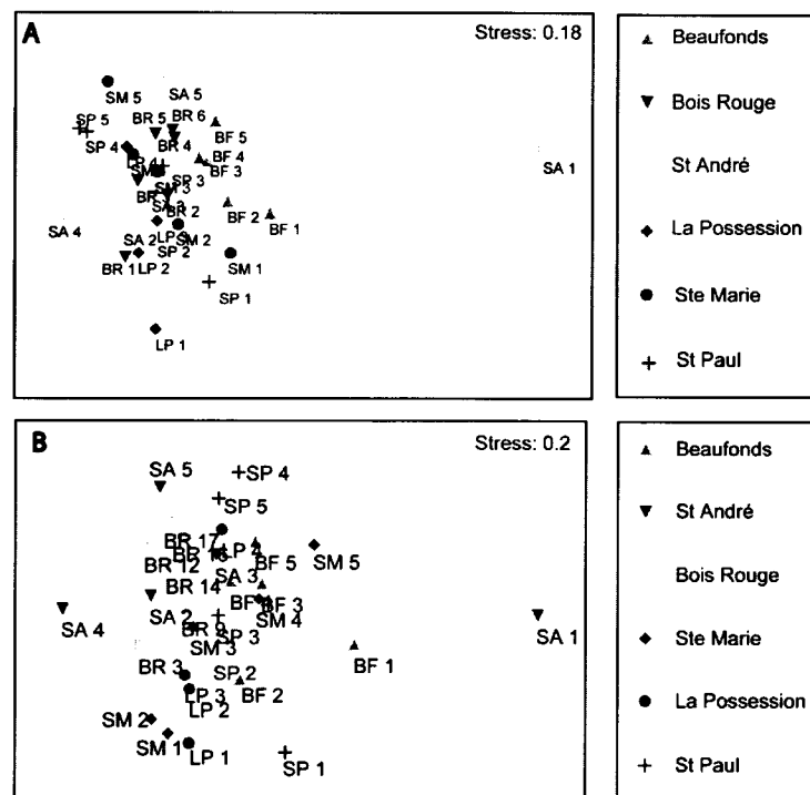
Figure 34: NMDS effectué sur les données d'abondance (A), et sur les données de biomasses (B) après transformation racine carrée.
