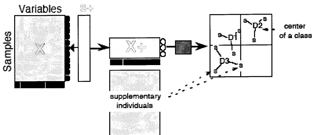
Figure 23: Schéma du principe de l'AFC interclasse. Le facteur discriminant noté S+ peut être l'effet « site » ou l'effet « profondeur ». X+ correspond à l'étape de regroupement des échantillons « synthétiques » vis-à-vis du facteur S+. Les échantillons supplémentaires correspondent eux à la matrice initiale. La projection finale sur les axes de l'AFC met en évidence les facteurs de discrimination (centre de gravité) et la manière dont se répartissent les échantillons (d'après Thioulouse, et al., 1996).
