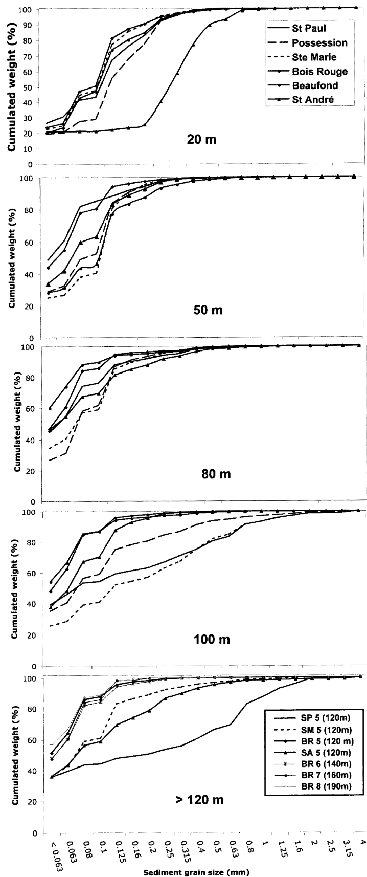
Figure 30 : Granulométrie des sédiments - courbes de fréquences cumulées par fractions granulométriques par profondeur et par sites échantillonnés.
