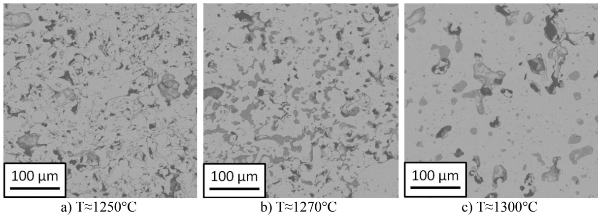
Figure 83 : Micrographies de trois zones d'acier X120Mn12 dont le frittage par induction est très hétérogène (densité moyenne de 82 %)
