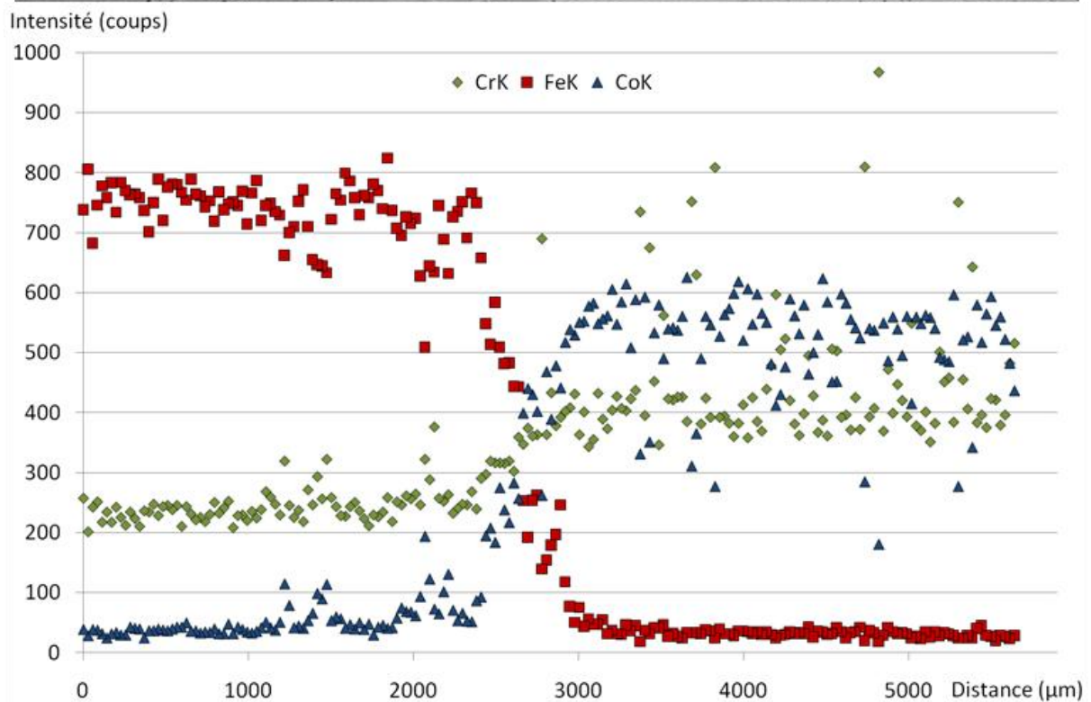
Figure 136 : Micrographie BSE et profil qualitatif de composition associé au niveau de l'interface du bimatériau bicouche Frittage réalisé avec un débit de 100 L/h de He+4 %vol. H 2 (1300°C, 1h)
