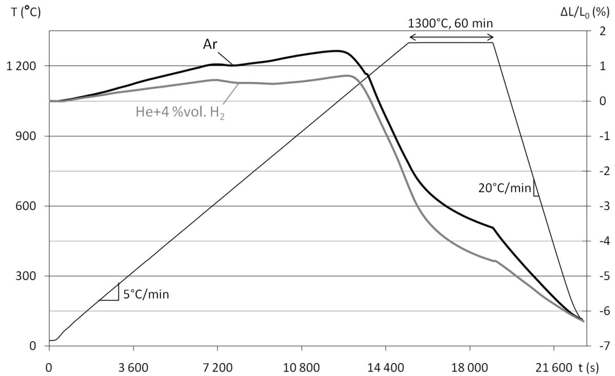
Figure 80 : Comparaison des courbes de retrait ( \Delta L/L_0 ) pour le monomatériau (acier X120Mn12 sans carbone+graphite) préalablement délianté suivant deux atmosphères, Ar et He+4 %vol. H_2 Frittage réalisé à 5°C/min jusqu'à 1300°C
