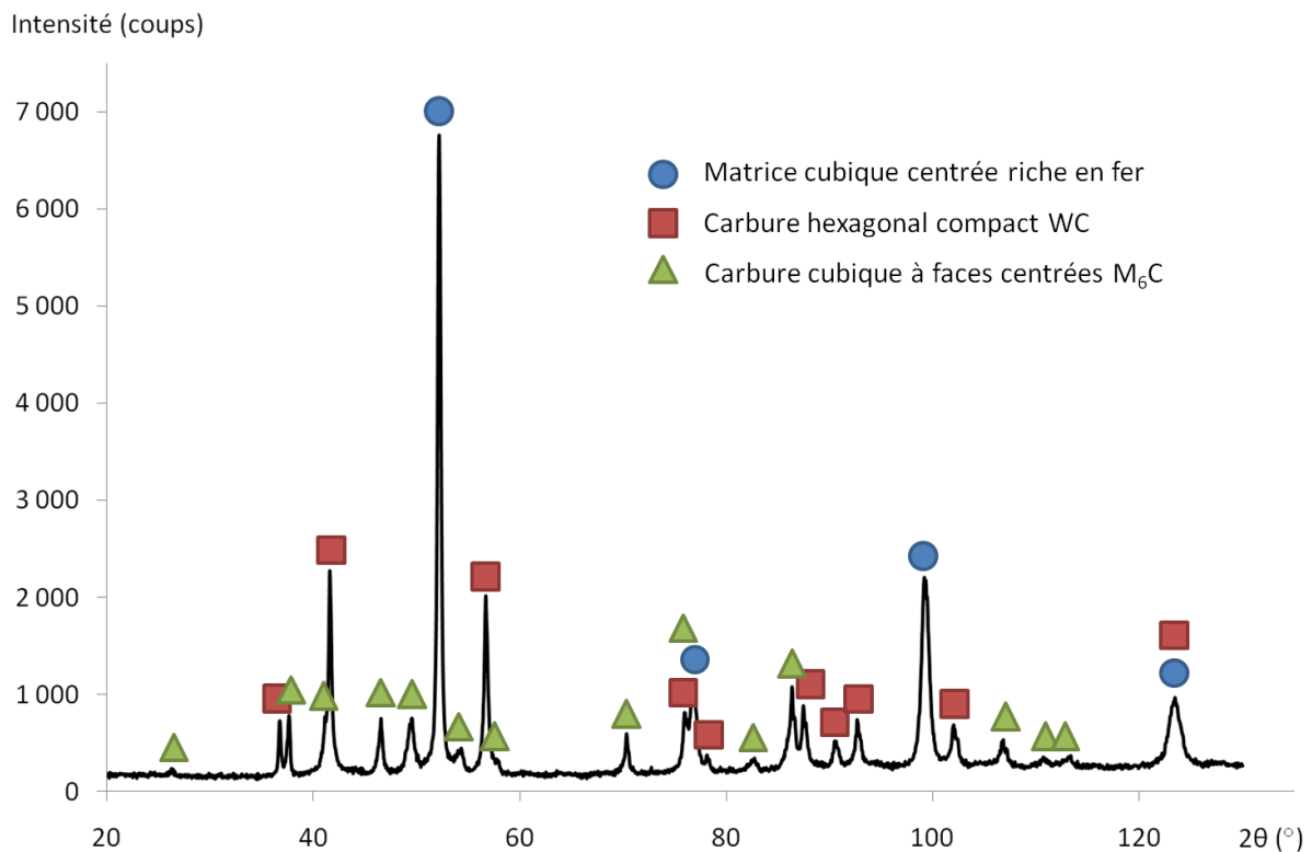
Figure 33 : Diffractogramme d'un échantillon du bimatériau fritté à 1300°C pendant une heure présentant la nouvelle phase formée à l'interface
