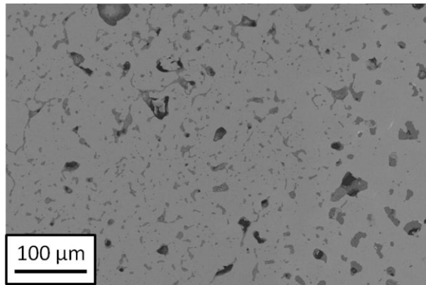
Figure 85 : Micrographie de l'acier X120Mn12 fritté dans un résistor en graphite T = 1290°C, t = 1h (densité non déterminée)
