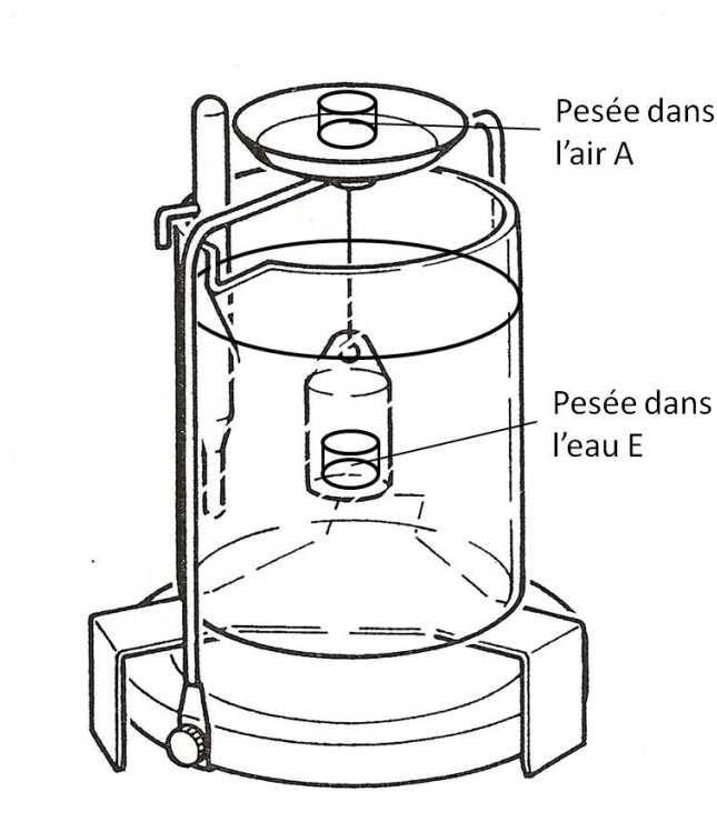
Figure 147 : Dispositif de pesée pour la détermination de la masse volumique d'un échantillon par le principe d'Archimède
