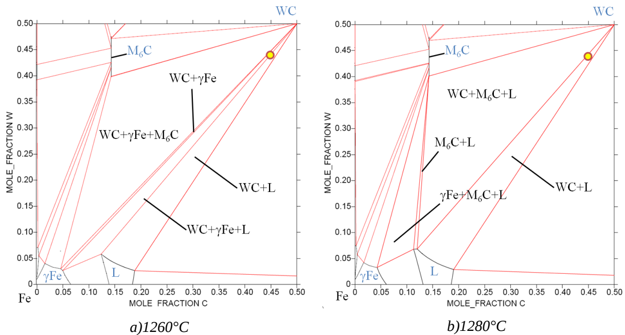
Figure 19 : Sections isothermes de la zone riche en fer du système ternaire C-Fe-W calculée à a) 1260 et b) 1280°C par le logiciel Thermo-Calc
