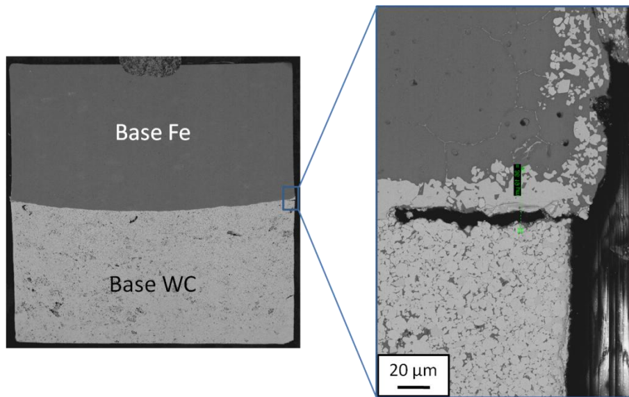
Figure 56 : Aspect microscopique d'un échantillon ayant formé de la phase \text{M}_6\text{C} sur la surface extérieure mais dont e=0\text{ }\mu\text{m} – C=0,62\text{ }\% m. – P=600\text{ MPa} – r=5^{\circ}\text{C}/\text{min} – T=1280^{\circ}\text{C} – t=60\text{ min}
