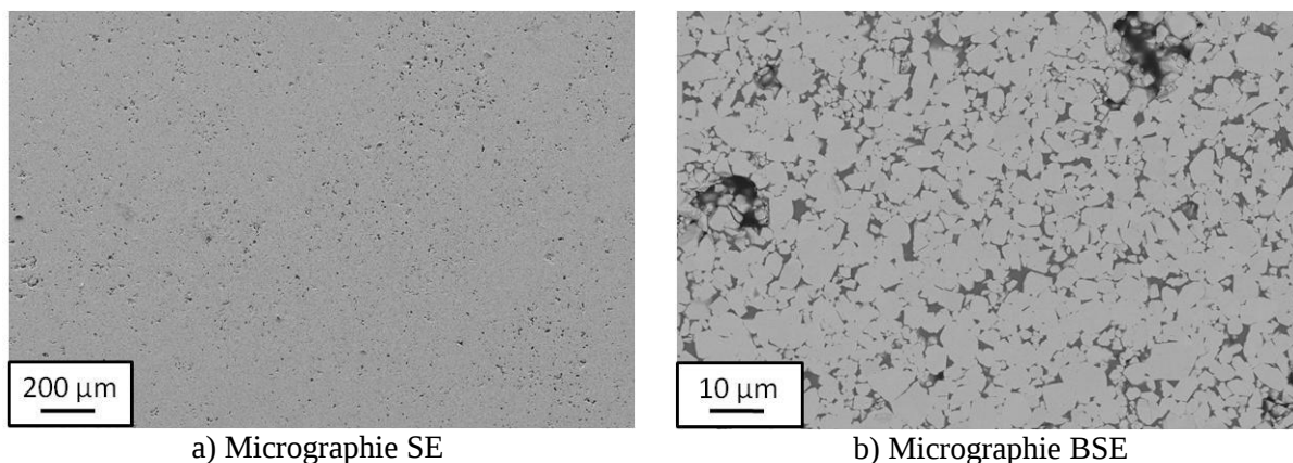
Figure 20 : Micrographies du monomatériau base WC après un frittage à 1300°C pendant 60 min Noir : pore / Gris foncé : liant riche en fer / Gris clair : carbure de tungstène
