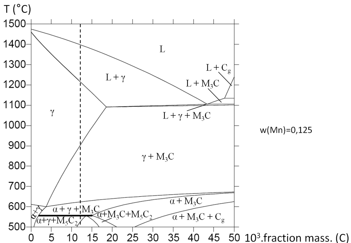
Figure 70 : Section isoplèthe du système C-Fe-Mn à 12,5 % Mn en fonction de la teneur en carbone calculée à partir de Thermo-Calc – La verticale en pointillés correspond à une teneur en carbone de 1,2 %m. (composition du X120Mn12)
