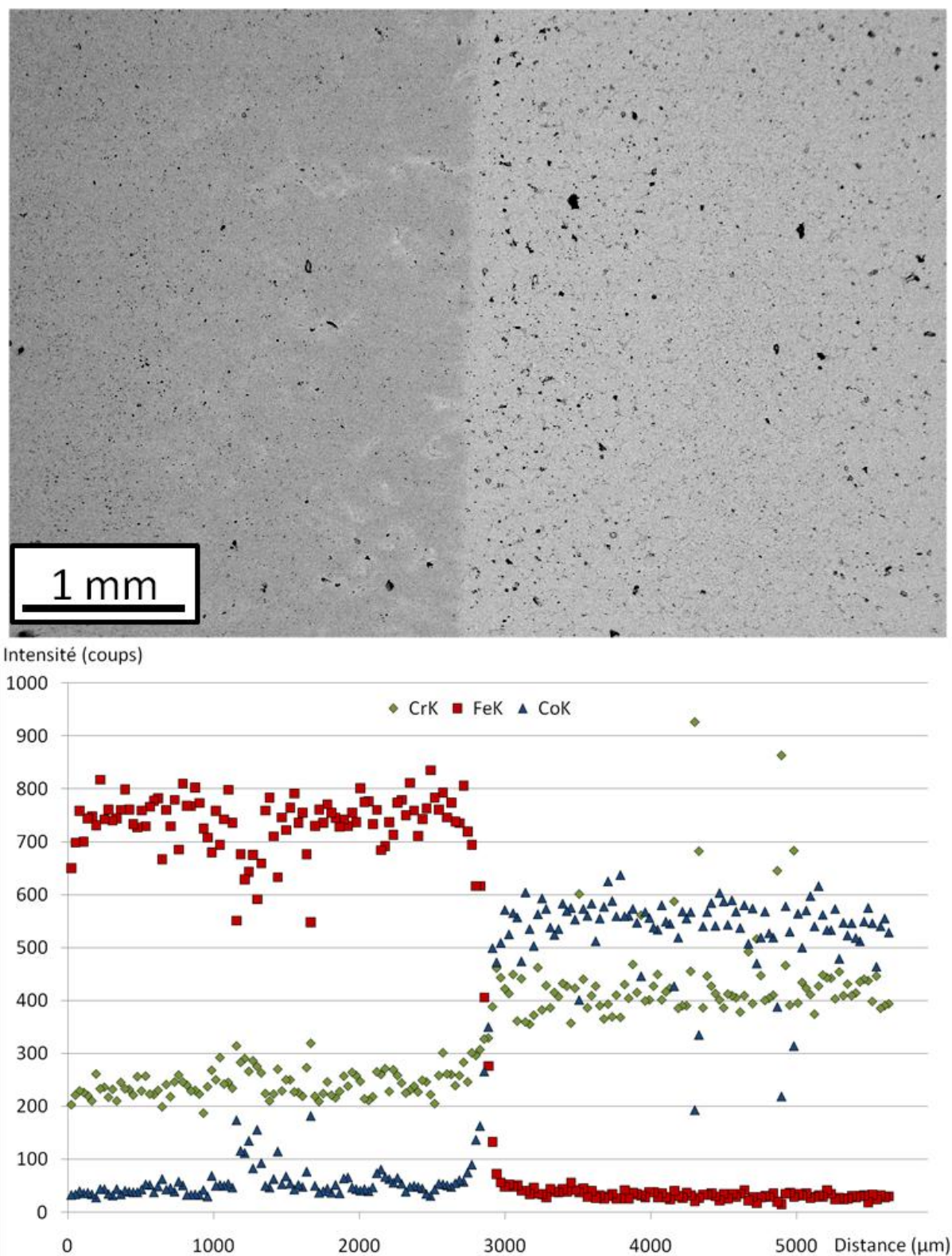
Figure 135 : Micrographie BSE et profil qualitatif de composition associé au niveau de l'interface du bimatériau bicouche Frittage réalisé avec un débit de 20 L/h de He+4 %vol. H 2 (1300°C, 1h)
