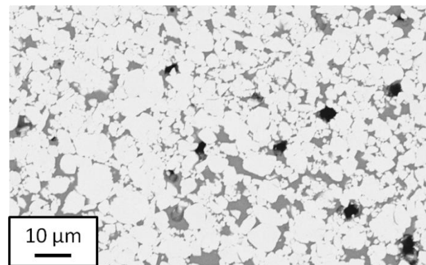
Figure 87 : Micrographie de l'échantillon base WC fritté dans un résistor en graphite T = 1280°C, t = 10 min (densité non déterminée)
