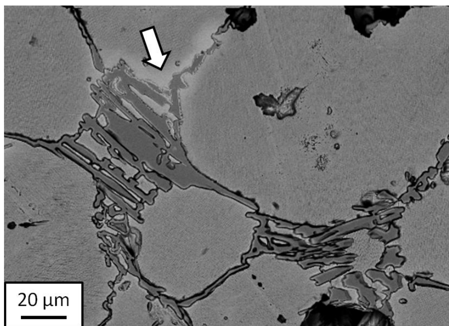
Figure 127 : Micrographie BSE du cœur de l'échantillon Stellite 6 fritté 60 min à 1305°C La flèche indique la présence d'une zone plus riche en tungstène (plus claire)
