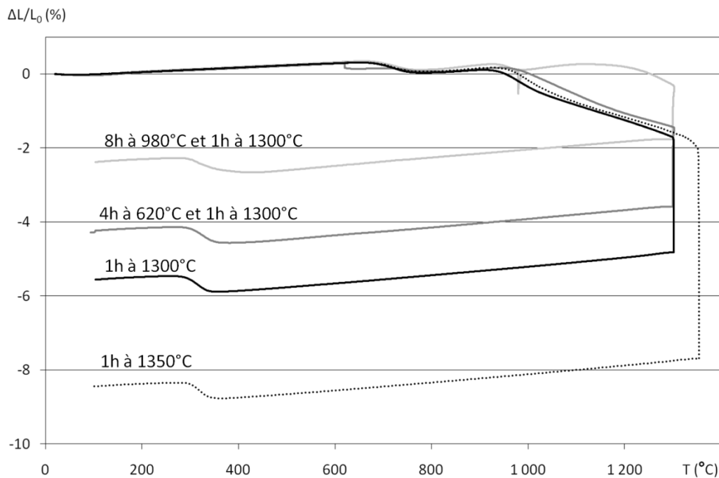
Figure 116 : Comparaison des courbes de retrait ( \Delta L/L_0 ) pour le monomatériau acier 1.4313 suivant différents cycles thermiques en fonction de la température Frittage réalisé sous He+4 %vol. H 2 à 10°C/min
