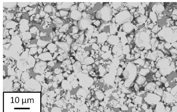
Figure 86 : Micrographie de l'échantillon base WC fritté par SPS T = 1150°C, t = 3 min 40 (densité non déterminée)
