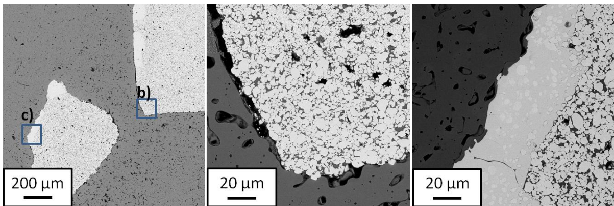
a) Vue générale et repérage des zones b et c b) Absence de contact matrice/insert c) Contact matrice/insert : Formation de M_6C
