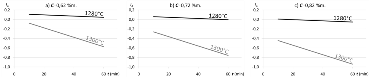
Figure 50 : Evolution de l'indice d'anisotropie de retrait I_A en fonction de la composition en carbone C , de la température T et du temps de frittage t – P=500\text{ MPa} – r=4^\circ\text{C/min}
