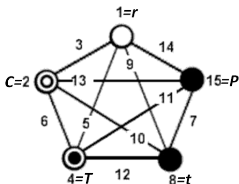
Figure 35 : Matrice de Taguchi L16 et diagramme utilisés pour la détermination de l'ordre des essais (les cinq paramètres étudiés sont représentés par les cercles) [TAG'93] - : niveau inférieur ; + : niveau supérieur
