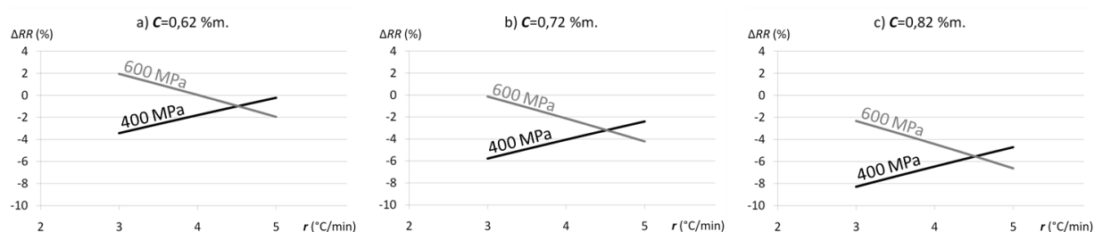
Figure 49 : Evolution de la différence de diamètres finaux \Delta\varnothing_f en fonction de la composition en carbone C , de la pression de compaction P , et de la vitesse de chauffe r – T=1290^\circ\text{C} - t=35 min
