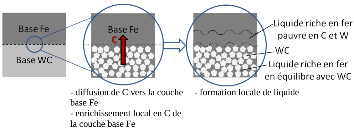
Figure 62 : Représentation schématique des prémices à la formation de la phase \text{M}_6\text{C}
