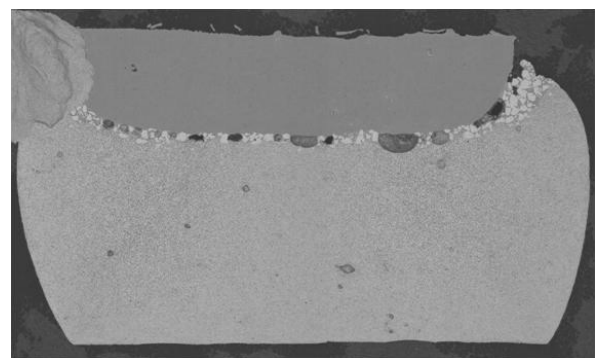
b) Type III ( C=0,82\text{ \%m.} - P=600\text{ MPa} - r=5^\circ\text{C/min.} - T=1300^\circ\text{C} - t=60\text{ min} )
