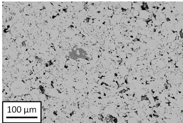
Figure 84 : Micrographie de l'acier X120Mn12 fritté par SPS T ≈ 1220°C, t = 1 min 20 (d = 85 %)
