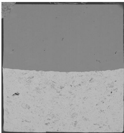
a) Type I ( C=0,82\text{ \%m.} - P=400\text{ MPa} - r=5^\circ\text{C/min.} - T=1280^\circ\text{C} - t=60\text{ min} )
