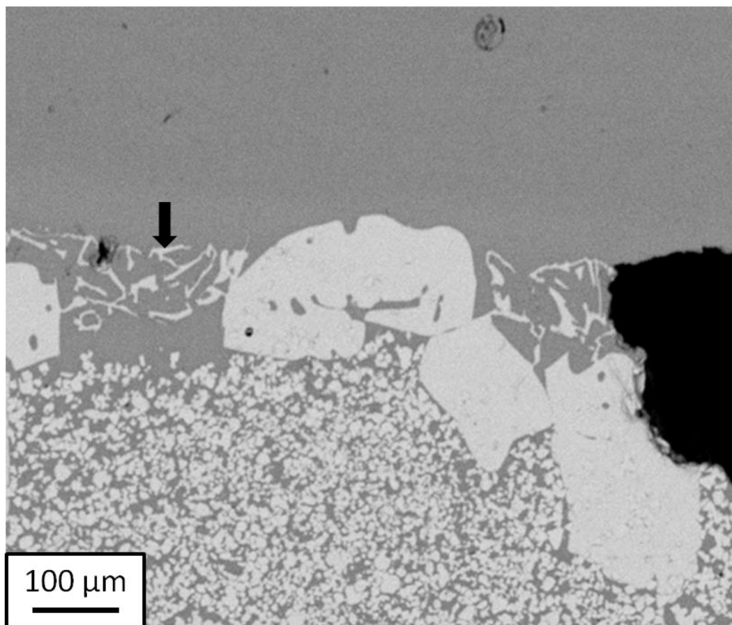
Figure 67 : Micrographie BSE au niveau de l'interface d'un échantillon de type III C=0,82\text{ \%m.} - P=400\text{ MPa} - r=3^{\circ}\text{C/min} - T=1300^{\circ}\text{C} - t=60\text{ min} La flèche indique la présence de M_6C en arête de poisson
