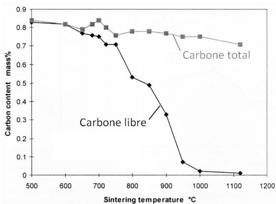
Figure 23 : Evolution de la teneur en carbone libre et de la teneur totale en carbone dans un mélange Fe-0,8 %m. C fritté 60 min sous \text{N}_2 en fonction de la température de frittage ( D_{50}(\text{Fe}) \approx 100 \mu\text{m} ) [DAN'01]
