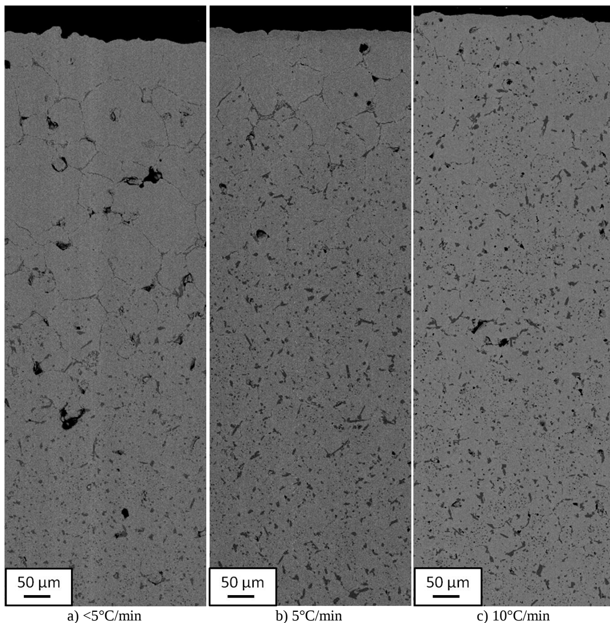
Figure 131 : Micrographies BSE de la surface du Stellite 6 pour les vitesses de chauffe
