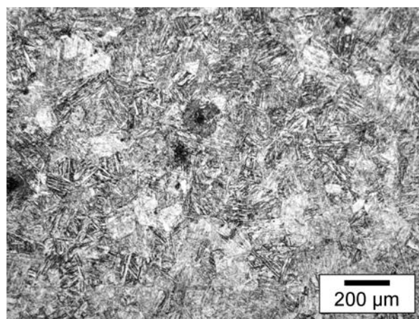
Figure 94 : Image au microscope optique de l'acier 1.4313 révéle à l'eau régale diluée montrant la structure martensitique
