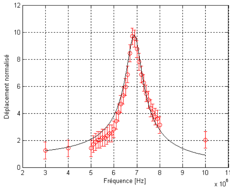
Figure 4.3-7 – Déplacement normalisé d'une poutre de dimension 5 \mu\text{m} \times 1 \mu\text{m} \times 50 \text{nm} en fonction de la fréquence d'excitation ( V_{\text{actionnement}} = 5 \text{mV} ).
