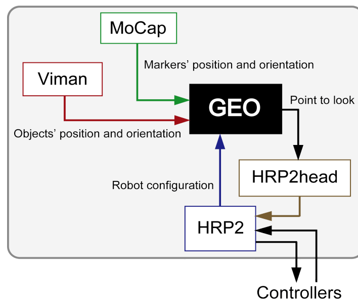
Figure 7.5: L'achitecture du système GEO, lequel reçoit l'information sur la capture du mouvement de l'homme ainsi que sur la position des objets dans l'environnement en utilisant les caméras embarquées .
