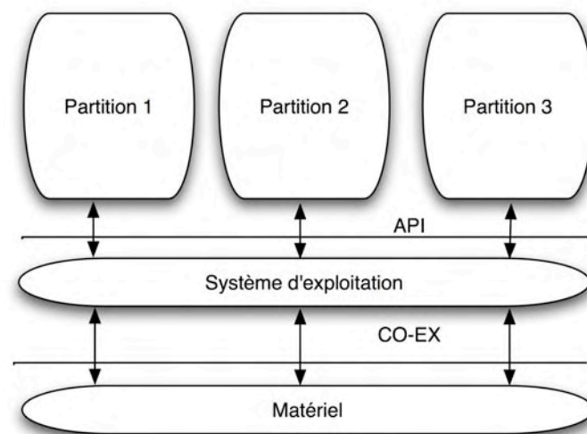
Figure II.3. Module IMA selon l'ARINC 653
