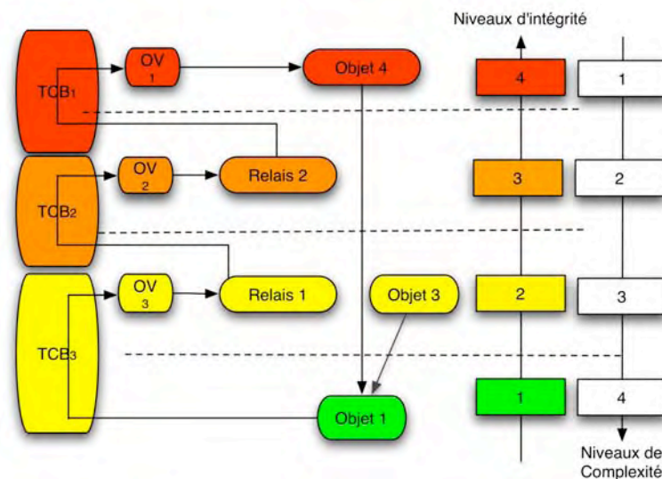
Figure V.10 Décomposition de la TCB
