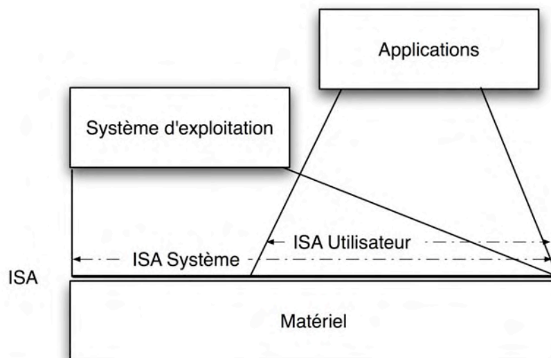
Figure IV.5 Architecture de jeu d'instructions (ISA)
