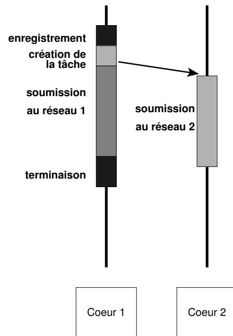
FIGURE 5.10 – Envoi d’un message sur deux réseaux simultanément en utilisant deux cœurs.
