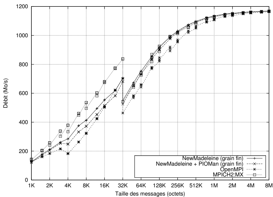
FIGURE 7.8 – Impact de PIOMAN sur le débit du réseau MYRINET
