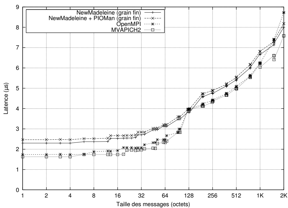
FIGURE 7.5 – Impact de PIOMAN sur la latence du réseau INFINIBAND
