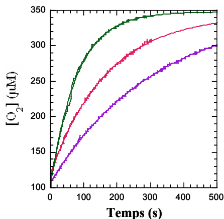
Figure 108 : Formation d'O 2 au cours de la réaction de la SOR sauvage (30 µM en violet et 50 µM en rose) et de son mutant E47A (80 µM en vert) avec H 2 O 2 (500 µM) dans 10 mM Tris/HCl pH 8.5 mesuré par électrode de Clark.
