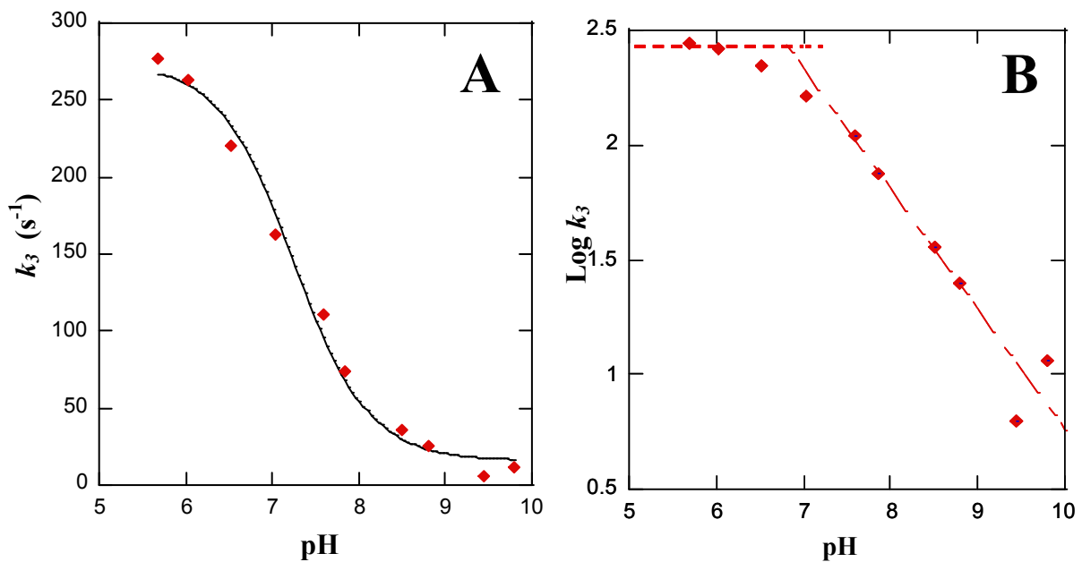
Figure 75 : Effet du pH sur k_3 , de la réaction de la SOR sauvage de D. baarsii (100 \mu\text{M} ) avec 8 \mu\text{M} ou 12 \mu\text{M} de \text{O}_2^- dans 10 mM formiate et 2 mM tampon. (A) Modélisation avec une sigmoïde, définissant un pKa : k_3 = (A_2 + A_1 \times 10^{(\text{pH} - \text{pKa})}) / (1 + 10^{(\text{pH} - \text{pKa})}) avec \text{pKa} = 7.2 \pm 0.1 . (B) A \text{pH} > 7 , \log k_3 est modélisable par l'équation \log k_3 = 6.97 - 0.64 \times \text{pH} . La cassure de pente est observée à \text{pH} 6.8 .
