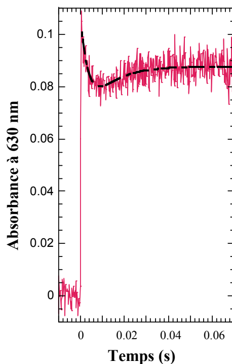
Figure 114 : Variation d'absorbance à 630 nm de la réaction de la SOR C13S (100 \mu\text{M} ) avec 20 \mu\text{M} de \text{O}_2^{\cdot -} générés par radiolyse pulsée dans 10 mM formiate et 2 mM Tris/HCl à pH 7.6. L'absorbance est mesurée dans une cuve de 2 cm de trajet optique.
