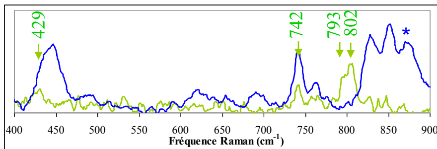
Figure 97 : Spectres de résonance Raman du site actif du mutant SOR K48I de D. baarsii réduit (4 mM) après réaction de sa forme réduite avec 30 équivalents de \text{H}_2^{16}\text{O}_2 (bleu), ou 6 équivalents de \text{H}_2^{18}\text{O}_2 (vert). La protéine est dans un tampon 50 mM Tris/HCl pH 8.5. Conditions d'enregistrement : Longueur d'onde d'excitation laser : 633 nm. Température : 100 K. Volume de l'échantillon 1 \mu\text{L} . Accumulation : 2 \times 10 s.
