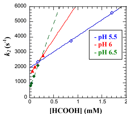
Figure 122 : Effet de la concentration de l'acide formique observé sur la constante de vitesse k_2 pour la réaction de la SOR de D. baarsii avec 9 ou 12 \mu\text{M} de \text{O}_2^- dans 2 mM de tampon à différent pH. pH 5.5 (bleu), pH 6 (rouge), pH 6.5 (vert).
