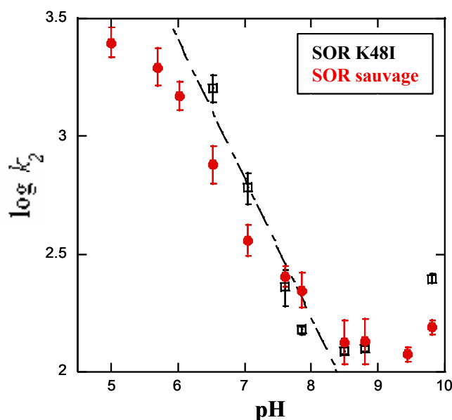
Figure 91 : Effet du pH sur la constante de vitesse k_2 , déterminée par radiolyse pulsée, pour la réaction de la SOR sauvage et le mutant K48I de D. baarsii (100 \mu M), avec 8 \mu M ou 12 \mu M de O_2^{\cdot-} dans 10 mM formiate et 2 mM tampon. Cette dépendance est modélisable entre pH 6 et pH 8.5 par l'équation : \log k_2 = \log(k_0) - 0.59 \times \text{pH} avec k_0 = 7.9 \times 10^6 \text{ M}^{-1} \cdot \text{s}^{-1} pour le mutant K48I et \log k_2 = \log(k_0) - 0.61 \times \text{pH} avec k_0 = 6.8 \times 10^6 \text{ M}^{-1} \cdot \text{s}^{-1} pour la SOR sauvage. k_0 représentant la valeur de k_2 lorsque le pH approche zéro.
