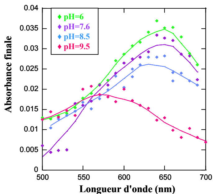
Figure 73 : Spectres de la SOR finale, 25 ms à 1 s après la réaction de la SOR WT de D. baarsii (100 \mu M) avec 8 \mu M de O_2^{\cdot -} dans 10 mM de formiate, 2 mM de tampon à pH 6, pH 7.6, pH 8.5 et pH 9.5. L'absorbance est mesurée dans une cuve de 2 cm de trajet optique.
