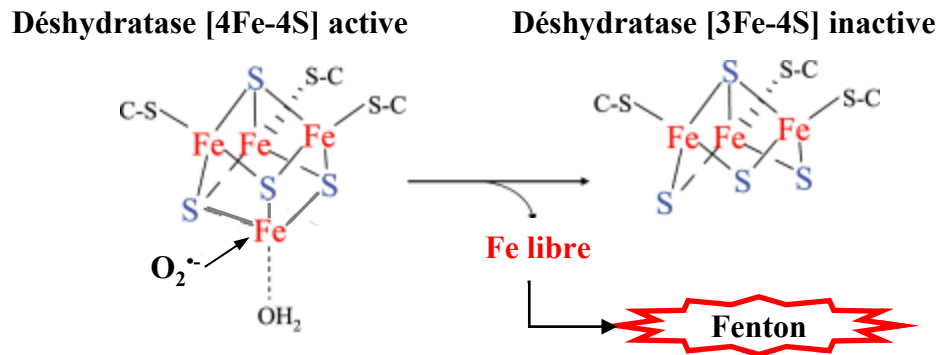
Figure 3 : Destruction du cluster [4Fe-4S] de déshydratase par O_2^{\bullet -} .
