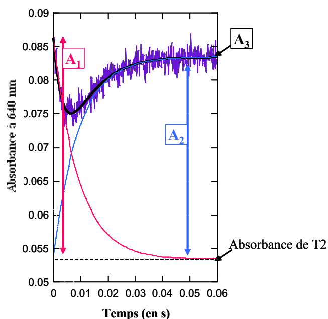
Figure 57 : Cinétique enregistrée à 640 nm ( violet ) durant la réaction de la SOR de D. baarsii (100 \mu M) dans 10 mM formiate, 2 mM Tris/HCl à pH 7.6 avec O_2^{\bullet-} (20 \mu M) généré par radiolyse pulsée, en présence de la lampe xénon et d'un filtre coupant en dessous de 345 nm. La courbe noire est la modélisation de la cinétique par un processus bi-exponentiel A = A_1 \exp(-255 \times t) - A_2 \exp(-110 \times t) + A_3 avec, A_1 = 0.0333 , A_2 = 0.0301 et A_3 = 0.0835 . Les courbes rose et bleue représentent chacune l'une des deux phases du modèle bi-exponentiel, correspondant soit à la formation du T_2 ( rose ) A = A_1 \exp(-255 \times t) - A_2 + A_3 soit à celle de du T_3 ( bleu ) A = A_3 - A_2 \exp(-110 \times t) .
