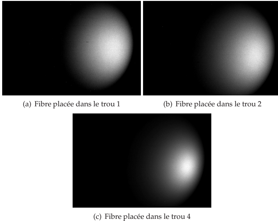
FIGURE IX.5 – Images 1500 \times 1020 pixels acquises par la caméra. Les échelles de couleurs sont adaptées dynamiquement en fonction du niveau de signal.
