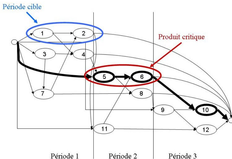
FIG. 3.5 – Représentation de la période cible
