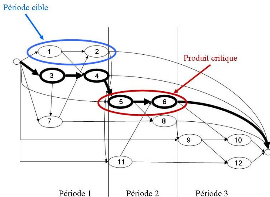
FIG. 3.3 – Représentation du chemin violé, du produit critique pour le période 2 et de la période cible
