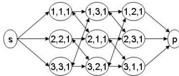
FIG. 2.1 – Graphe disjonctif avec 3 produits et 3 machines
