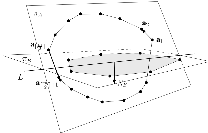
FIG. 2.16 – Principe de la recherche dichotomique. Cas où \mathbf{v} < 0 et \mathbf{v}' > 0 , la sous-chaîne \mathbf{a}_1, \mathbf{a}_2, \dots, \mathbf{a}_{\lceil m/2 \rceil} peut être supprimée.
