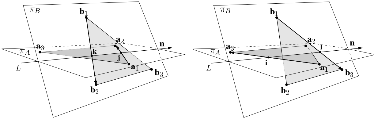
FIG. 2.7 – Une fois les sommets de chaque triangle permutés dans une forme canonique, les triangles s'intersectent si et seulement si [\mathbf{a}_1, \mathbf{a}_2, \mathbf{b}_1, \mathbf{b}_2] \leq 0 et [\mathbf{a}_1, \mathbf{a}_3, \mathbf{b}_3, \mathbf{b}_1] \leq 0 .
