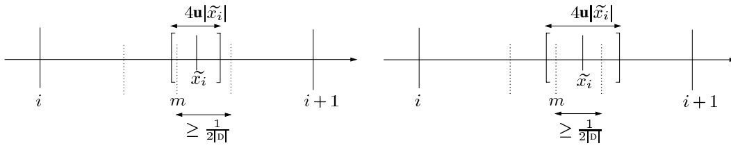
FIG. 3.3 – À gauche, \frac{1}{2|D|} > 4u|\tilde{x}_i| et m est la seule valeur possible de la construction, à droite \frac{1}{2|D|} < 4u|\tilde{x}_i| et le résultat de la construction reste ambiguë.
