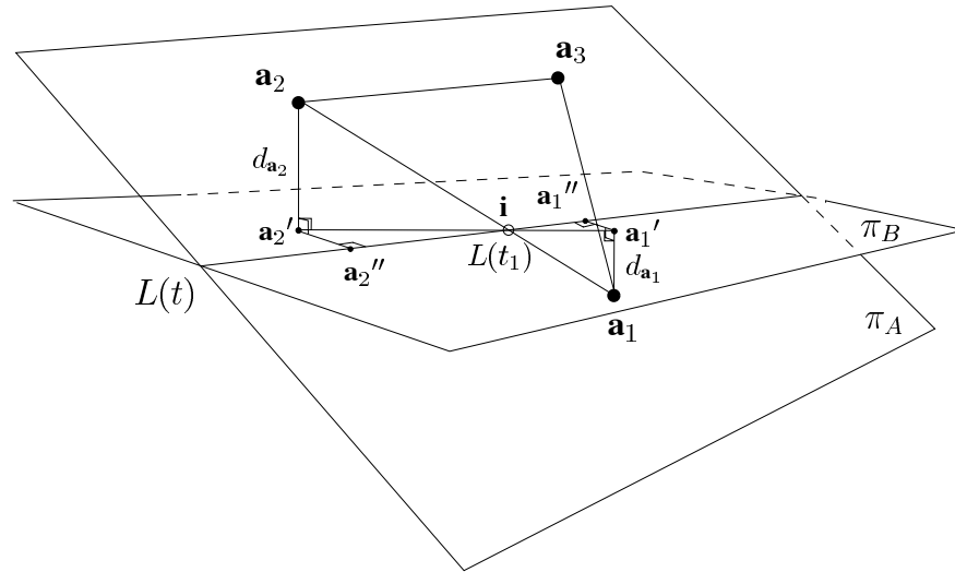
FIG. 2.5 – Les triangles \Delta \mathbf{a}_1 \mathbf{i} \mathbf{a}_1' et \Delta \mathbf{a}_2 \mathbf{i} \mathbf{a}_2' sont similaires.
