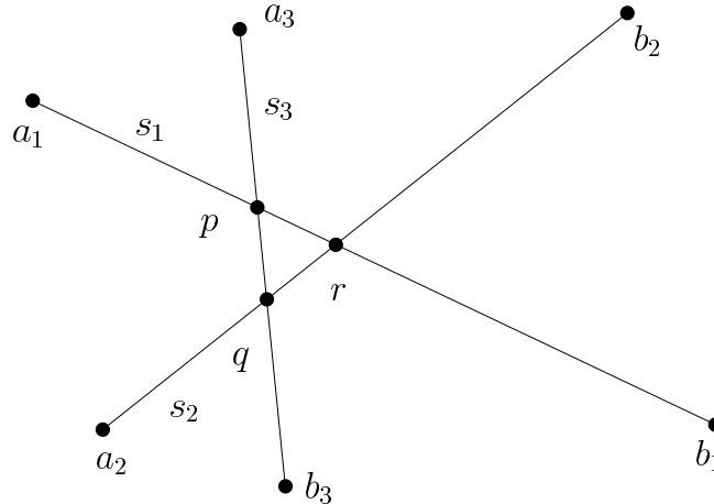
FIG. 1.5 – Incohérences potentielles de l'algorithme de balayage.
