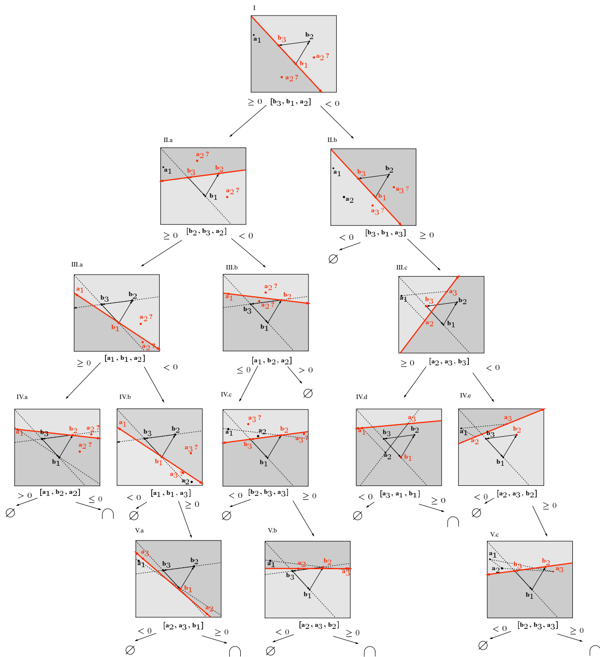
FIG. 2.13 – Arbre de décision correspondant au cas où \mathbf{a}_1 appartient à la région R_2 .
