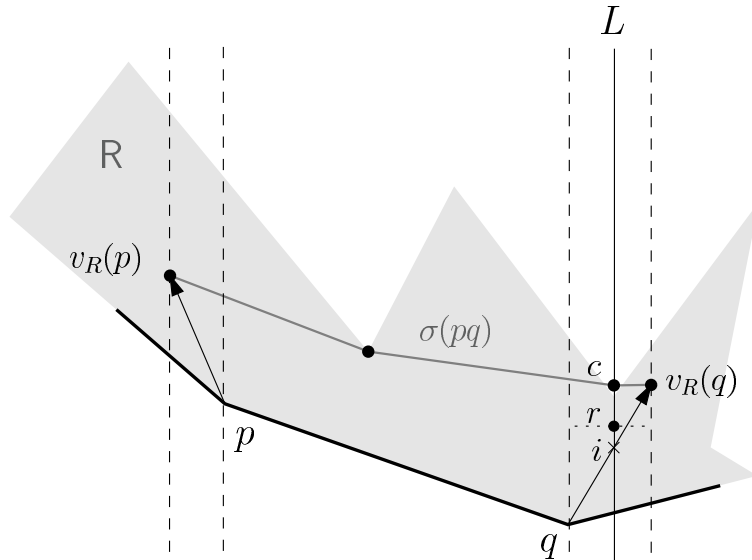
FIG. 4.8 – Si c est un sommet de \sigma(pq) entre v_R(p) et v_R(q) alors c est verticalement visible depuis pq dans R .
