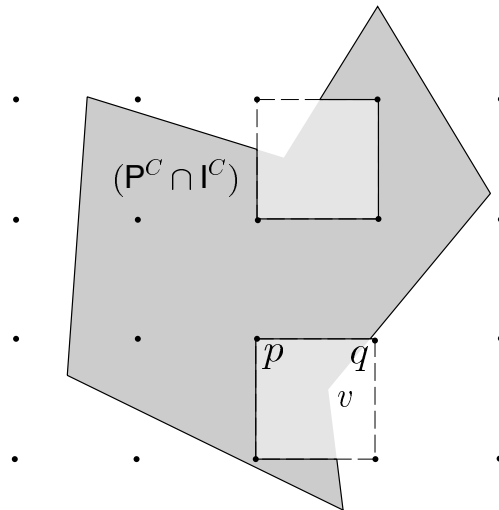
FIG. 4.13 – Si l'arête pq est issue d'une arête de I et au moins une de ses extrémités est un point de la grille alors \sigma(pq) \subseteq pq et \sigma(pq) est à une distance inférieure à \sqrt{2} du sommet v de R .
