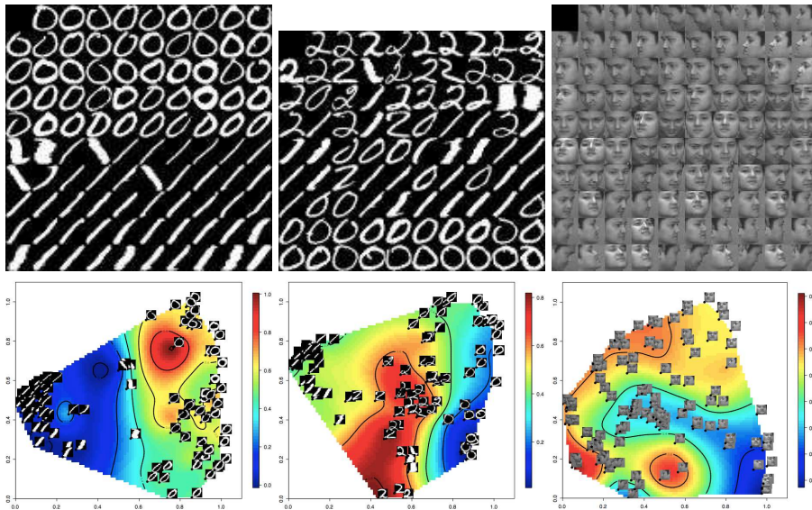
FIG. 5.4: Calcul de distance avec l'équation eikonale sur des bases de données d'images — application à l'ordonnancement de variétés d'images. Comparaison avec les résultats obtenus avec l'algorithme des k plus proches voisins utilisant la distance Euclidienne. Chaque résultat présenté est ordonné du plus proche (en haut à gauche) au plus éloigné (en bas à droite) en terme de distance et en accord avec les marqueurs présentés à la figure 5.3. Dans la première partie : les résultats obtenus avec l'algorithme des k plus proches voisins. Dans la seconde partie : les résultats obtenus avec notre approche ( la première ligne ) et les cartes de distances obtenues avec l'équation eikonale ( la seconde ligne ).
