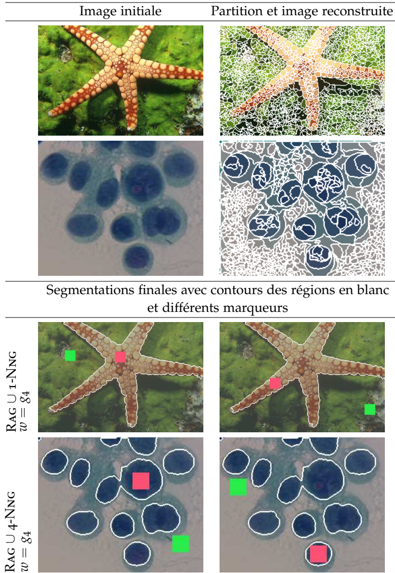
FIG. 5.8: Segmentation non locale d'image avec graphes basés régions. Dans la première partie, pour chaque ligne et de gauche à droite : l'image initiale et l'image reconstruite avec la couleur moyenne. Les régions de la partition sont également superposées en blanc. La première image contient 154 401 pixels et la seconde 49 000 pixels. Les partitions contiennent respectivement 2 391 régions et 741 régions (98% de réduction pour les deux cas). Dans la seconde partie, pour chaque ligne et de gauche à droite : les segmentations obtenues où les contours des régions segmentées sont superposés en blanc sur l'image initiale. Les marqueurs originaux sont également représentés, de couleur rouge pour les objets à segmenter et de couleur verte pour l'arrière-plan.
