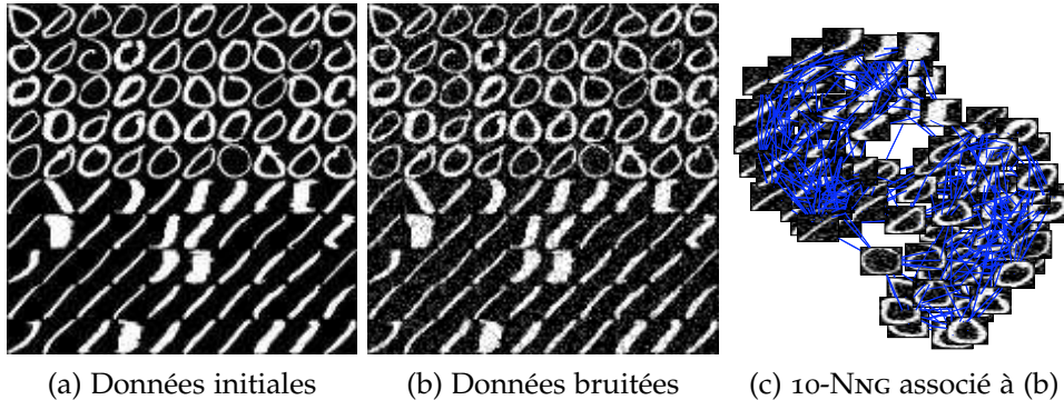
FIG. 3.1: Échantillon de tests pour le débruitage des données de la base USPS par filtrage isotrope (figure 3.2) et anisotrope (figure 3.9 page 67). (b) : données bruitées à partir de (a) par un bruit Gaussien de variance égale à 40. (c) : 10-NNG pondéré par la fonction g_3 , \text{card}(V) = 100 et chaque sommet est caractérisé par une fonction initiale f^0 : V \rightarrow \mathbb{R}^{16 \times 16} .
