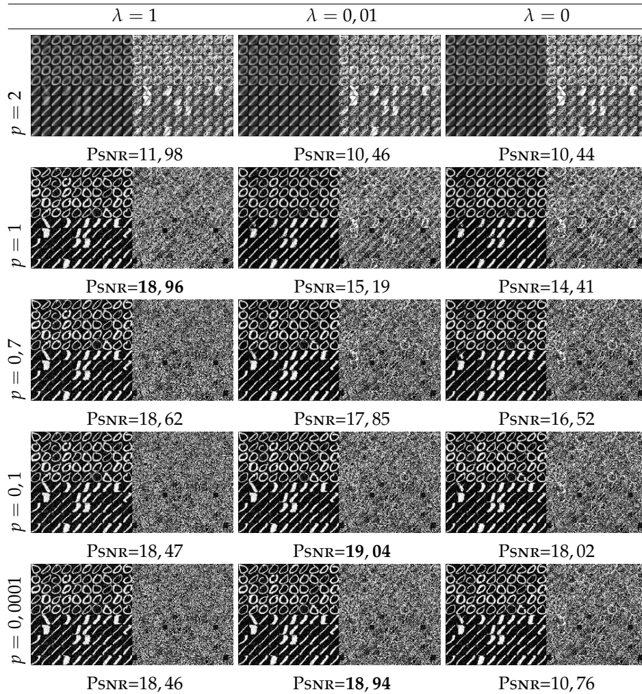
FIG. 3.9: Filtrage anisotrope d'une variété d'images (base Usps). Les données filtrées sont celles de la figure 3.1 page 57 avec différentes valeurs des paramètres p et \lambda . Chaque résultat présente le résultat du filtrage (la fonction finale f ), la différence avec les données initiales ( |f^0 - f| ) et une valeur de PSNR.
