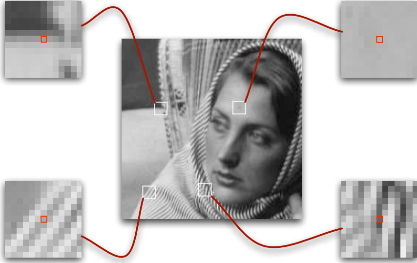
FIG. 2.4: Quatre exemples de patches comme vecteur d'attributs caractérisant les sommets du graphes. Ici, le pixel central (en rouge) est caractérisé par un vecteur de niveaux de gris défini grâce à un patch de taille 13 \times 13 .
