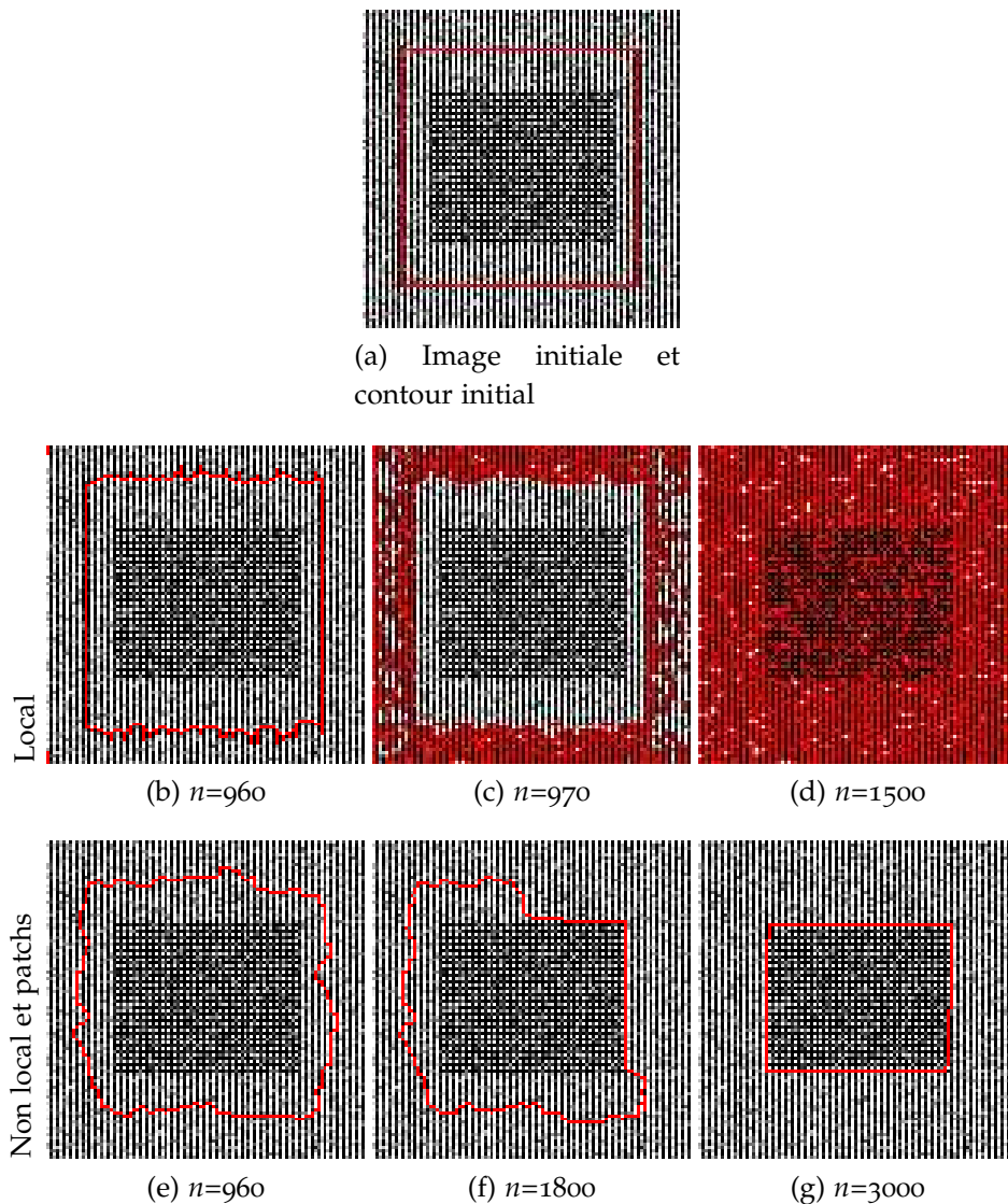
FIG. 3.33: Modèle de Cv discret défini sur des graphes appliqué à la segmentation non locale d'images. (a) : Image initiale et marqueur initial. À la première ligne : résultats avec une configuration locale. À la seconde ligne : résultats avec une configuration non locale et patches. De gauche à droite évolution de la segmentation en fonction du nombre n d'itérations.
