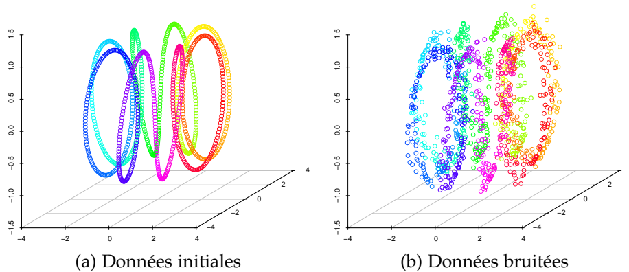
FIG. 3.3: Hélice toroïdale bruitée pour illustrer la simplification de variétés par filtrage isotrope (figures 3.4 et 3.5) et anisotrope (figures 3.10 page 68 et 3.11 page 69). (b) : données bruitées à partir de (a) avec un bruit Gaussien de variance égale à 10.
