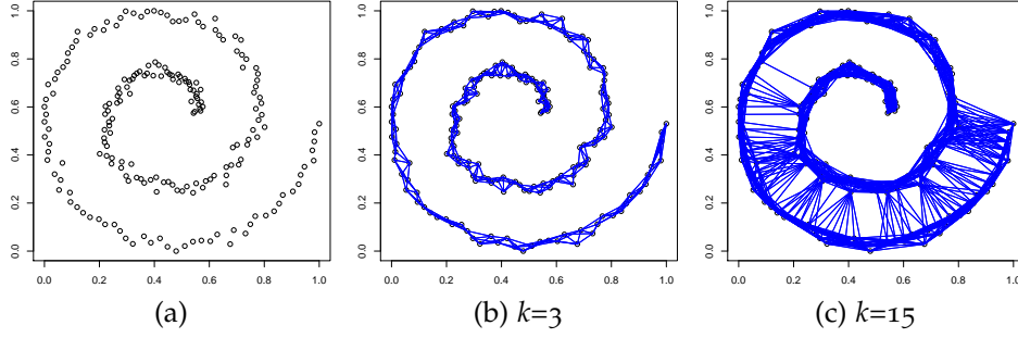
FIG. 2.1: Exemples de graphes des k plus proches voisins. (a) : données initiales dans \mathbb{R}^2 , (b) : 3-NNG, (c) : 15-NNG.
