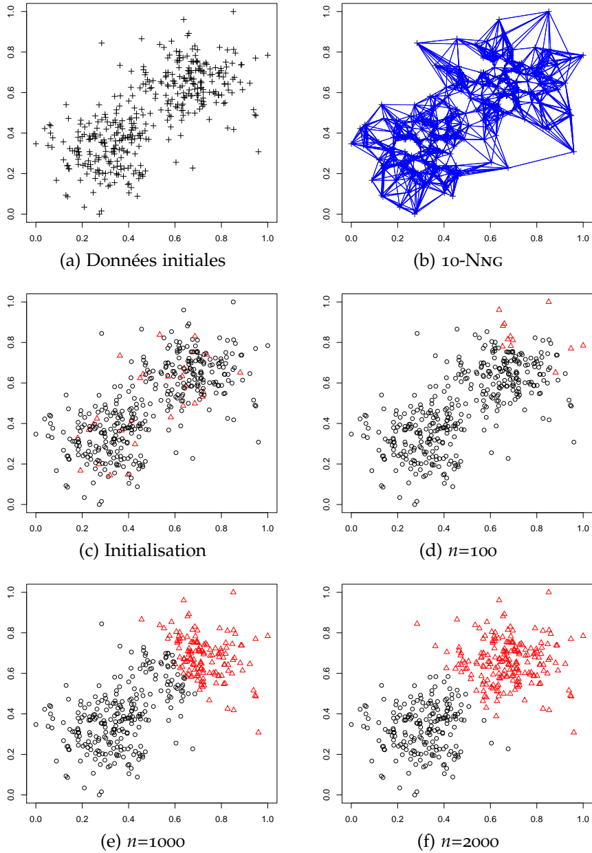
FIG. 3.34: Partitionnement de nuages de points (deux Gaussiennes) avec le modèle discret de C_v défini sur des graphes. (a) : les données initiales ( f^0 : V \rightarrow \mathbb{R}^2 ). (b) : 10-NNG associé aux données initiales. (c) : initialisation aléatoire des marqueurs. (d) et (e) évolution du partitionnement en fonction du nombre n d'itérations (f) : partitionnement final.
