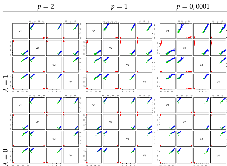
FIG. 3.7: Filtrage isotrope de la base de données « iris » avec différentes valeurs des paramètres p et \lambda . La première ligne montre les résultats pour \lambda = 1 et la seconde avec \lambda = 0 .
