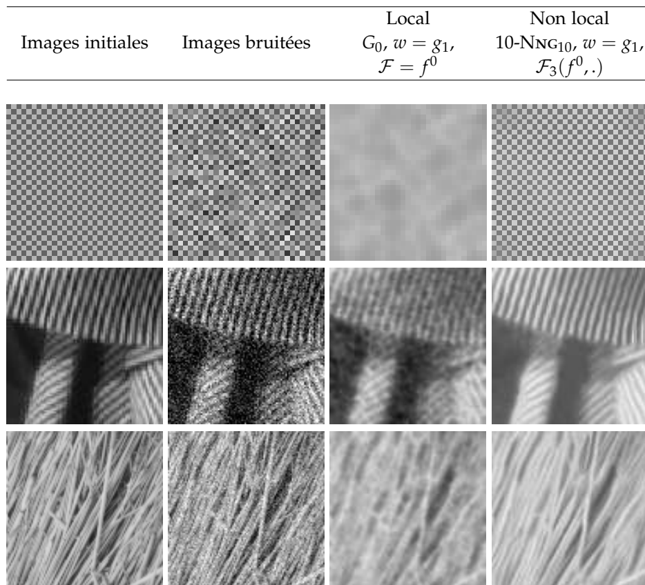
FIG. 4.4: Comparaison entre fermetures locales et non locales avec des patches. Images initiales (première colonne). Images bruitées (Gaussien de variance égale à 20) (deuxième colonne). Local (troisième colonne). Non Local avec des patches (dernière colonne).
