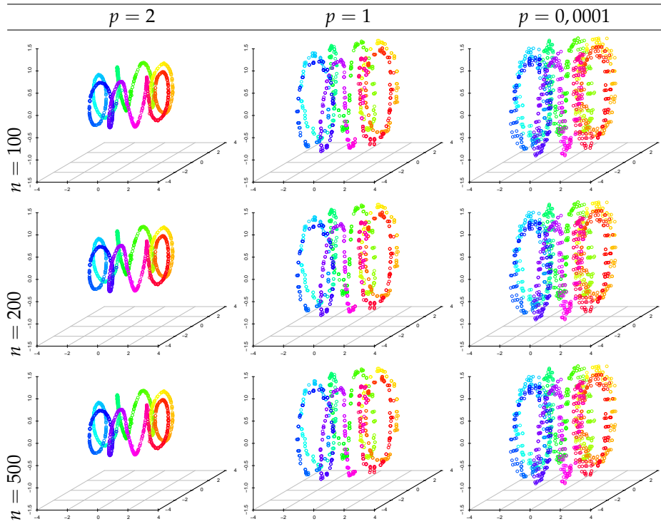
FIG. 3.10: Évolution (en fonction du nombre d'itérations n ) du filtrage anisotrope de la variété avec différentes valeurs des paramètres p et \lambda = 1 . Les données traitées correspondent à celles représentées par la figure 3.3 page 59.
