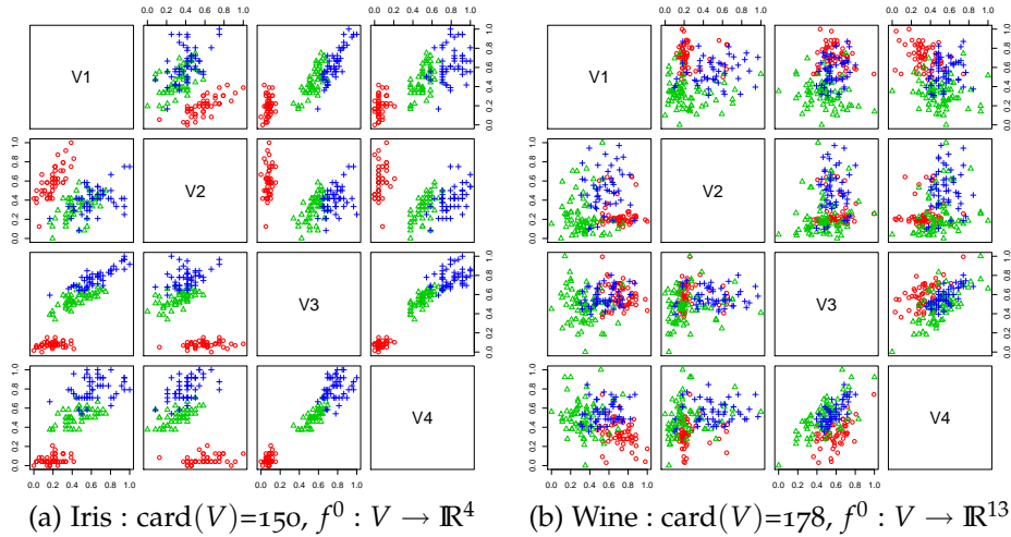
FIG. 3.6: Bases de données provenant du dépôt de l'UCI pour illustrer le filtrage et la simplification de données (isotrope : figures 3.7 et 3.8, anisotrope : figures 3.12 page 70 et 3.13 page 70) comme pré-traitement à une étape de regroupement ou de classification. Les figures représentent des projections par paires selon les attributs de chaque base. Pour la base « wine », la projection est faite sur les 4 premiers attributs des 13 contenus dans la base initiale.
