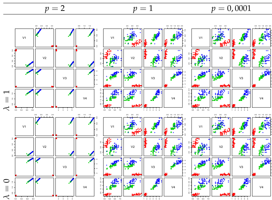
FIG. 3.12: Filtrage anisotrope de la base de données « iris » avec différentes valeurs des paramètres p et \lambda . La première ligne montre les résultats pour \lambda = 1 et la seconde pour \lambda = 0 .
