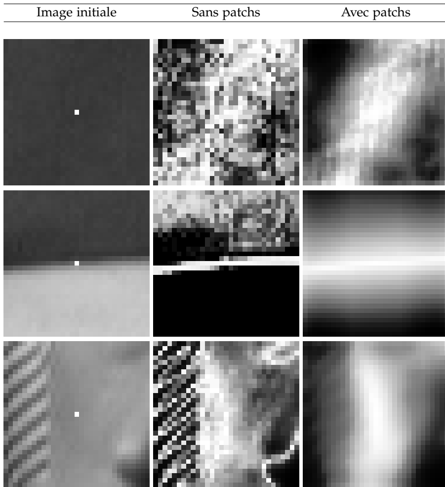
FIG. 2.5: Exemples de distribution des poids sur des images et influence de l'utilisation des patches comme vecteurs d'attributs. Les distributions sont estimées pour le pixel central (représenté par le pixel blanc) de l'image initiale. Le graphe considéré est un graphe reliant le pixel central à tous les autres pixels.
