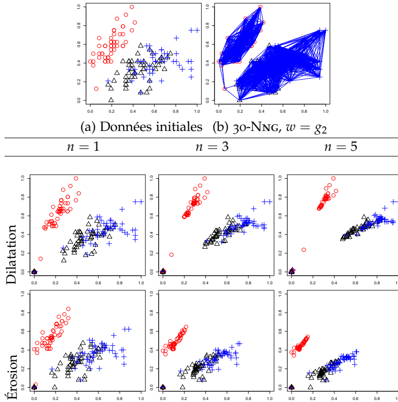
FIG. 4.7: Évolution des opérations de dilatation et d'érosion sur la base « iris ». La fonction f^0 associée aux données est définie (et traitée) comme une fonction f^0 : V \rightarrow \mathbb{R}^4 . Les résultats présentent uniquement une projection sur deux attributs. (a) : données initiales ; (b) : 30-NNG. La première ligne : évolution d'une dilatation ; la deuxième ligne : évolution d'une érosion.
