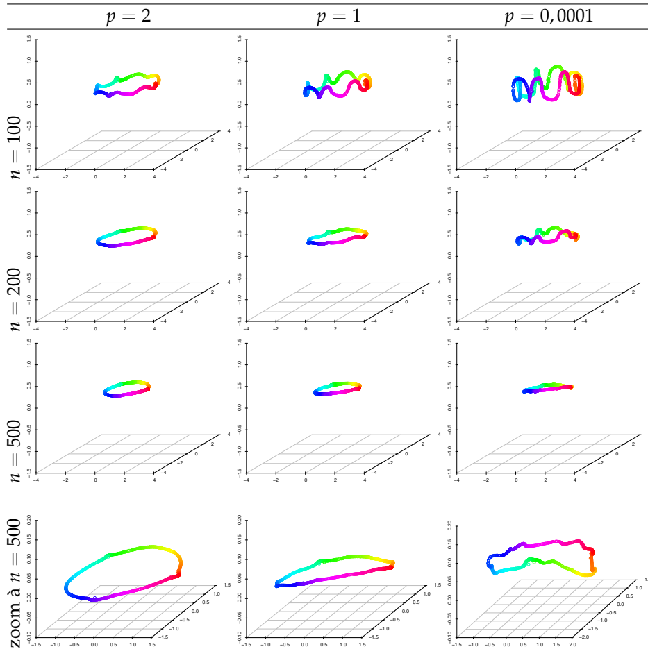
FIG. 3.5: Évolution (en fonction du nombre d'itérations n ) du filtrage isotrope d'une variété avec différentes valeurs des paramètres p et \lambda = 0 . Les données traitées correspondent à celles représentées par la figure 3.3. Les figures de la dernière ligne correspondent à un zoom pour l'itération n = 500 .
