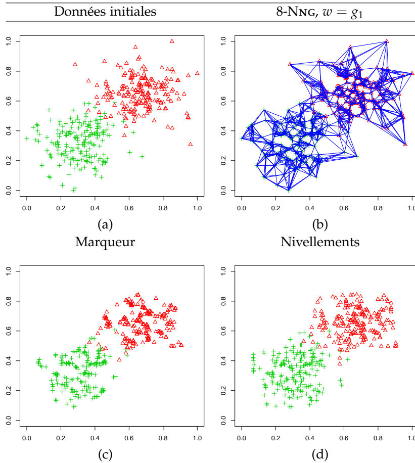
FIG. 4.9: Filtrage par nivellements de deux Gaussiennes. La fonction f^0 associée aux données est définie et traitée comme une fonction f^0 : V \rightarrow \mathbb{R}^2 . (a) : les données initiales. (b) : 8-NNG associée aux données. (c) : marqueur obtenu par régularisation discrète isotrope. (d) : résultat du filtrage par nivellements.
