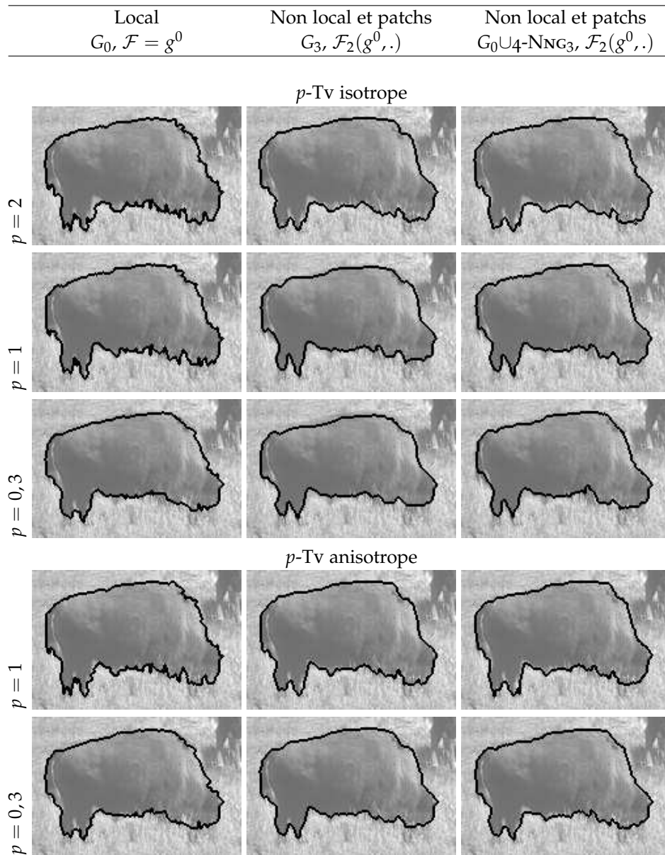
FIG. 3.18: Segmentation non locale d'images. Les graphes associés sont construits à partir de l'image initiale g^0 : V \rightarrow \mathbb{R} de la figure 3.17. Les segmentations sont obtenues avec les marqueurs initiaux présentés dans la figure 3.17. Chaque résultat correspond à une structure de graphe différente et à une valeur du paramètre p différent. Les contours des régions obtenus sont superposés en noir sur l'image initiale (volontairement blanchie afin d'avoir une meilleure visualisation).
