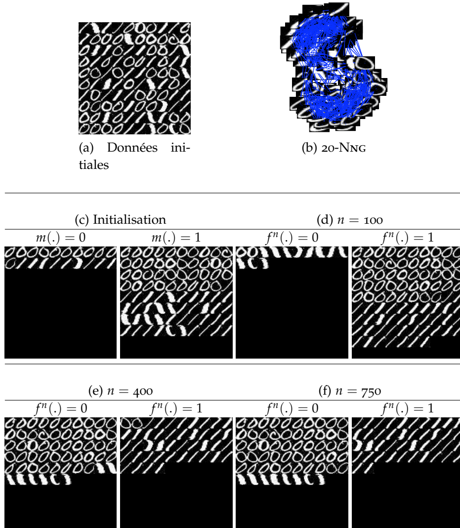
FIG. 3.35: Partitionnement de base de données (base de l'USPS) avec le modèle de Cv discret défini sur des graphes. (a) : données initiales ( f^0 : V \rightarrow \mathbb{R}^{256} ). (b) : 20-NNG associé aux données initiales. (c) : initialisation où m(\cdot) = 0 et m(\cdot) = 1 représentent les partitions initiales. (d) et (e) : évolution du partitionnement. en fonction du nombre n d'itérations. (f) : partitionnement final.
