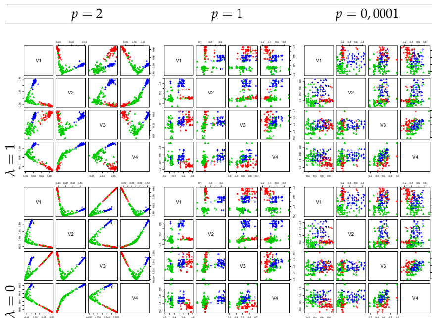
FIG. 3.13: Filtrage anisotrope de la base de données « wine » avec différentes valeurs des paramètres p et \lambda . La première ligne montre les résultats pour \lambda = 1 et la seconde pour \lambda = 0 .
