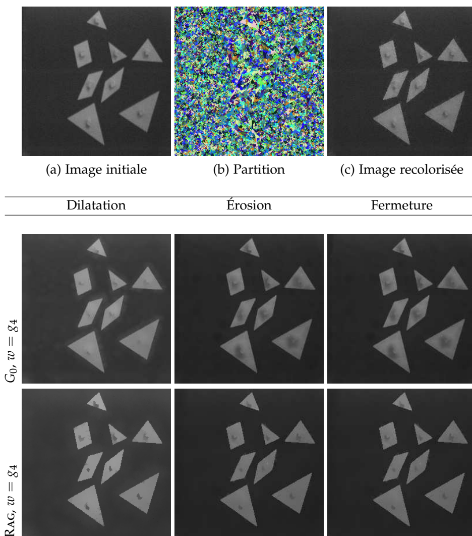
FIG. 4.6: Extension de la dilatation, de l'érosion et de la fermeture sur graphe de régions. (a) : image initiale (65 536 pixels). (b) : partition calculée à partir de (a) (11 853 régions soit 82% de réduction). (c) : image reconstruite à partir de la partition et de la valeur moyenne des régions. Deuxième ligne : résultats avec un graphe grille en 4-voisinage ( G_0 ). Dernière ligne : résultats avec un RAG.
