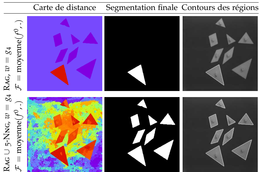
FIG. 5.7: Segmentation non locale d'image avec graphes basés régions. (a) : image initiale (65 536 pixels) et marqueurs originaux en blanc. (b) : partition calculée à partir de (a) (1 324 régions soit 98% de réduction). (c) : image reconstruite à partir de la partition et la valeur moyenne des régions. Dans la seconde partie de cette figure : à la première ligne, résultats obtenus avec un RAG à la seconde ligne, résultats obtenus avec un \text{RAG} \cup 5\text{-NNG} . Les deux graphes sont construits à partir de la partition et de l'image recolorisée. Pour chaque cas, de gauche à droite : la carte de distance, la segmentation calculée par seuillage et les contours des régions obtenues superposés en blanc sur l'image initiale.
