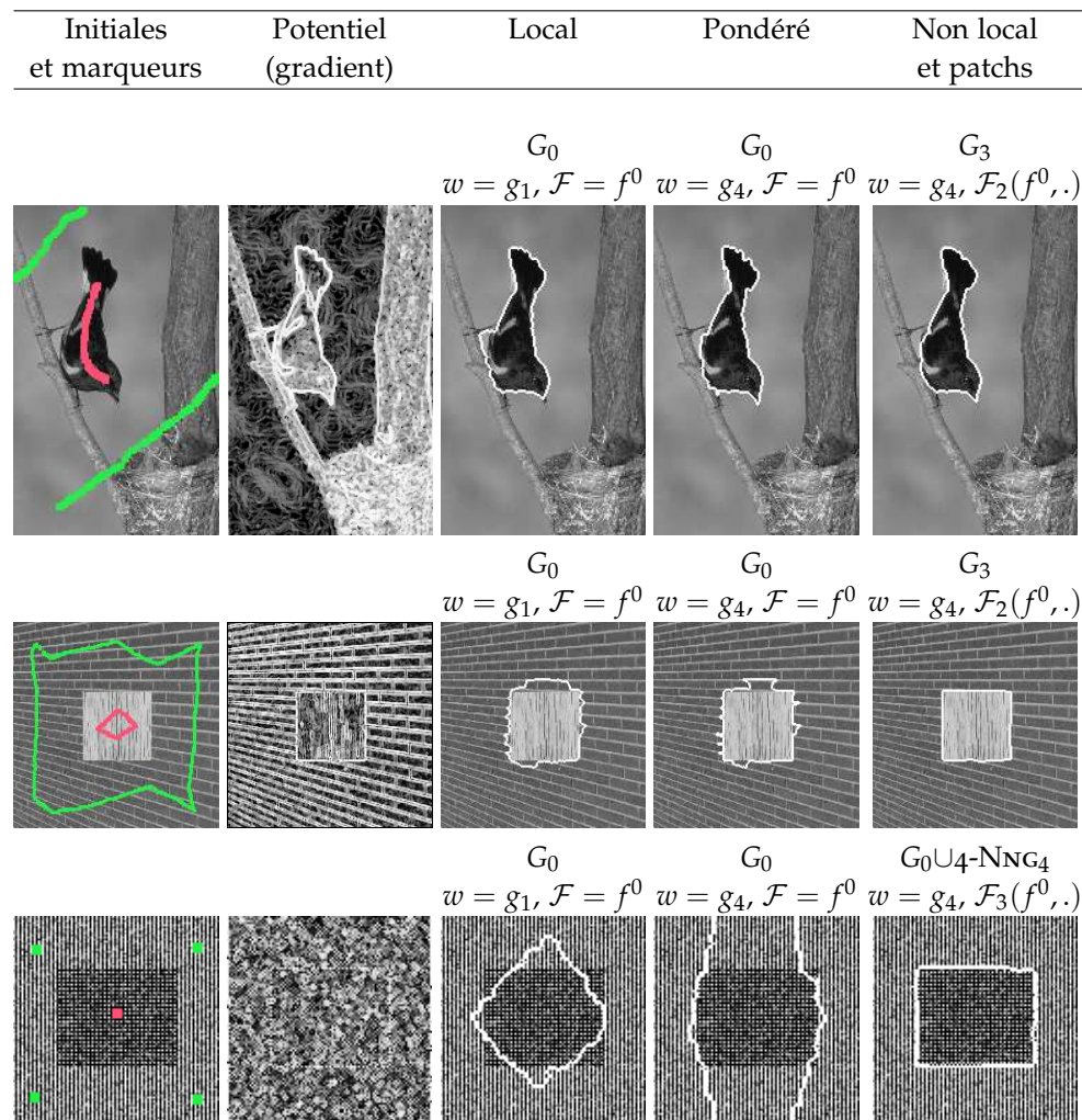
FIG. 5.5: Segmentation d'images avec l'équation eikonale avec différentes structures de graphes. À chaque ligne et de gauche à droite : l'image initiale avec les marqueurs superposés (la couleur verte représente l'arrière plan et la couleur rouge l'objet à extraire); l'image de gradient utilisée comme potentiel P ; les résultats obtenus (avec les différents graphes spécifiés) où les contours des régions trouvées sont superposées en blanc. Les images initiales sont définies comme des fonctions f^0 : V \subset \mathbb{Z}^2 \rightarrow \mathbb{R} .
