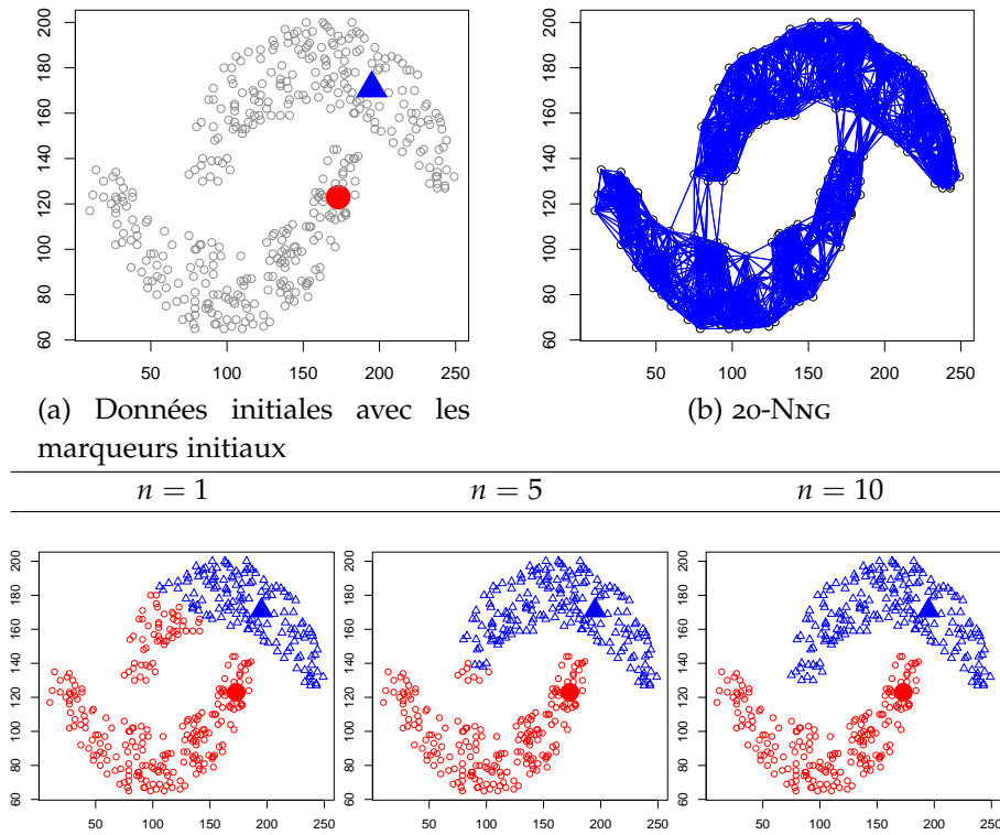
FIG. 3.16: Exemple de propagation de labels sur un nuage de points pour la classification semi supervisée de données. (a) : données initiales avec les marqueurs initiaux et (b) : le graphe associé. À la dernière ligne : évolution de la classification en fonction du nombre d'itérations n .
