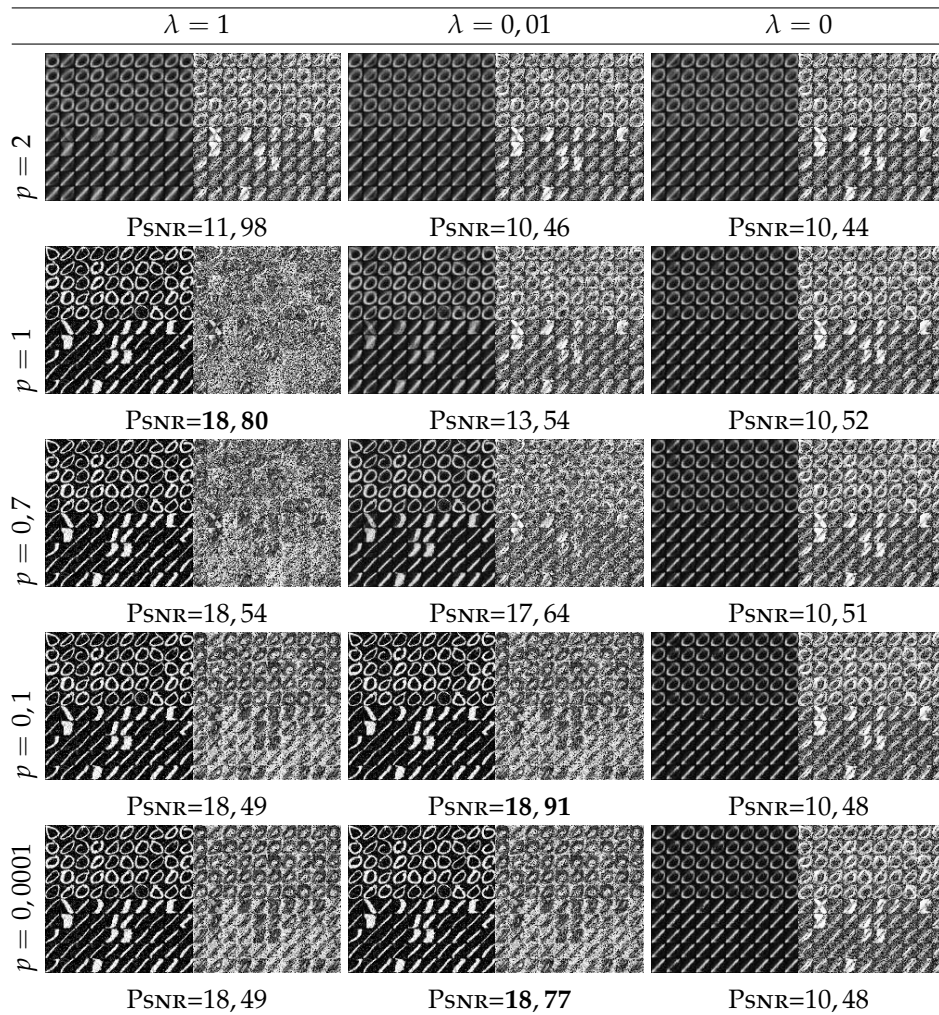
FIG. 3.2: Filtrage isotrope d'une variété d'image (base USPS) avec différentes valeurs des paramètres p et \lambda . Les données filtrées sont celles de la figure 3.1. Chaque résultat présente le résultat du filtrage (la fonction finale f ), la différence avec les données initiales ( |f^0 - f| ) et une valeur de PSNR.
