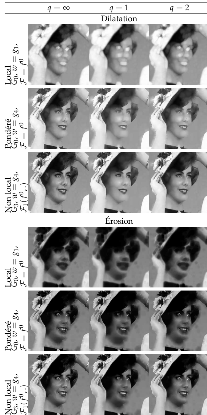
FIG. 4.3: Dilatation et érosion avec différentes valeurs de q , de fonctions de poids w et de topologies de graphe G . Pour chaque opération : local non pondéré (première ligne); local pondéré (deuxième ligne); non local avec des patches (dernière ligne). En colonne, de gauche à droite : q = \infty , q = 1 et q = 2 .
