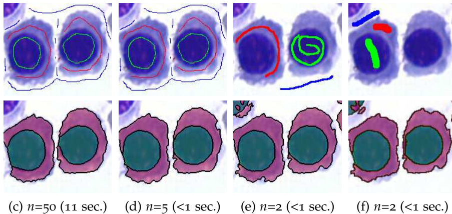
FIG. 3.22: Segmentation semi supervisée et comparaison avec différentes structures de graphes. De gauche à droite : les structures de graphes sont les suivantes. (c) : graphe grille en 8-voisinage ; (d) : RAG calculé à partir de la partition (b) ; (e) et (f) : graphes complets calculés à partir de la partition (b).
