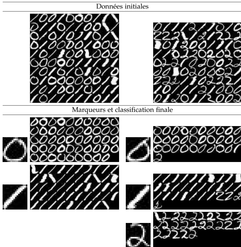
FIG. 5.9: Classification de variétés d'images avec l'équation eikonale. Chaque colonne présente deux exemples différents. Dans la première partie : les données initiales définies comme des fonctions f^0 : V \subset \mathbb{R}^m \rightarrow \mathbb{R}^{256} . Dans la seconde partie, pour chaque exemple : les marqueurs (à gauche) et les résultats de la classification (à droite) en accord avec le marqueur initial.
