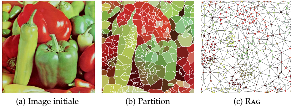
FIG. 2.3: Exemple de graphe d'adjacence des régions associé à une partition d'une image. (a) : image initiale. La partition (b) est représentée avec les contours de ses régions (en blanc) et chaque région est caractérisée par la couleur moyenne des pixels de l'image initiale qui la compose. Chaque sommet du graphe (c) correspond à une région de la partition et est représenté par sa couleur.
