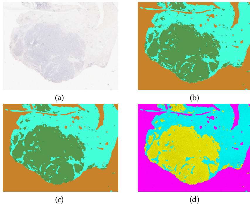
FIG. 3.29: Segmentation du deuxième niveau de la pyramide représentant la lame entière 3.27. (a) : filtrage par régularisation isotrope, (b) : classification par k moyennes ( k=2 ), (c) : classification semi supervisée pour affiner les contours et (d) : segmentation finale superposée sur l'image initiale.
