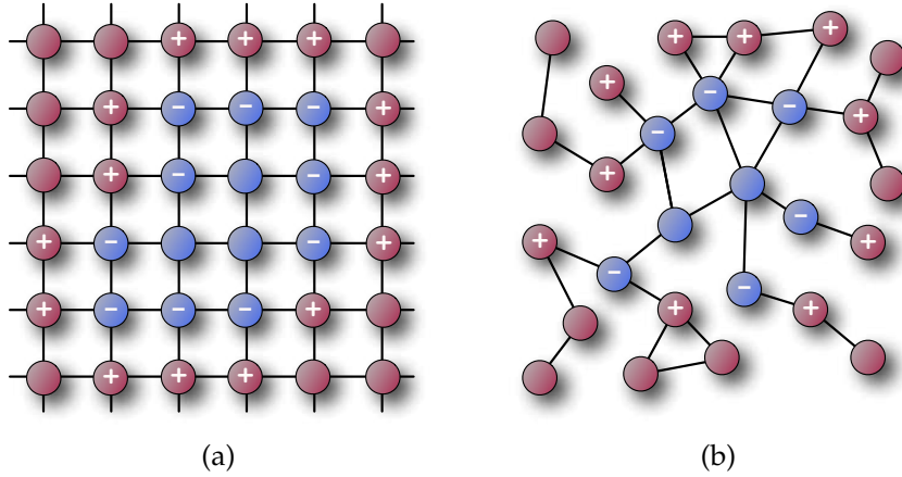
FIG. 2.6: Illustrations des bords d'un graphe sur deux graphes différents. (a) : un graphe grille en 4-voisinage ; (b) : un graphe non orienté quelconque. Les sommets en bleu correspondent à l'ensemble \mathcal{A} . Les sommets marqués par le signe « - » correspondent au bord interne \partial^- \mathcal{A} et ceux marqués par le signe « + » correspondent au bord externe \partial^+ \mathcal{A} .
