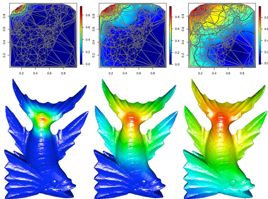
FIG. 5.2: Propagation et évolution de fronts sur un graphe de Delaunay et un maillage 3D. (a) et (b) : graphes originaux. Sur chaque ligne et de gauche à droite : évolution du front pour Les marqueurs initiaux sont représentés par un disque noir sur les graphes originaux. Chaque résultat correspond à une carte de distance. La dernière colonne correspond à la carte de distance finale.
