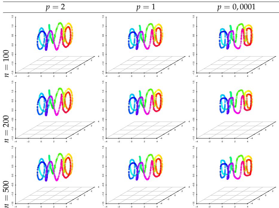
FIG. 3.4: Évolution (en fonction du nombre d'itérations n ) du filtrage isotrope d'une variété avec différentes valeurs des paramètres p et \lambda = 1 . Les données traitées correspondent à celles représentées par la figure 3.3 page 59.
