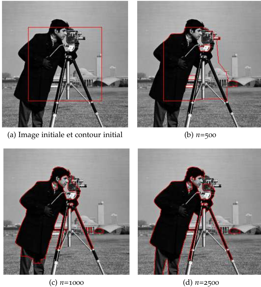
FIG. 3.32: Modèle discret de C_v défini sur des graphes appliqué à la segmentation d'images. Les images (b), (c) et (d) présentent l'évolution de la courbe initiale représentée en rouge pour un nombre n d'itérations de l'algorithme 4.
