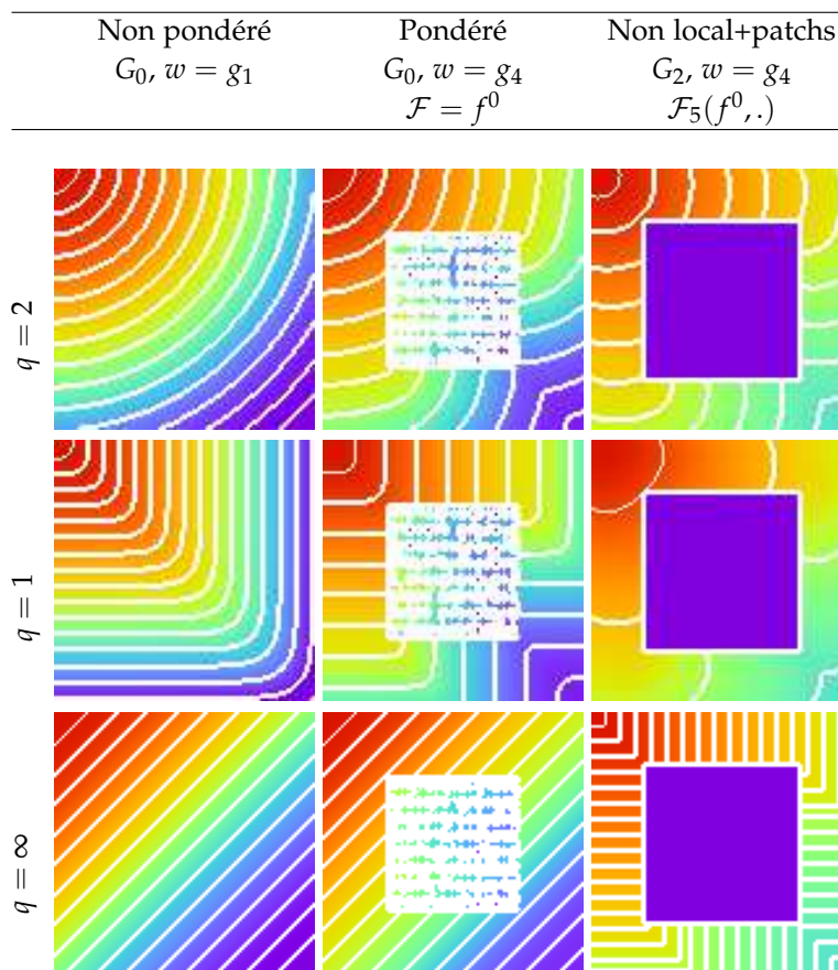
FIG. 5.1: Calculs de distances adaptatifs avec différentes valeurs de q , de fonctions de poids w et de topologies de graphe G . (a) : l'image initiale. À la première, la deuxième et la dernière ligne respectivement : cas où q = 2 , q = 1 et q = \infty . Chaque colonne présente des résultats obtenus avec des structures de graphes et des fonctions de poids différentes calculée à partir de (a). Chaque résultat correspond à une carte de distances où les iso-contours sont superposés. Le marqueur initial correspond à un pixel qui est situé dans le coin en haut et à gauche de l'image initiale.
