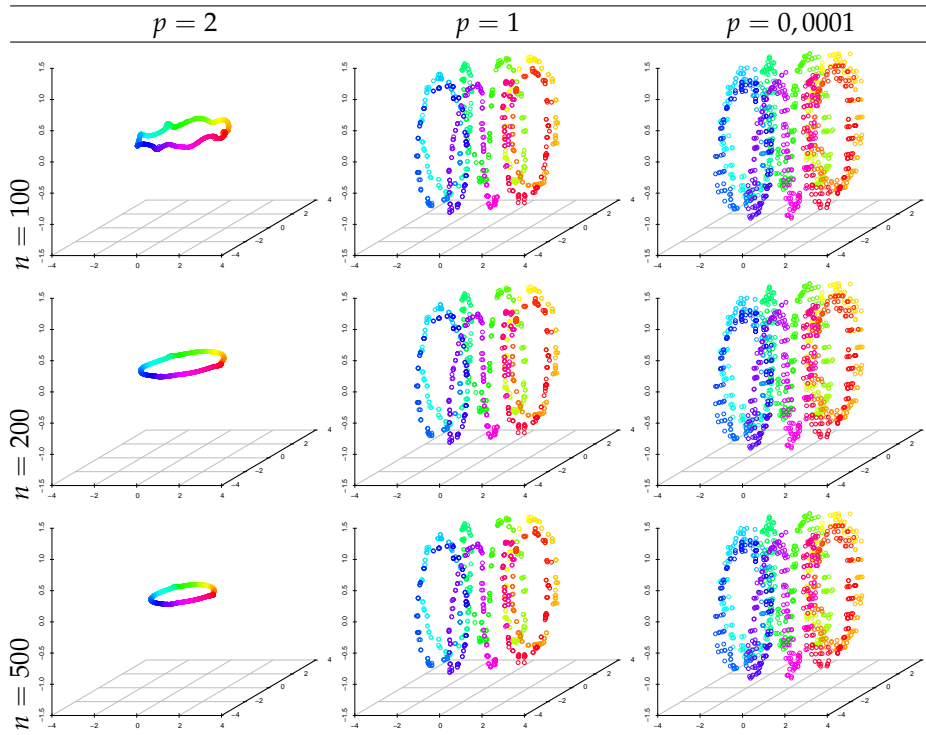
FIG. 3.11: Évolution (en fonction du nombre d'itérations n ) du filtrage anisotrope de la variété avec différentes valeurs des paramètres p et \lambda = 0 . Les données traitées correspondent à celles représentées par la figure 3.3 page 59.
