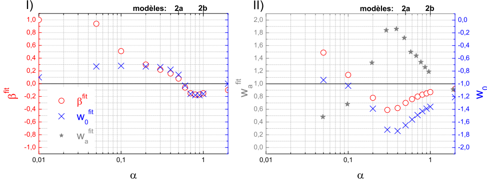
FIGURE 6.1: Valeurs centrales des paramètres \beta (rouge) et w_x (bleu), cas I), et des paramètres \beta (rouge), w_0 (bleu), et w_a (gris), cas II), pour les modèles 2 en fonction du paramètre \alpha .
