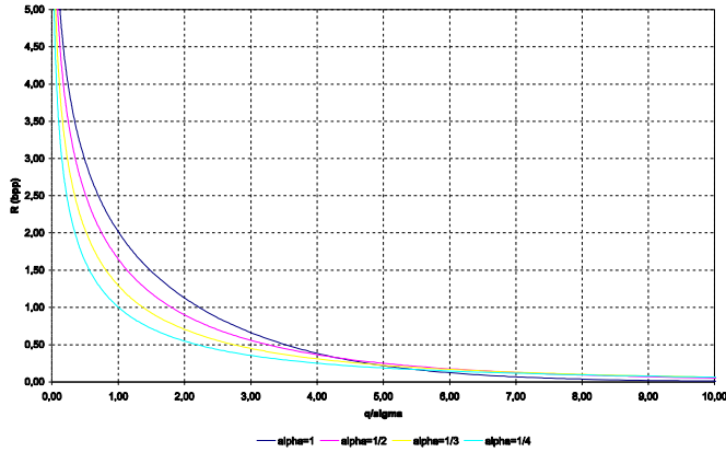
FIG. 3.2 – Débit R pour un quantificateur scalaire uniforme sans zone morte ( z = q ) en fonction du pas de quantification q et pour différentes valeurs du paramètre \alpha de la distribution Gaussienne généralisée.
