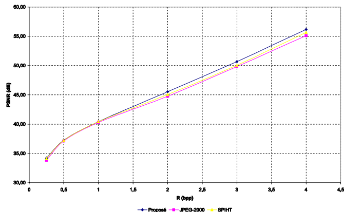
FIG. 3.6 – Rapport Signal-à-Bruit pic en fonction du débit pour l'image LENA (8 bpp–512 × 512 pixels). 3 niveaux de décomposition pour la transformée en ondelettes.
