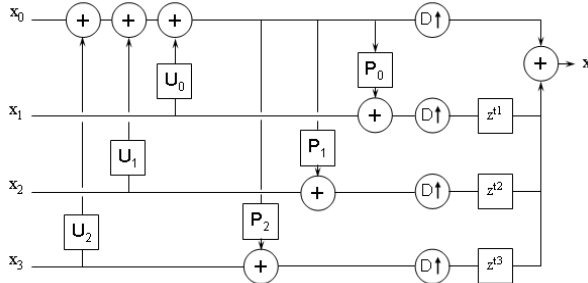
FIG. 2.11 – Schéma lifting de synthèse sur 4 canaux. Les opérateurs p_i et u_i sont respectivement le prédicteur et la mise à jour pour le sous-signal x_i .
