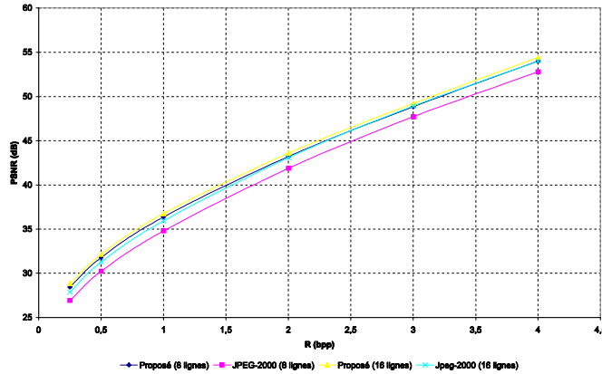
FIG. 3.10 – Rapport Signal-à-Bruit pic en fonction du débit pour l’image NIMES (8 bpp–512 × 512 pixels). 3 niveaux de décomposition pour la transformée en ondelettes. Compression au “fil de l’eau” avec la méthode proposée EBWIC sur des zones de traitement de tailles 8 lignes et 16 lignes image. Comparaison avec JPEG-2000 en mode tuilé avec des tuiles de tailles 8 et 16 lignes image.
