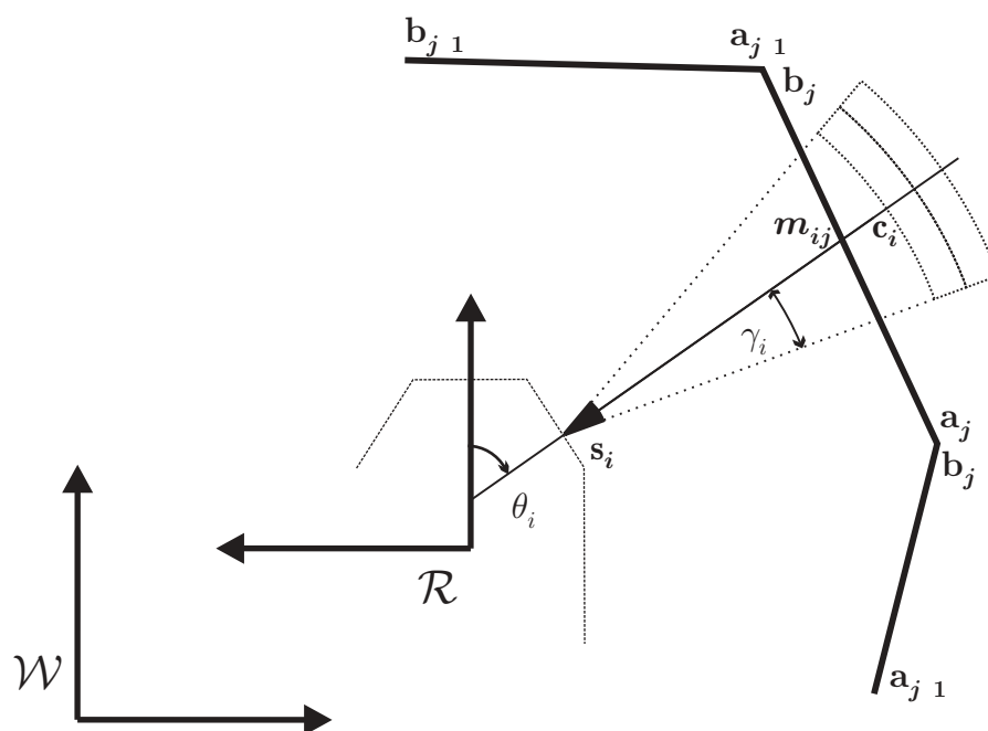
Figure 4-11: Le test leg_{in_i} vaut faux.
