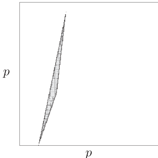
Figure 3-20: Ensemble des p admissibles et incertains avec une borne e = 0.035 obtenue par Meboe.
