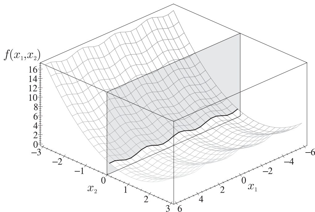
Figure 3-8: Représentation de f(\mathbf{x}) = \sin^2(x_1 - 1) + (x_2 - 1)^2 sur [-6, 6] \times [-3, 3] .
