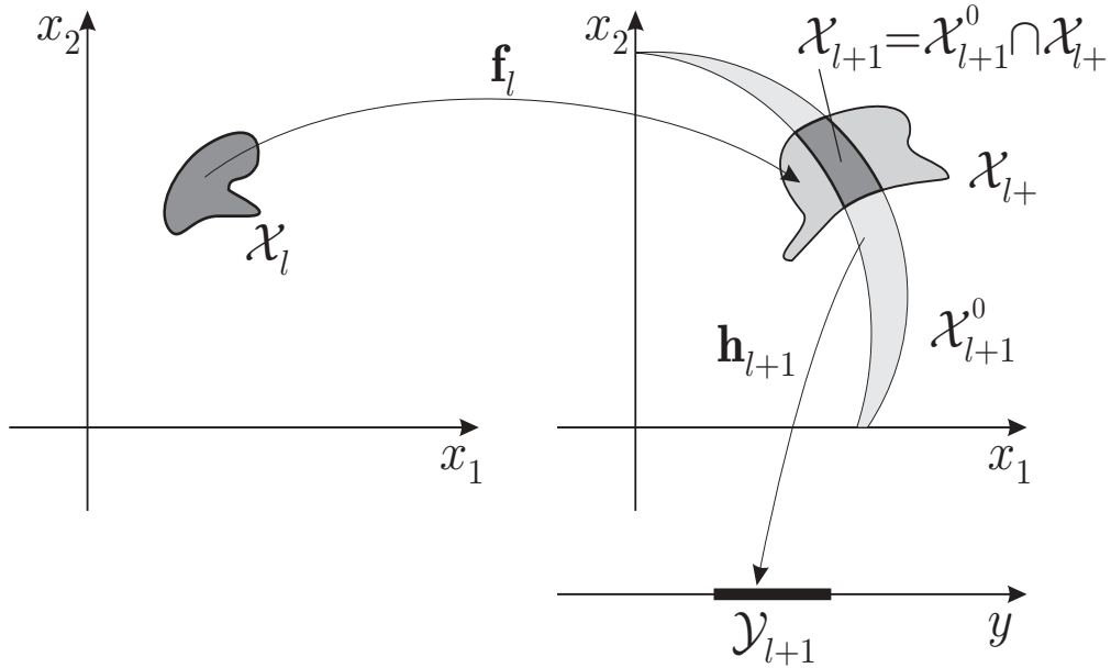
Figure 5-1: Principe de l'algorithme d'estimation d'état idéalisé. \mathcal{X}_l est l'état à l'instant l . \mathcal{X}_+ est l'état prédit à l'instant l+1 . Une mesure \mathcal{Y}_{l+1} est faite à l+1 , \mathcal{X}_{l+1}^o est l'ensemble des états ayant pu conduire à une mesure appartenant à \mathcal{Y}_{l+1} . Par conséquent, l'état à l'instant l+1 est \mathcal{X}_{l+1}^o \cap \mathcal{X}_+ .
