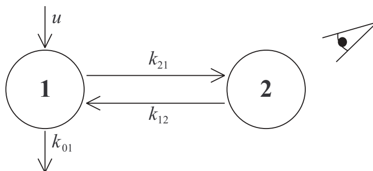
Figure 3-11: Modèle à deux compartiments.
