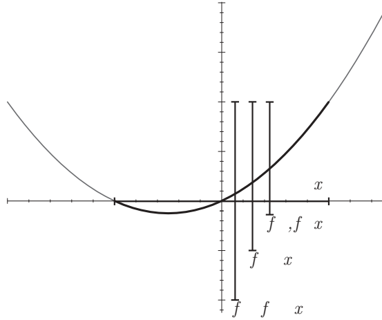
Figure 2-2: Comparaison de fonctions d'inclusion d'une même fonction.
