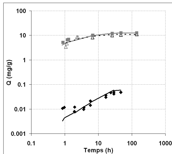
Figure VI.16 Comparaison des cinétiques d'adsorption et de biosorption du NAP. Données expérimentales de cinétique d'adsorption du NAP ( C_0=12\text{ppm} ) sur du CAG PICA S35 ( 1\text{g/L} ) brut (■) et CAG-MO( \Delta ) et données expérimentales de biosorption du NAP ( C_0=1\text{ppm} ) sur de la biomasse en suspension ( [\text{MES}]=6\text{g/L} ) (◆). Les résultats de simulation sont représentés par des traits.
