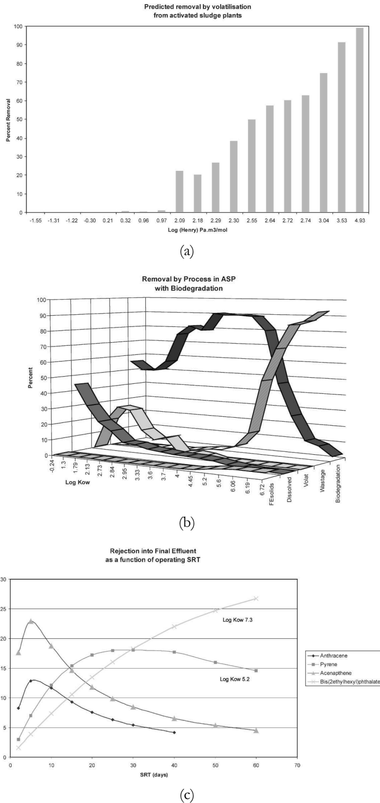
Figure I.8: Résultats de l'étude de Byrns et al. (2001) sur le devenir de micropolluants organiques au sein d'un procédé boue activée: (a) influence de la constante de Henry sur la fraction volatilisée; (b) influence du coefficient de partage octanol-eau sur les fractions sorbées sur les boues contenues dans l'effluent final (FEsolids),dissoutes (dissolved), volatilisée (Volat), sorbées sur les boues purgées (Wastage) et biodégradée (biodegraded), (c) influence de l'âge de boues sur les rejets de 4 HAPs dans l'effluent final
