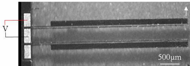
Fig. 5.7. A pair of thermal actuators.
