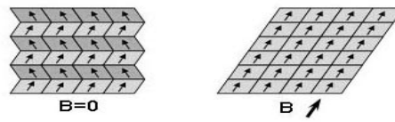
Fig. 1.30. Principle of FSMAs.
