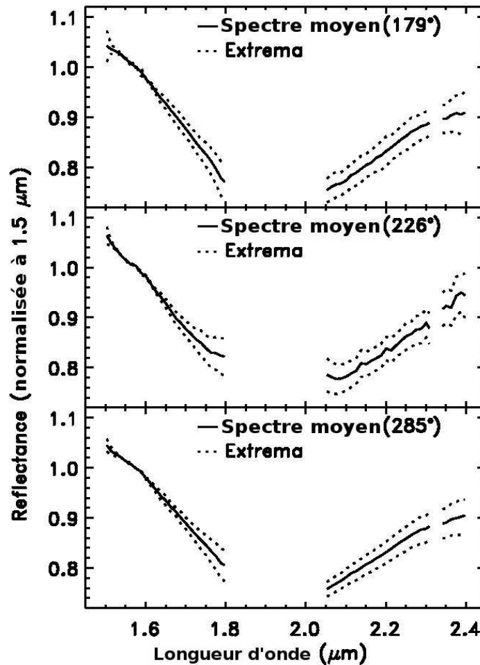
FIG. IV.22: Spectre moyen et extrema normalisés à l'unité à 1.5 \mu\text{m} . Chaque cadre correspond à une géométrie donnée comme reporté sur la figure (voir Table IV.16). L'hétérogénéité de la surface de Vesta se voit ici par les différences forme présenté par la bande à 2 microns (vu ici par l'enveloppe des extrema en traits pointillés).
