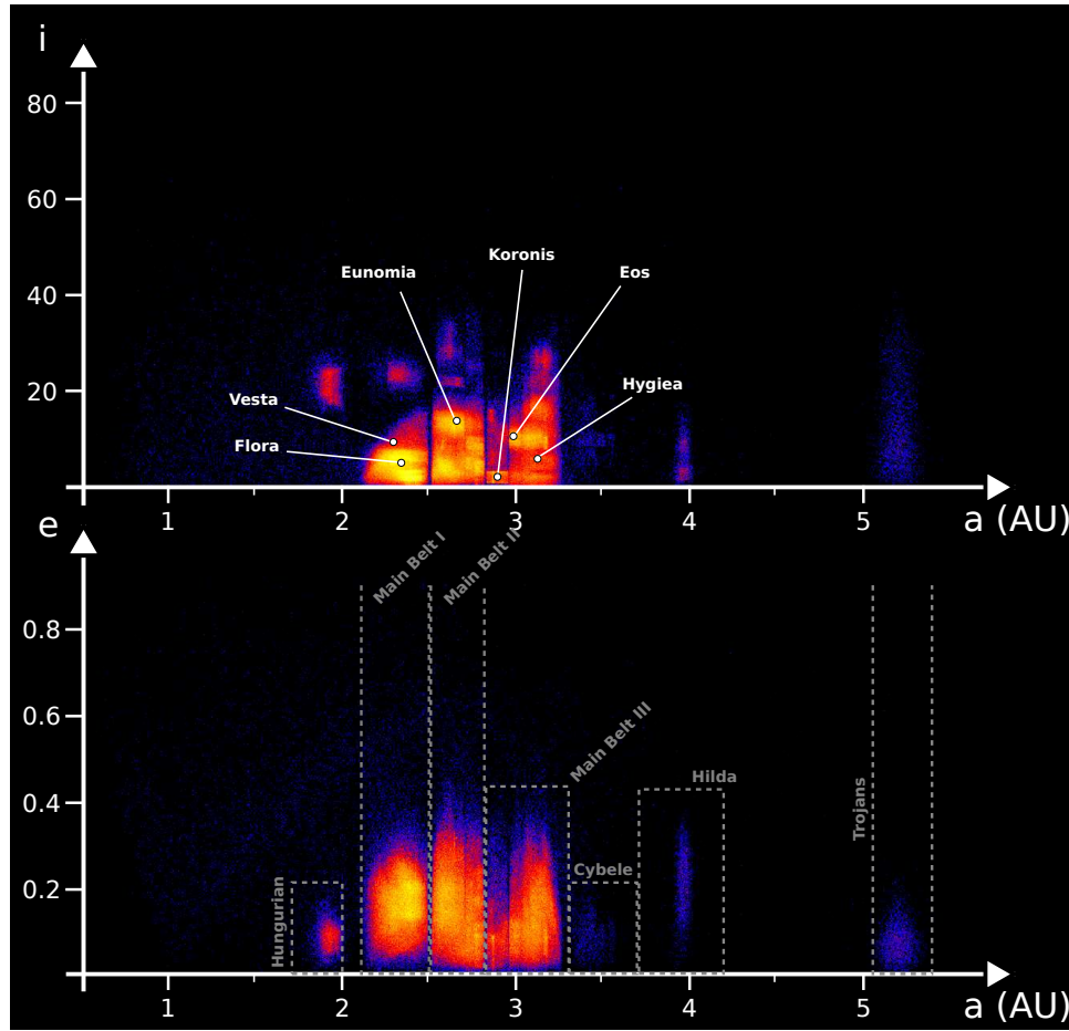
FIG. I.1: Distribution des astéroïdes dans l'espace des éléments orbitaux (a, e, i) . L'échelle de couleur va de l'absence de corps connu (en noir), aux grandes concentrations (en rouge). Les principales familles sont libellées, ainsi que les grandes régions de la ceinture principale. Les gaps où la densité d'astéroïdes est proche de zéro situés autour de 2.5, 2.82, 2.95 et 3.27 UA sont produits par l'action gravitationnelle de Jupiter (lieu de résonances). Il est à noter que si ces gaps apparaissent de manière franche sur cette figure, ils ne correspondent pas à des régions dépourvues d'objet. En effet, une vue de la ceinture principale prise depuis le dessus du plan de l'écliptique montrerait une répartition homogène des astéroïdes.
