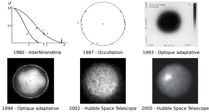
FIG. IV.1: Panorama des observations directes de (1) Cérés. Par interférométrie, Tokovinin [1980] avait évalué une limite inférieure au diamètre de Cérés (courbe de visibilité du haut) de 981 km. L’occultation de BD+8°471 [Millis et al., 1987] montra que Cérés était bien représenté par un ellipsoïde oblongue. Néanmoins, la mesure des trois axes n’était que marginale, trois occultations étant nécessaires pour contraindre complètement le système [Drummond and Cocke, 1989]. Les années 90 virent l’apparition de l’OA, mais les premières observations [Saint-Pé et al., 1993a] ne permirent pas de mesures précises. Il faudra attendre la fin des années 90 pour obtenir la première détermination basée sur toute une nuit d’observation [Drummond et al., 1998]; puis les années 2000 pour les observations HST [Parker et al., 2002; Thomas et al., 2005] et la détection de marques d’albédo.
