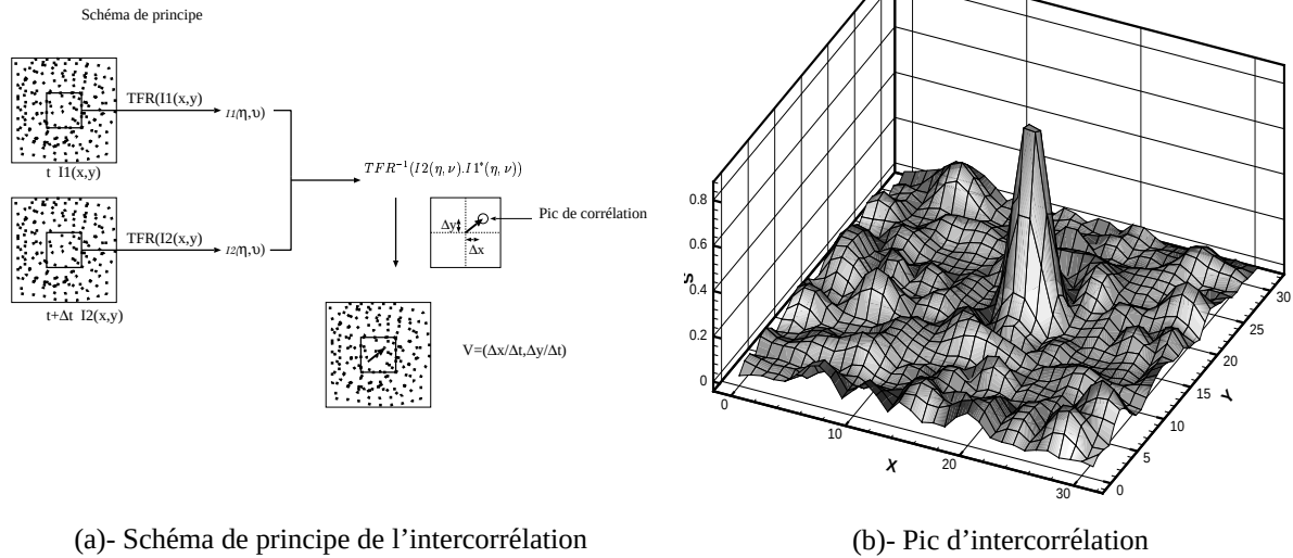
FIG. II.16 – Principe de base de la PIV par intercorrrelation.
