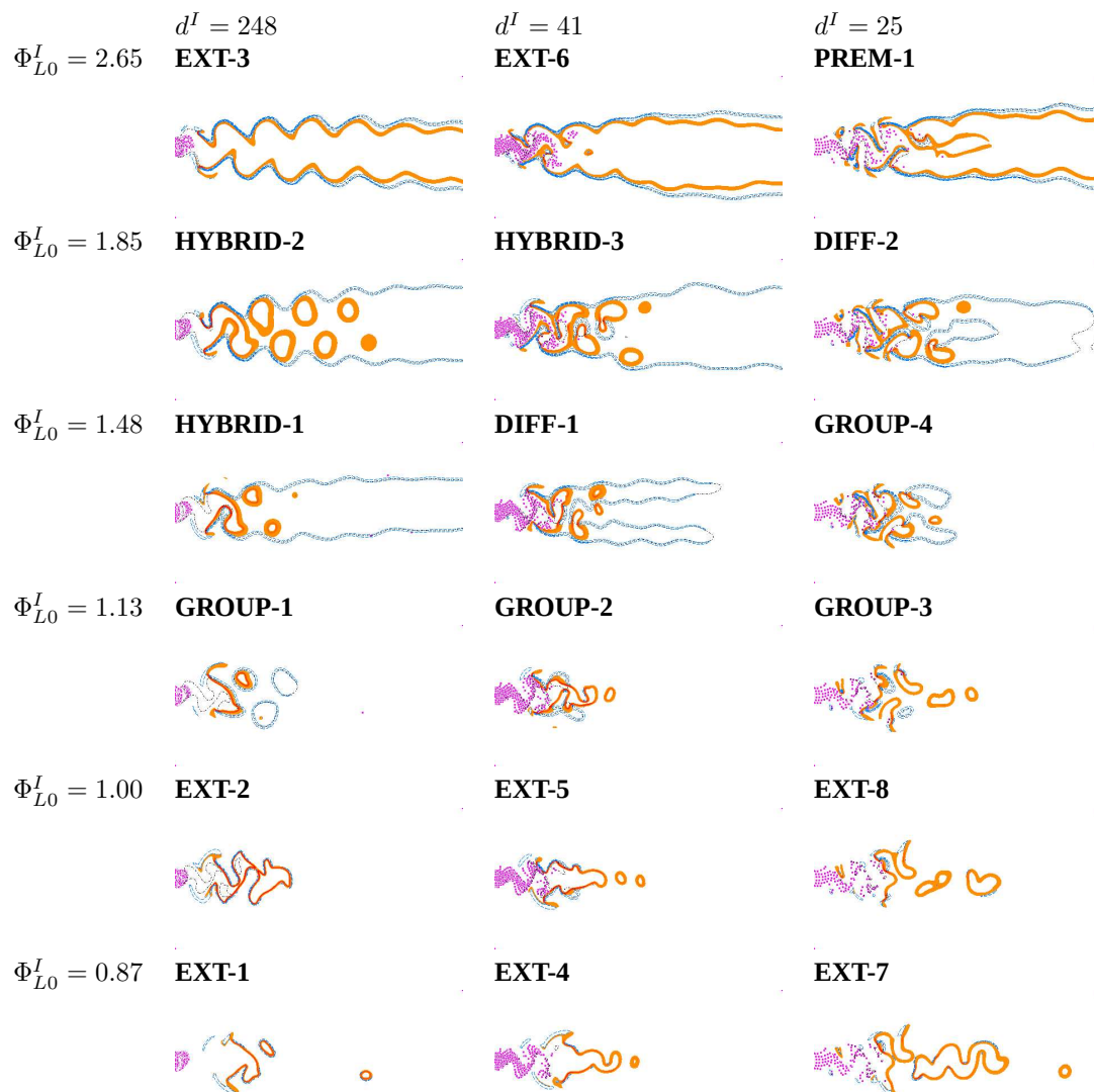
PII.12. - Taux de réaction instantanés de l'ensemble des simulations. Orange: flammes prémélangées, bleu: flammes de diffusion, tirets: iso-stoichiométrie de la fraction de mélange.
