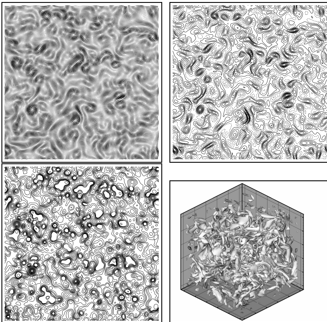
PII.21. - Résultats des simulations 2D et 3D après 10 temps de retournement. Haut gauche, vecteurs vitesse (2D); haut droit, champ de vorticit  (2D); bas gauche, champ de pression (2D); bas droit: chmapr de vorticit  (3D).
