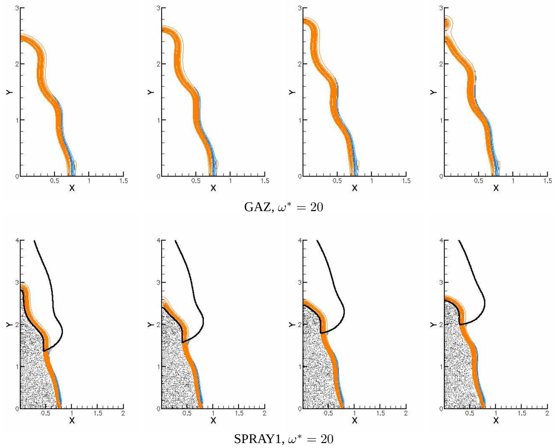
PII.17. - Taux de réaction (orange: prémélange, bleu: diffusion) des différentes flammes avec contours de la fraction de mélange Z (ligne épaisse: Z_{stoechio} , tirets: Z riche, ligne continue: Z pauvre). Haut: cas GAZ, pulsation réduite \omega^* = 20 , bas: cas SPRAY1, pulsation réduite \omega^* = 20 .
