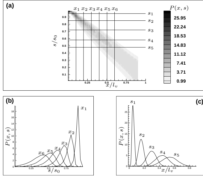
PII.1.a - Iso-contours (haut) et profils (bas, gauche et droite) de la PDF P(x, s) . Un comportement similaire est observé dans l'ensemble des simulations. Les profils sont tracés selon s (en bas à gauche) et x (en bas à droite) pour différentes positions indiquées sur la figure du haut. x_1/l_v = 0.09 , x_2/l_v = 0.20 , x_3/l_v = 0.30 , x_4/l_v = 0.41 , x_5/l_v = 0.52 , x_6/l_v = 0.62 , et s_1/s_0 = 0.95 , s_2/s_0 = 0.85 , s_3/s_0 = 0.72 , s_4/s_0 = 0.58 , s_5/s_0 = 0.48
