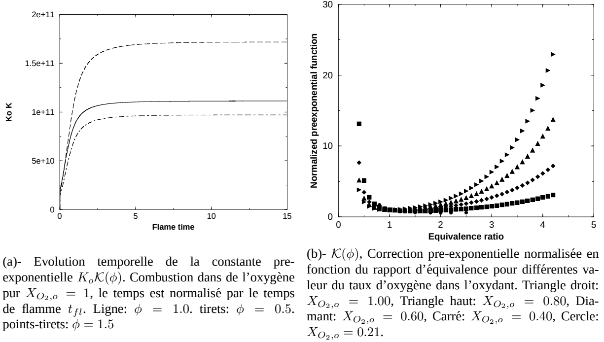
FIG. II.15 – Convergence des paramètres chimiques.
