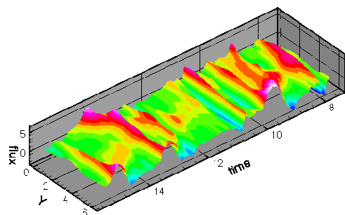
PII.7.a - Flux de chaleur instantané, simulation monophase BASE
