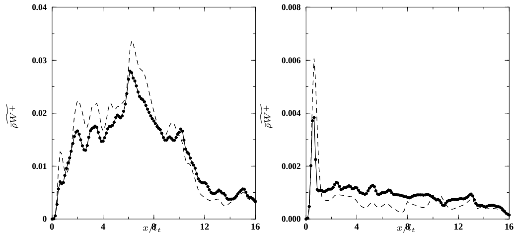
FIG. II.5 – Evaluation du modèle pour le terme source massique, \widetilde{W}^+ . Symboles : données DNS, modèle : tirets. Gauche : évaporation lente, droite : évaporation rapide
