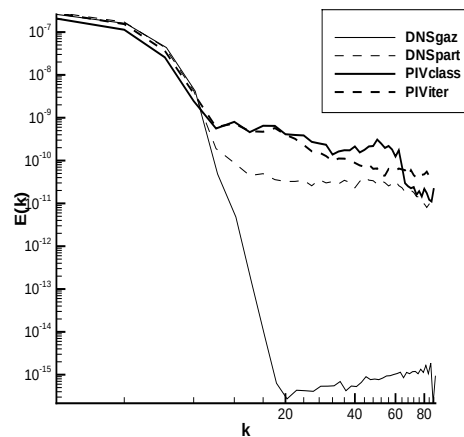
PII.24.b - Spectres de la turbulence
