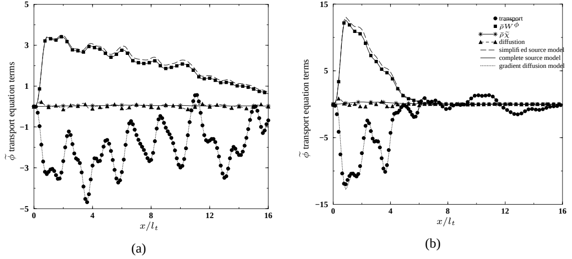
FIG. II.7 – Evolution spatiale des différents termes de l'équation d'évolution de \tilde{\Phi} = \widetilde{Z(1-Z)} . Symboles: DNS, lignes: modèles. figure (a): évaporation lente, figure (b): évaporation rapide.
