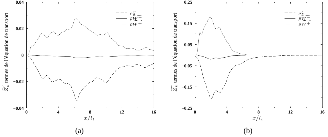
FIG. II.4 – Evolution spatiale du taux de dissipation \widetilde{\chi} (tirets) et des termes sources \widetilde{W}^+ (ligne pointillée) et \widetilde{W}^- (ligne continue). Figure (a) : évaporation lente, figure (b) : évaporation rapide.
