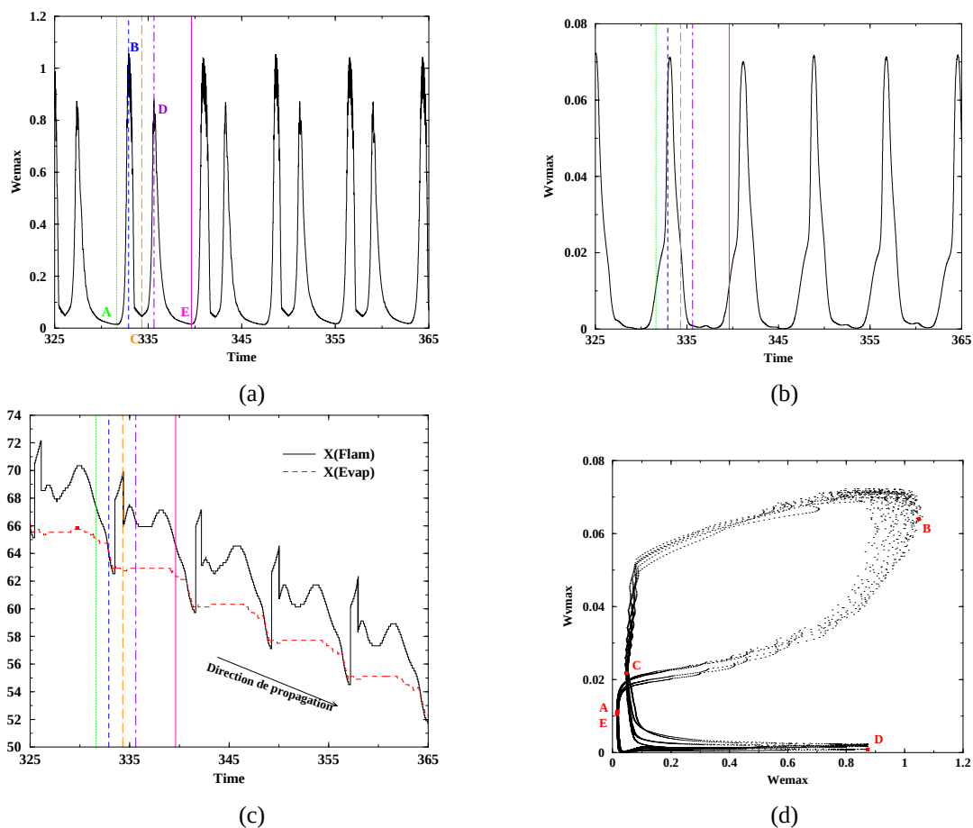
PII.8. - Propagation d'une flamme monodimensionnelle au sein d'un spray riche en combustible liquide. (a) Evolution du taux de réaction maximum au cours du temps. (b) évolution du taux d'évaporation maximum au cours du temps, (c) évolution des positions des taux de réaction et taux d'évaporation maximums au cours du temps, (d) évolution du taux d'évaporation maximum en fonction du taux de réaction maximum.
