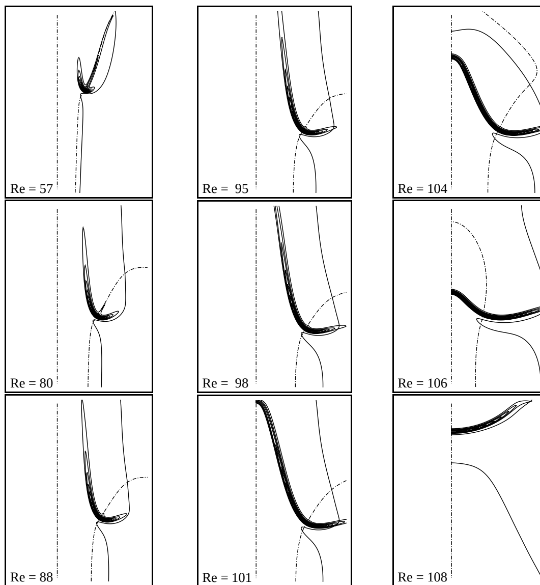
PII.20. - Structures des flammes liftées pour différents nombres de Reynolds. Visualisation du taux de dégagement de chaleur. Ligne verticale pointillée: axe de symétrie, ligne pointillée: iso-stœchiométrie de la fraction de mélange, ligne continue : iso-vitesse de flamme laminaire, axe horizontal : direction radiale, axe vertical: direction de l'écoulement.
