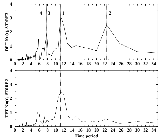
PII.5.c - Transformée de Fourier discrète du signal de transfert de chaleur exprimé en terme de période de temps de jet. Haut: Re_J = 1350 (ST0-RE3) et bas: Re_J = 900 (ST0-RE2).
