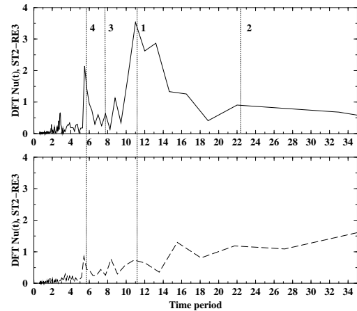
PII.6.c - Transformée de Fourier discrète du signal de tranfert de chaleur exprimé en terme de période de temps de jet. Haut: Re_J = 1350 (ST2-RE3) et bas: Re_J = 1350 (ST2-RE2).
