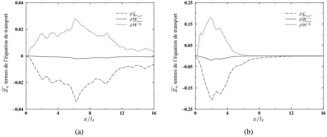
FIG. II.4 – Evolution spatiale du taux de dissipation \tilde{\chi} (tirets) et des termes sources \tilde{W}^+ (ligne pointillée) et \tilde{W}^- (ligne continue). Figure (a) : évaporation lente, figure (b) : évaporation rapide.
