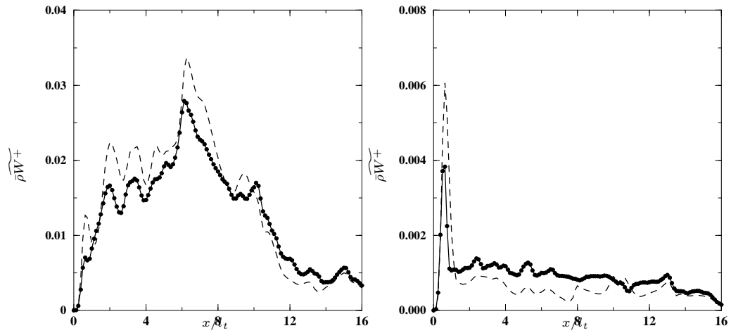
FIG. II.5 – Evaluation du modèle pour le terme source massique, \widetilde{\rho W^+} . Symboles : données DNS, modèle : tirets. Gauche : évaporation lente, droite : évaporation rapide
