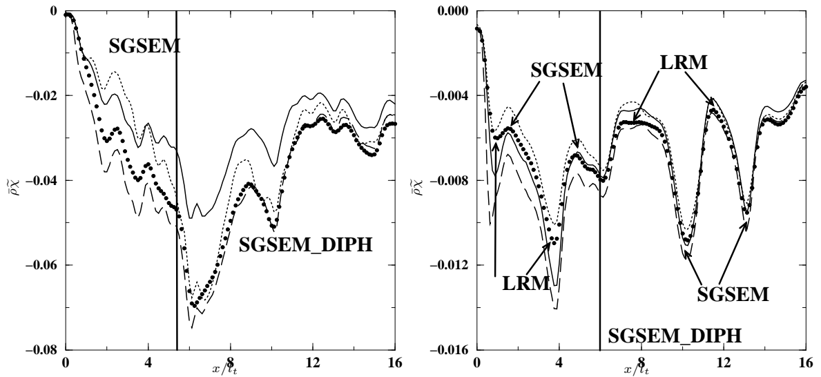
FIG. II.6 – Comparaison des modèles permettant la détermination du taux de dissipation de sous-maille : \widetilde{\chi} . Symboles : données DNS, pointillés : modèle LRM, ligne continue : SGSEM, tirets : SGSEM-DIPH. Gauche : évaporation lente, droite : gouttes légères.
