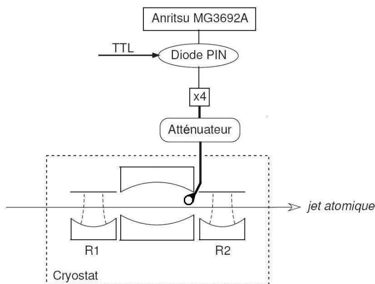
FIG. II.18 – Schéma du dispositif d'injection dans les cavités de grande finesse.
