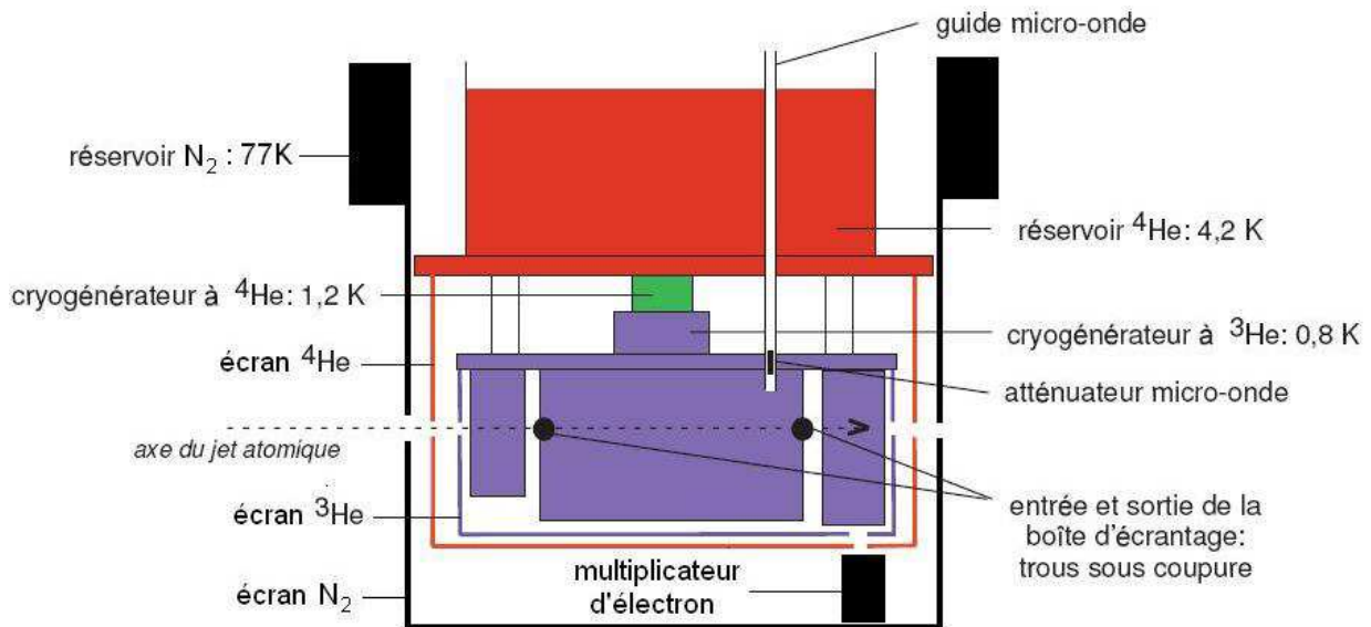
FIG. II.19 – Schéma du cryostat utilisé pour maintenir les cavités à 0,8 K et pour maintenir cette température le long du trajet des atomes de Rydberg circulaires.
