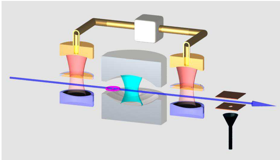
FIG. 2 – Schéma de principe de nos expériences d'électrodynamique quantique en cavité. La cavité de grande finesse est insérée dans un interféromètre de Ramsey formé de deux cavités de faible facteur de qualité. Les atomes de Rydberg traversent un à un l'interféromètre avant d'être détectés par ionisation.
