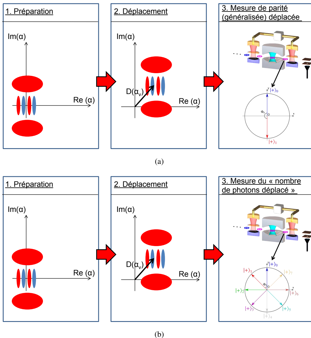
FIG. IV.19 – Schéma de principe de la procédure de reconstruction. La mesure a lieu en 3 étapes successives. La dernière étape consiste à mesurer le champ déplacé par interférométrie atomique. (a) Les données expérimentales dont nous disposons ont été prises avec un réglage voisin de celui de la mesure de parité (voir III.4.2). (b) Il est plus avantageux d'utiliser un réglage permettant de distinguer parmi un grand nombre d'états de Fock (voir III.4.4).
