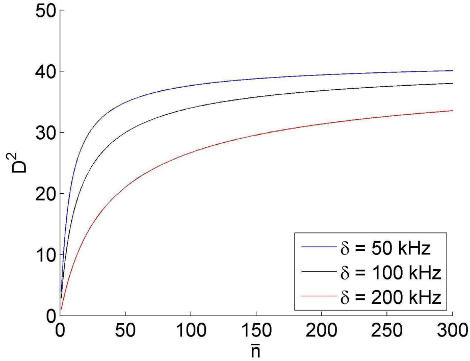
FIG. V.9 – Taille de la superposition produite (en nombre de photons) en fonction du nombre de photons dans le champ cohérent injecté pour différentes valeurs du désaccord atome-champ.
