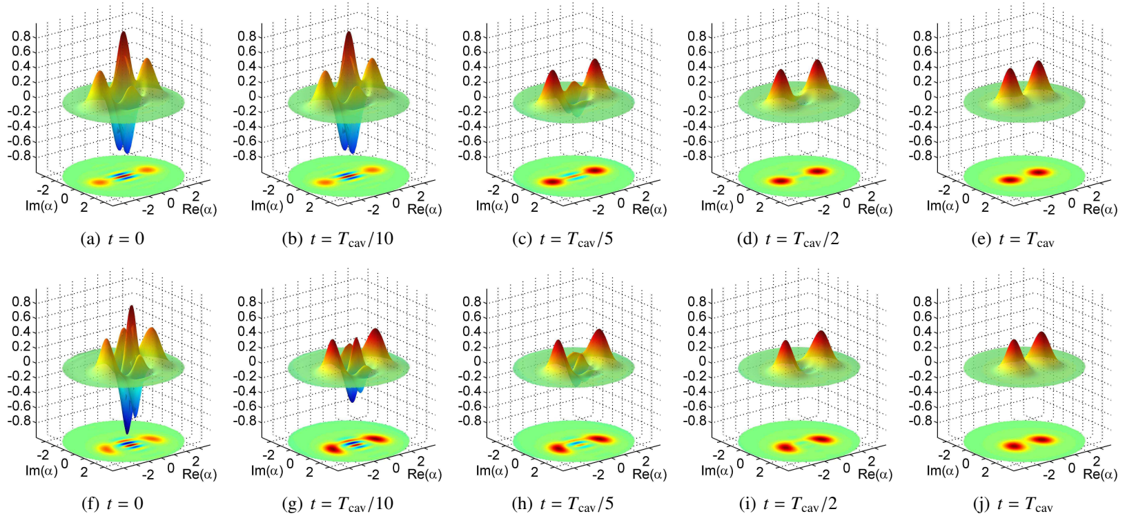
FIG. V.1 – La première ligne représente l'évolution de la fonction de Wigner d'un état chat de Schrödinger maximalement séparé dans un environnement à température nulle tel que décrit par la solution analytique (V.32) pour \alpha = \sqrt{3,5} . La deuxième ligne montre la même évolution pour un chat produit à l'aide d'un atome désaccordé de 51 kHz par rapport à la fréquence de la cavité interagissant avec un champ cohérent d'amplitude \alpha = \sqrt{3,5} . Cette fois, on considère la situation réaliste où le nombre moyen de photons thermiques dans l'environnement est de 0,05. Les images correspondent aux instants t = 0 , t = T_{\text{cav}}/10 , t = T_{\text{cav}}/5 , t = T_{\text{cav}}/2 et t = T_{\text{cav}} .
