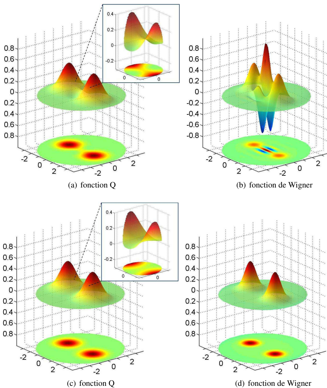
FIG. I.10 – Fonction Q et fonction de Wigner de l'état chat de Schrödinger |\psi_{\text{pair}}\rangle ((a) et (b)) et du mélange statistique \rho_{\text{mélange}} ((c) et (d)).
