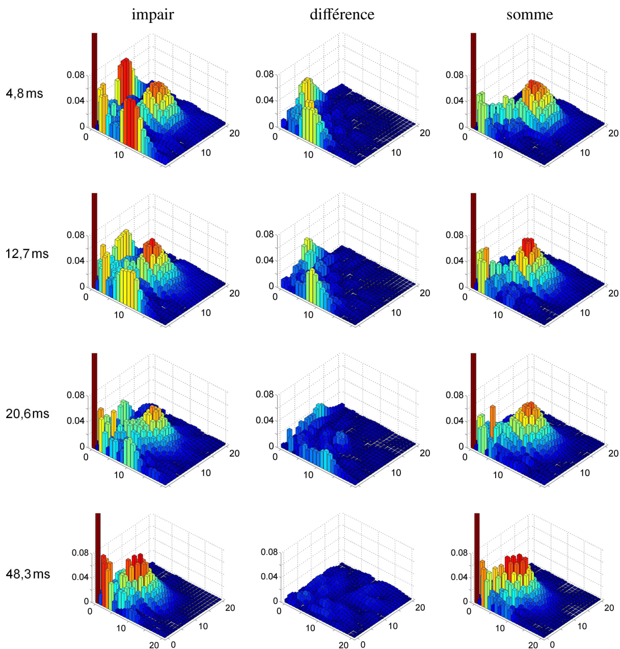
FIG. V.6 – Module des éléments de la matrice densité déplacée (chat impair) reconstruite pour les quatre instants successifs \tau = 4,8 , 12,7 , 20,6 et 48,3 ms. Les éléments \rho_{0,0} , tronqués sur les images sont voisins de 0,38 sur l'ensemble des images.
