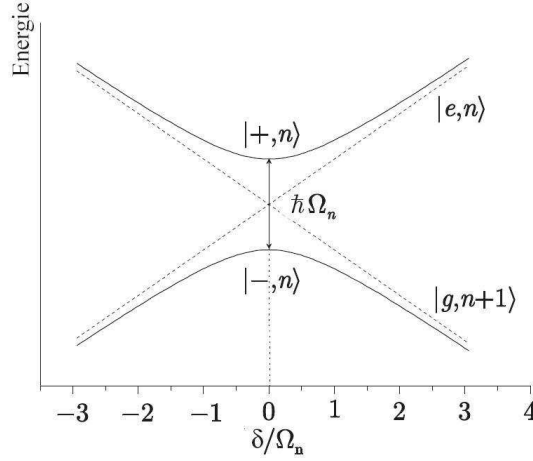
FIG. I.14 – Energie des états habillés en fonction du désaccord atome-champ \delta . Les lignes pointillées représentent l'énergie des états non couplés. L'interaction lève la dégénérescence des niveaux à résonance, formant un anticroisement.
