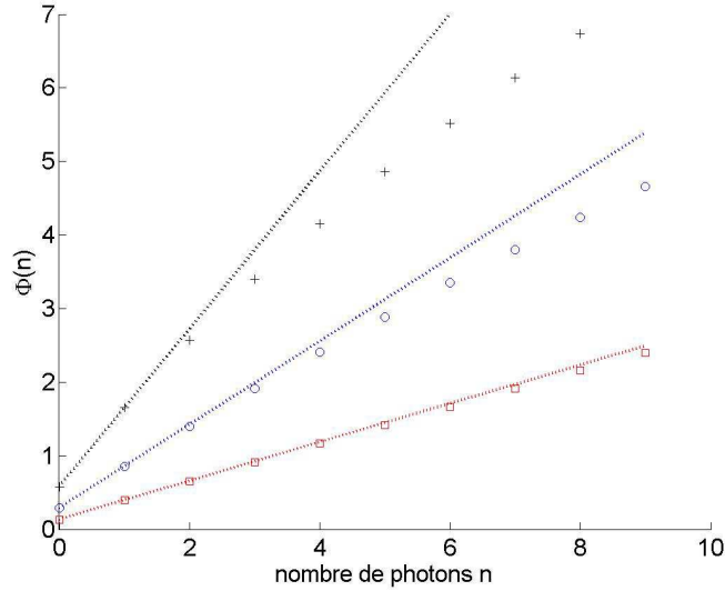
FIG. III.3 – Déphasage \Phi(n)/\pi subi par la superposition atomique en fonction du nombre de photons pour une vitesse v = 250\text{m/s} , et un désaccord \delta = 55\text{ kHz} (croix), 120\text{ kHz} (ronds), 270\text{ kHz} (carrés). Les courbes en traits pointillés correspondent à un ajustement linéaire sur les deux premiers points. L'ordonnée à l'origine de ces différentes courbes correspond au déplacement de Lamb aux différents désaccords \delta .
