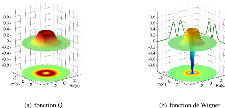
FIG. I.6 – Fonction Q (a) et fonction de Wigner (b) de l'état de Fock |n = 1\rangle
