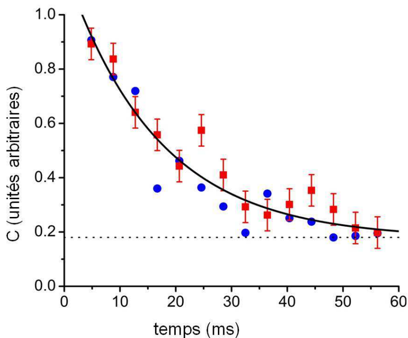
FIG. V.7 – Cohérence C(t) évaluée comme la somme des modules des éléments \rho_{0,n}(\tau) / n \geq 5 . Les points rouges correspondent au chat pair et les points bleus, au chat impair. Les barres d'erreurs (non représentées pour le chat impair pour plus de lisibilité) sont obtenues en effectuant la reconstruction sur des partitions aléatoires des données expérimentales. Le trait noir représente un ajustement exponentiel donnant un temps de décohérence T_D = 17 \pm 3 ms.
