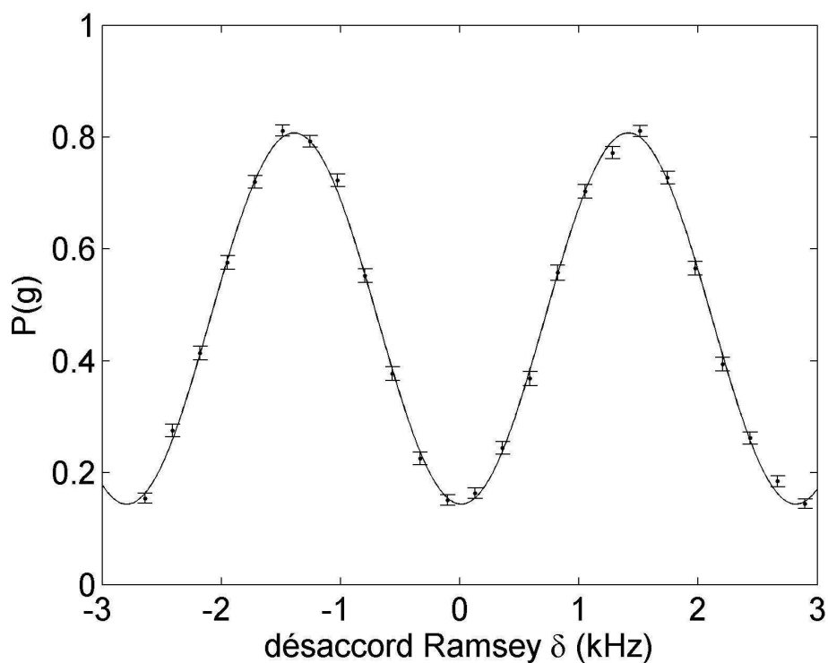
FIG. II.16 – Franges de Ramsey obtenues par interférométrie atomique entre les zones de Ramsey R_1 et R_2 . Les deux impulsions sont séparées de 360,3 \mu\text{s} , soit le temps de transit des atomes entre les deux zones de Ramsey. La courbe en trait plein est un ajustement sinusoïdale. Le contraste mesuré est de 75 %.
