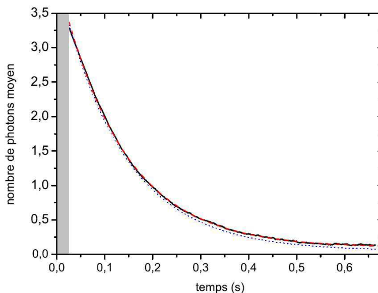
FIG. III.14 – Moyenne sur toutes les réalisations du nombre de photons inféré \langle n \rangle au cours du temps. L'ajustement exponentiel (pointillés rouges) est indistinguable des points expérimentaux. La courbe en pointillés bleus est la prédiction purement théorique. La zone grisée correspond aux 26 premières ms nécessaires à la détection des 110 atomes réalisant la première mesure.
