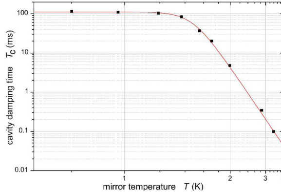
FIG. II.4 – Temps de vie d’une cavit  supraconductrice mesur  en fonction de la temp rature du cryostat. L’ chelle horizontale est r ciproque tandis que l’ chelle verticale est logarithmique.
