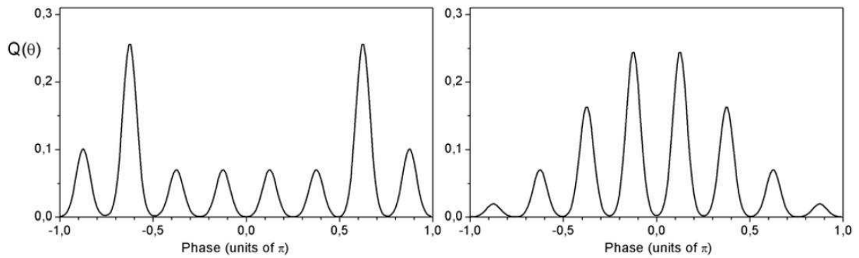
FIG. V.11 – Comparaison entre une marche aléatoire quantique et une marche aléatoire classique dans un système d'électrodynamique quantique en cavité. A gauche, distribution de phase du champ (fonction Q sur un cercle) après 9 étapes d'une marche aléatoire quantique partant d'un champ cohérent contenant 36 photons en moyenne. L'incrément de phase à chaque étape est de \pi/8 . A droite, distribution de phase pour la marche aléatoire classique correspondante obtenue en mesurant l'atome à chaque étape.
