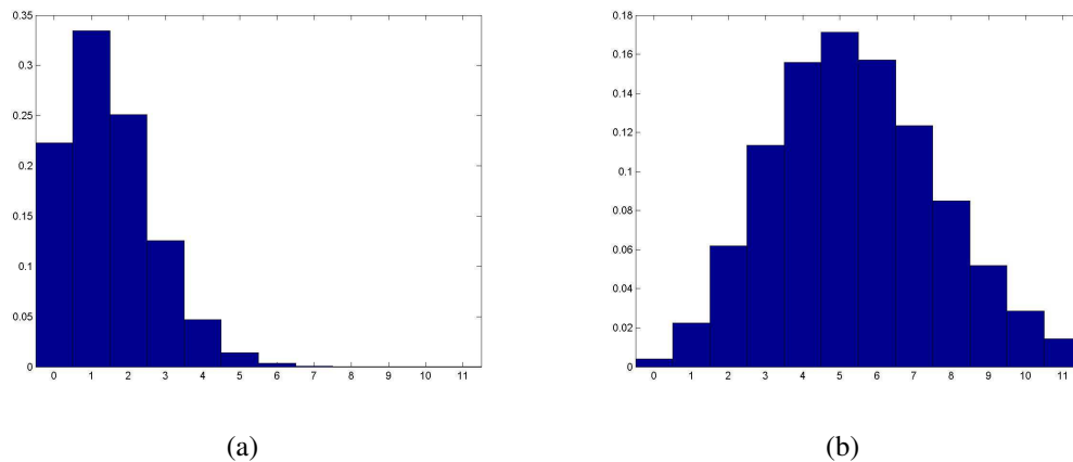
FIG. IV.11 – Population des différents états de Fock dans un champ cohérent contenant (a) 1,5 photons en moyenne, (b) 5,5 photons en moyenne.
