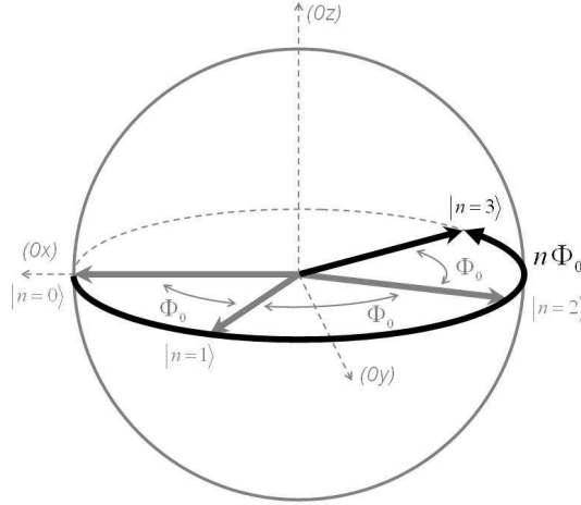
FIG. III.2 – Evolution du vecteur de Bloch lors d’une interaction dispersive avec le champ supposé dans un état de Fock. La fréquence Ramsey a été ajustée ici pour que le vecteur de Bloch soit aligné avec (Ox) lorsque la cavité est dans l’état vide.
