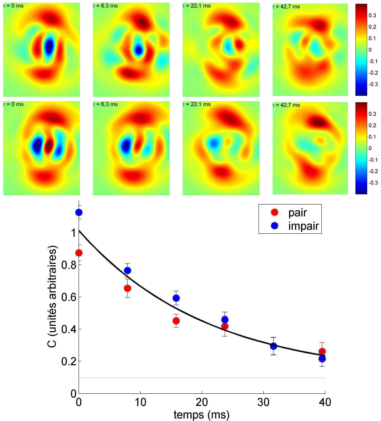
FIG. V.8 – Reconstruction résolue en temps de chats de Schrödinger de séparation D^2 = 10,3 photons. La première ligne représente quatre images successives de la fonction de Wigner du chat impair, la deuxième ligne représente la fonction de Wigner du chat pair aux mêmes instants \tau = 0, 6,3, 22,1 et 42,7 ms. Enfin, les courbes composées des points bleus et rouges montre la cohérence des états pairs et impairs en fonction du temps. La ligne noire est un ajustement exponentiel commun aux deux jeux de données. Le temps de décohérence obtenu est de T_D = 21 \pm 4 ms.
