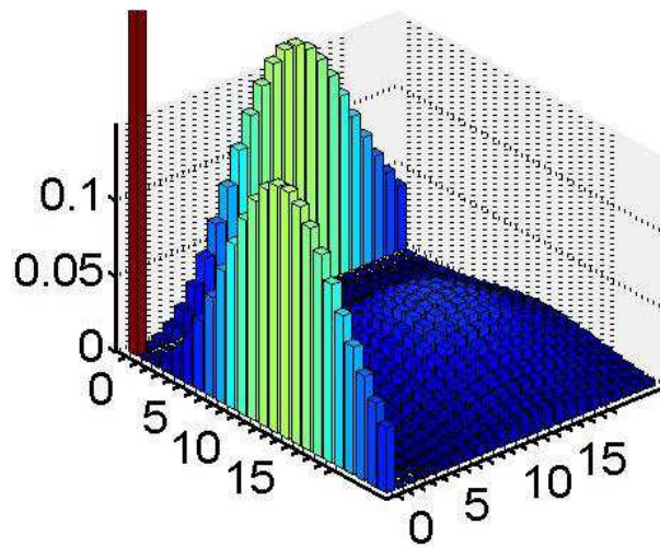
FIG. V.5 – Modules des éléments de la matrice densité \rho(\beta) . On distingue bien quatre « secteurs » où les éléments sont non-nuls, correspondant chacun à un terme de l'expression (V.59).
