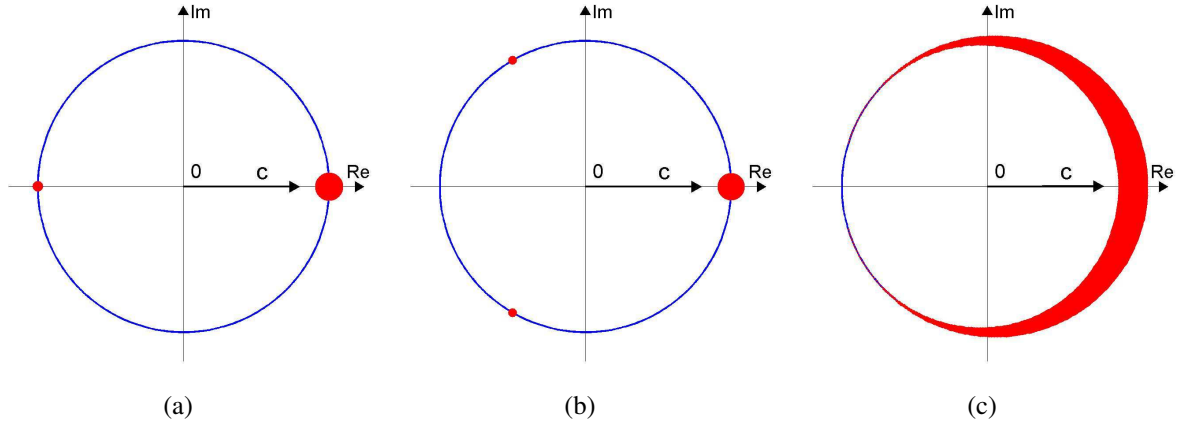
FIG. III.5 – Les points e^{i\phi_k} sont représentés sur le cercle unité par un point rouge de surface proportionnelle à leur poids statistique w_k . La flèche noire représente le contraste c de l'interféromètre ( c = \sum_k w_k e^{i\phi_k} ). Les différentes figures correspondent à un interféromètre dont le contraste fini est dû uniquement aux fausses détections atomiques (a), à un brouillage de phase prenant trois valeurs discrètes \phi_0 = 0 , \phi_1 = 2\pi/3 et \phi_2 = -2\pi/3 (b), ou encore, à un brouillage continu de la phase de détection (c).
