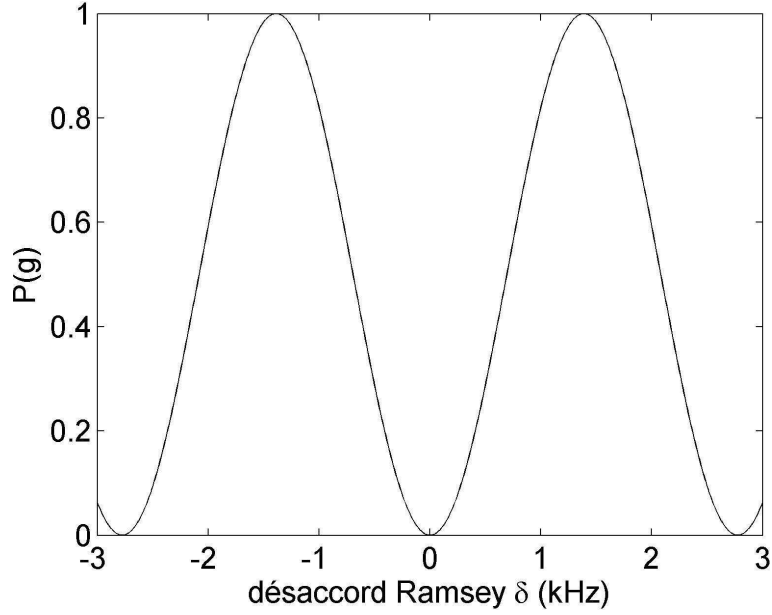
FIG. I.13 – Franges de Ramsey : La probabilité de détecter l'atome dans |g\rangle dépend sinusoidalement de la phase accumulée entre les deux impulsions de Ramsey.
