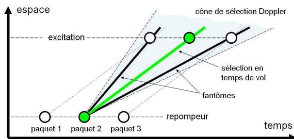
FIG. II.12 – La sélection en temps de vol produit des paquets parasites lorsqu'on tente de préparer des paquets successifs. Ces « fantômes » correspondent aux classes de vitesses sélectionnés par le repompeur du paquet 2 et l'impulsion d'excitation des paquets 1 et 3.
