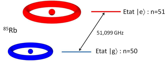
FIG. II.2 – La transition atomique utilisée dans l’expérience relie deux niveaux circulaires successifs, et se situe dans le domaine des micro-ondes à 51,099 GHz
