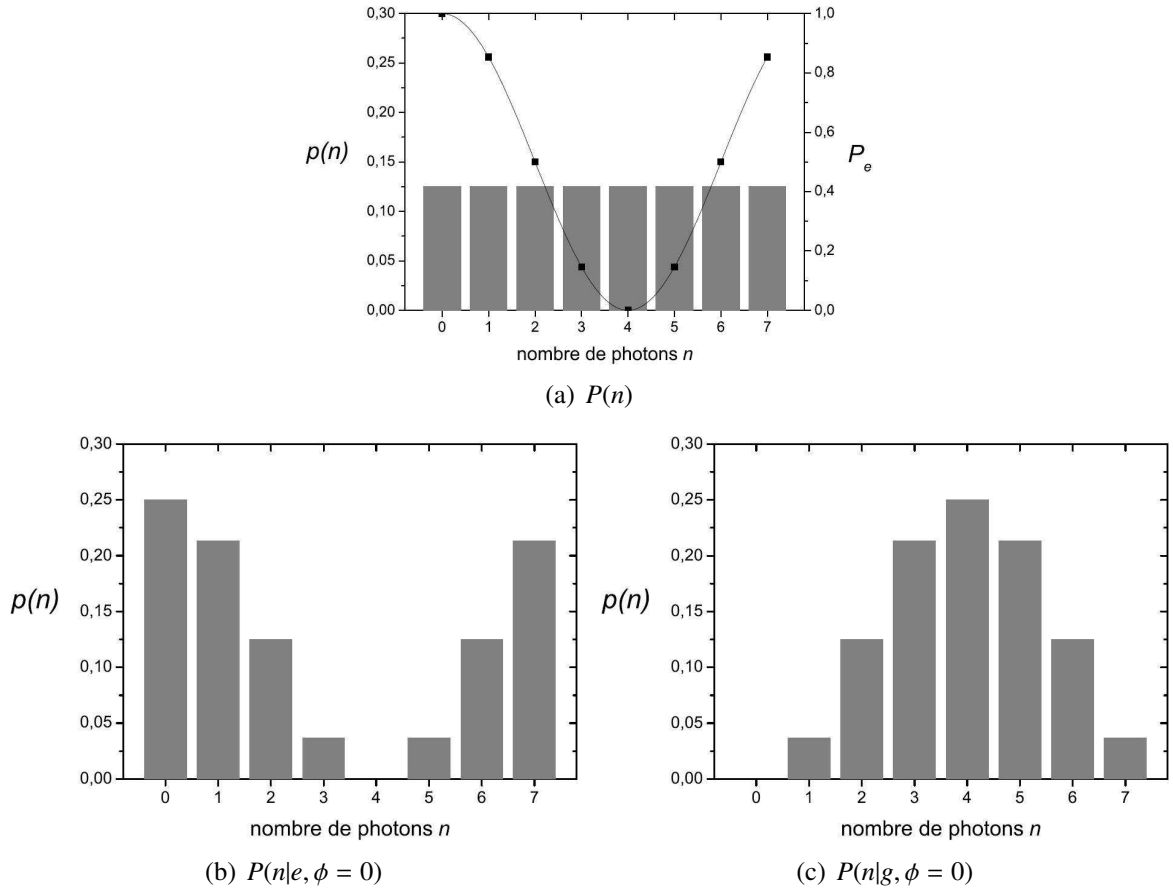
FIG. III.10 – Evolution des populations lors de la détection d'un atome pour un déphasage par photon \Phi_0 = \pi/4 et une phase de mesure \phi = 0 . (a) Probabilités initiales des états de Fock (barres grises, axes de gauche). On prend ici l'exemple d'un champ initial complètement inconnu dont la distribution de probabilités est donc uniforme (de n = 0 à n = 7 ). Les points et la courbe noirs correspondent aux probabilités conditionnelles de détection de l'atome dans l'état |e\rangle (axe de droite). (b) Populations des états de Fock après la mesure si l'atome a été détecté dans |e\rangle . (c) Populations des états de Fock après la mesure si l'atome a été détecté dans |g\rangle .
