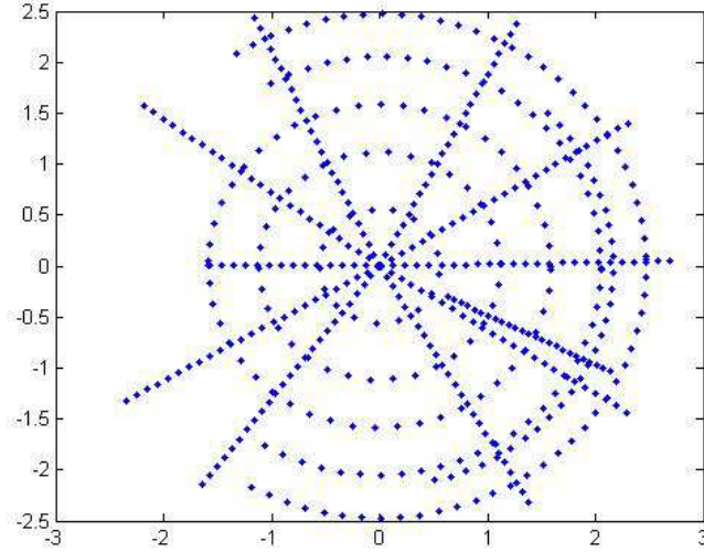
FIG. IV.7 – Les différents point de mesure de la fonction de Wigner généralisée \alpha_v dans le plan complexe.
