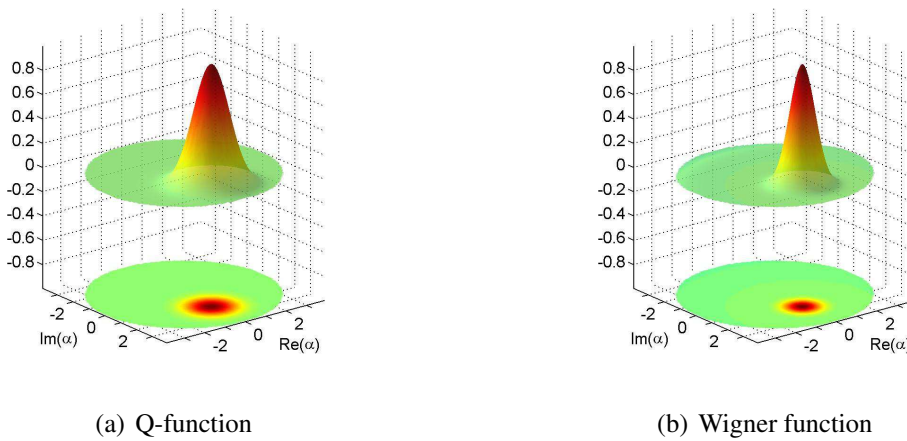
FIG. I.4 – (a) Fonction Q d'un état cohérent |\beta\rangle avec \beta = \sqrt{3} . L'axe vertical est gradué en unité de 1/\pi , (b) fonction de Wigner du même état cohérent (axe vertical en unité de 2/\pi )
