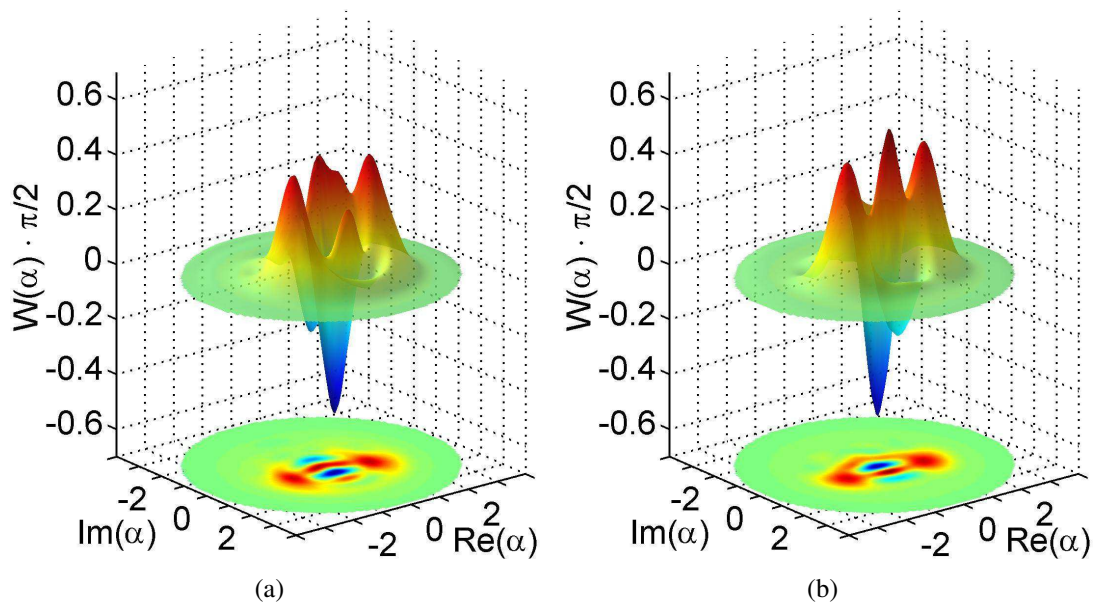
FIG. IV.10 – Les fonctions de Wigner d'états chat de Schrödinger pairs et impairs reconstruits par la méthode d'entropie maximum. Ces états ont été préparés par interaction d'un atome avec un champ cohérent de 2,1 photons en moyenne. Le désaccord est de 65 kHz. La reconstruction a lieu dans un espace de Hilbert de dimension 7.
