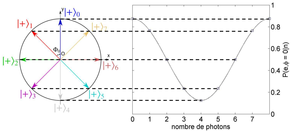
FIG. III.9 – La probabilité de détecter l'atome dans |e\rangle lors d'une mesure avec la phase \phi varie sinusoidalement avec le nombre de photons.
