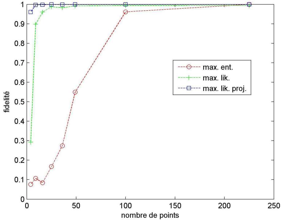
FIG. IV.22 – Evolution de la fidélité de l'état reconstruit en fonction du nombre de points de mesure dans l'espace des phases.
