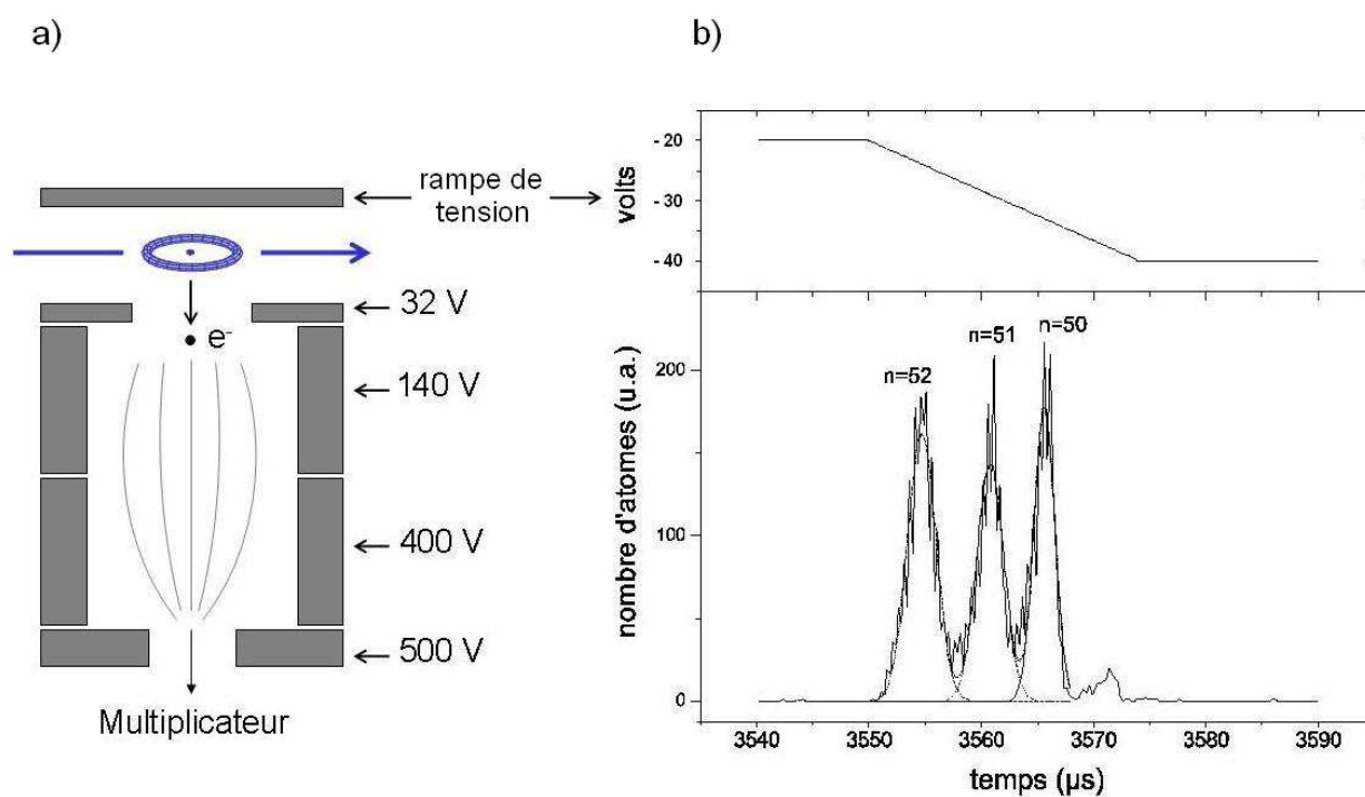
FIG. II.15 – Les atomes de Rydberg sont ionisés dans un champ électrique variable. L'électron est focalisé vers un multiplicateur d'électrons. L'instant auquel l'électron est détecté indique le niveau atomique.
