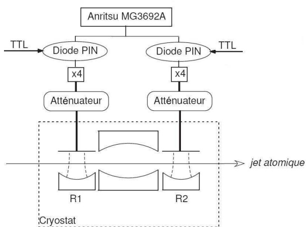
FIG. II.14 – Dispositif d'injection micro-onde dans les zones de Ramsey.
