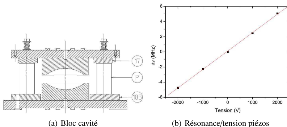
FIG. II.17 – (a) Schéma d'un bloc cavité. 17 et 18B sont les cales en cuivre permettant d'ajuster grossièrement la distance entre les miroirs entre chaque remontage et P est un tube piézoélectrique utilisé pour compenser les petits écarts de fréquences en appliquant une tension à froid.(b) Variation de la fréquence de résonance en fonction de la tension appliquée sur les tubes piézoélectriques.
