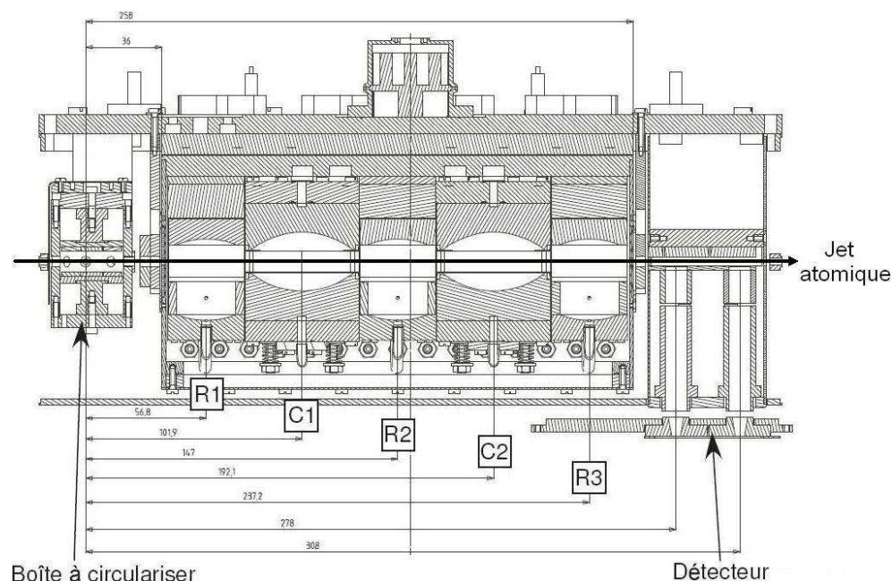
FIG. II.7 – Schéma du cœur du dispositif expérimental. Les pièces vues par les atomes tout le long de leur trajet de la boîte à circulariser jusqu’aux détecteurs sont maintenues à un potentiel bien contrôlé afin de minimiser les inhomogénéités de champ électrique.
