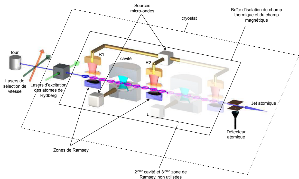
FIG. II.6 – Schéma du dispositif expérimental. Le montage actuel comprend deux cavités de grande finesse en vue de réaliser des expériences sur des champs non-locaux, cependant, la deuxième cavité, montée hors résonance lors du dernier assemblage de l'expérience était inutilisable. Ainsi, les éléments grisés n'ont pas été utilisés dans les expériences décrites dans ce mémoire.
