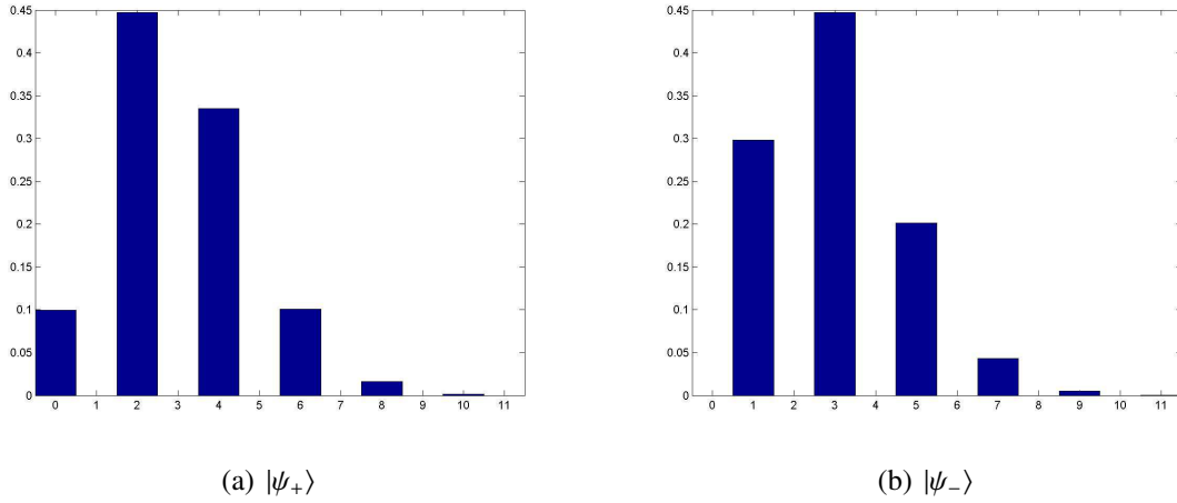
FIG. I.8 – Population des différents états nombres dans les états |\psi_{\text{pair}}\rangle et |\psi_{\text{impair}}\rangle .
