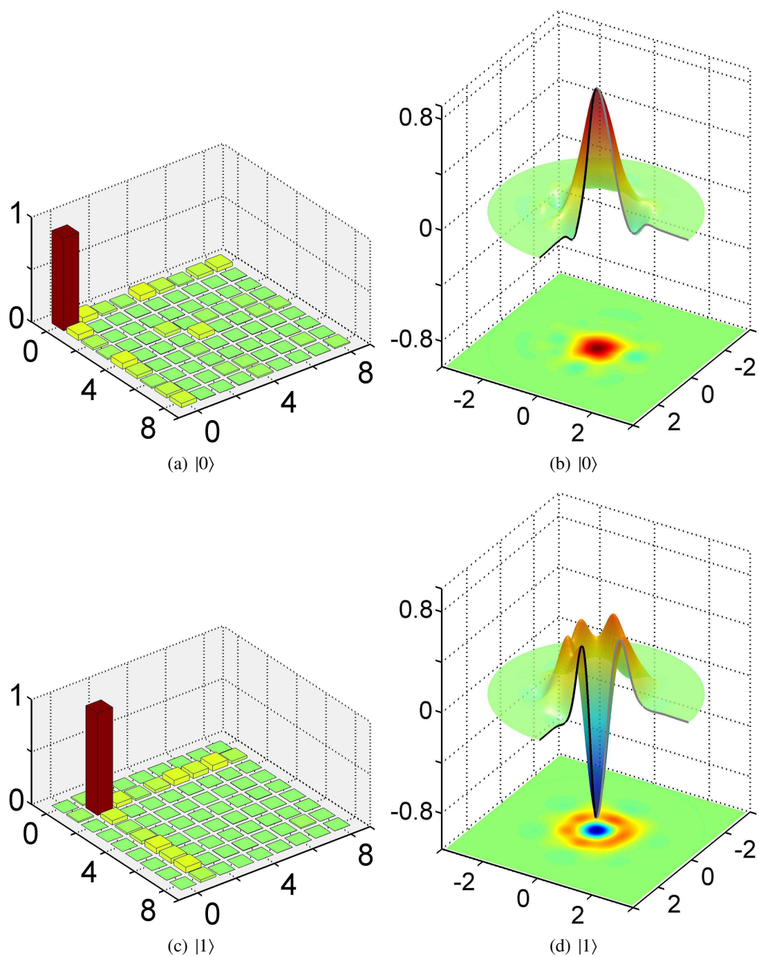
FIG. IV.13 – Modules des éléments des matrices densités reconstruites ((a) et (c)) et fonctions de Wigner correspondantes ((b) et (d)) pour les états de Fock |0\rangle et |1\rangle .
