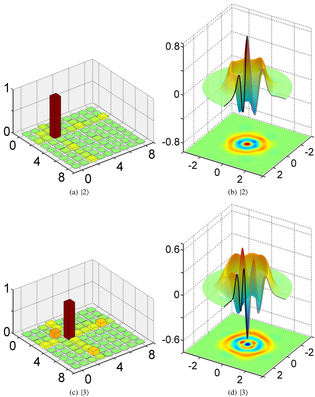
FIG. IV.14 – Modules des éléments des matrices densités reconstruites ((a) et (c)) et fonctions de Wigner correspondantes ((b) et (d)) pour les états de Fock |2\rangle et |3\rangle .
