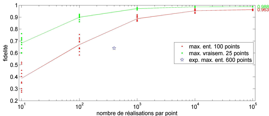
FIG. IV.23 – Evolution de la fidélité en fonction du nombre de réalisations du système utilisées. Les nuages de points correspondent à des reconstructions réalisées à partir de différents jeux de données simulées, afin d'évaluer la variabilité du résultat. Les traits pleins représentent la fidélité moyenne obtenue. Enfin, l'étoile bleue représente la fidélité obtenue lors de notre reconstruction expérimentale par la méthode d'entropie maximum avec une grille de 600 points.
