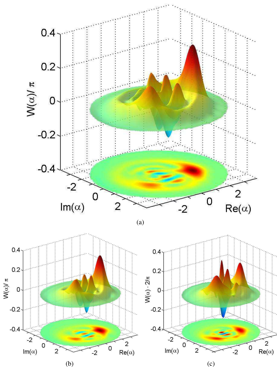
FIG. IV.17 – (a) Fonction de Wigner du chat pair calculée à partir de la matrice densité \rho_{100} . (b) La fonction de Wigner a été obtenue en déplaçant l'état \rho_{100} de l'amplitude -\alpha_{\text{centre}} , en tronquant la matrice obtenue à la dimension 9, en la renormalisant et en la redéplaçant de l'amplitude \alpha_{\text{centre}} . (c) Fonction de wigner du chat impair, obtenue de la même manière.
