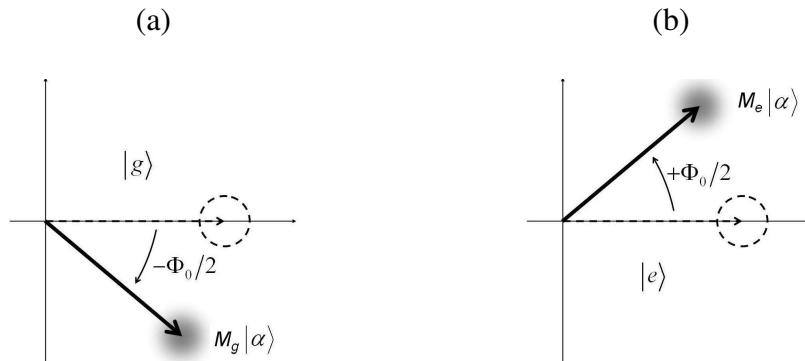
FIG. IV.1 – Évolution du champ dans le plan de Fresnel tournant à la fréquence \omega_0 en présence d'un atome dans (a) |g\rangle ou (b) |e\rangle .
