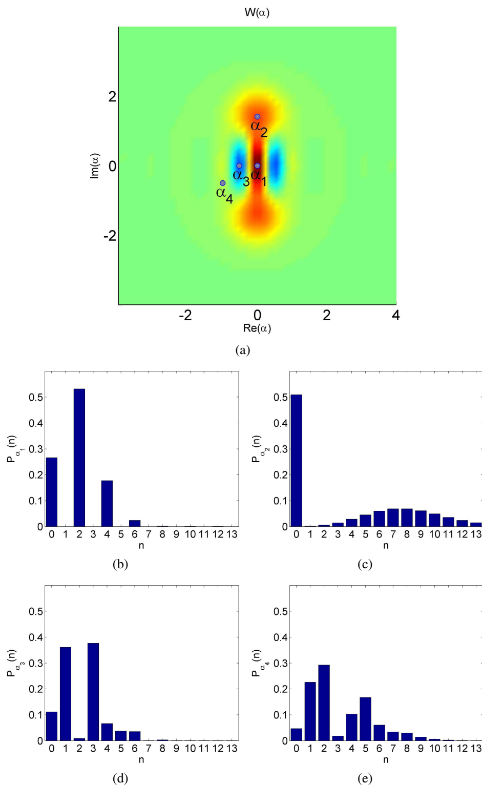
FIG. IV.18 – (a) La fonction de Wigner d'un chat de Schrödinger pair idéal |\Psi_{\text{pair}}\rangle = (|\beta\rangle + |-\beta\rangle)/\mathcal{N}_+ avec \beta = i\sqrt{2} . Les histogrammes (b) à (e) représentent les populations dans les états déplacés de l'amplitude complexe \alpha_\gamma . L'histogramme (b) représente la distribution de population dans l'état non-déplacé ( \alpha_1 = 0 ). Seuls les nombres pairs de photons sont peuplés, ce qui implique que W^{|\Psi_{\text{pair}}\rangle}(0) = 2/\pi . La figure (c) représente la population de l'état déplacé de l'amplitude complexe \alpha_2 = \beta . L'état après déplacement s'écrit donc |\Psi\rangle = (|0\rangle + | -2\beta\rangle)\mathcal{N}_+ . La distribution de population est bien essentiellement la moyenne entre celle de l'état vide et celle d'un champ cohérent centré autour de 2\sqrt{2} (donc autour de \bar{n} = 8 ). Les deux dernières valeurs de \alpha_\gamma sont quelconques
