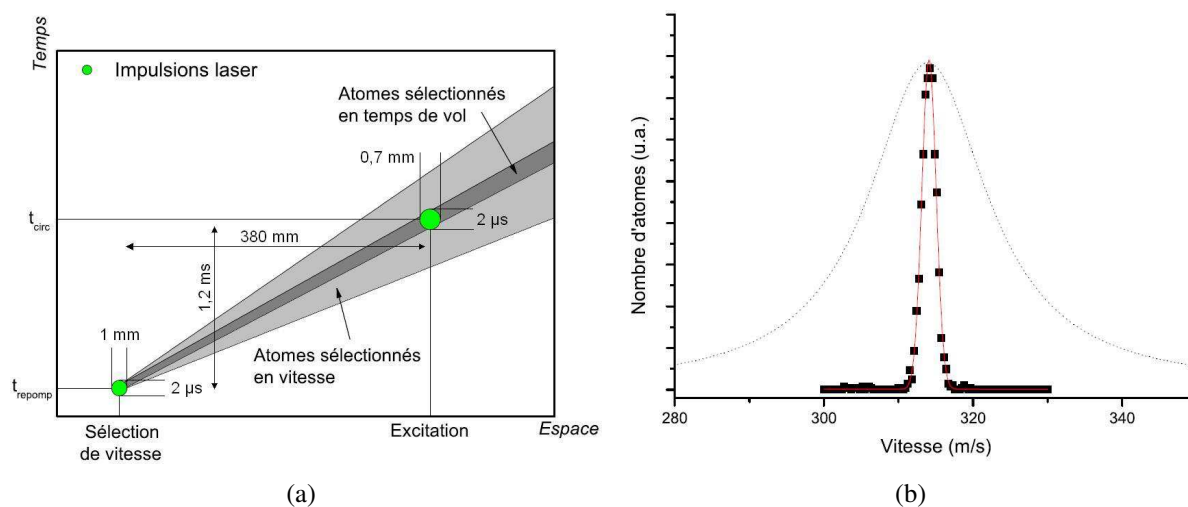
FIG. II.11 – (a) Principe de la sélection par temps de vol : Dans ce diagramme temps-espace, la trajectoire des atomes est une droite dont la pente correspond à la vitesse. Seule une fine classe de vitesse pour laquelle les atomes passent par les points où le repompeur et le laser d'excitation sont allumés est sélectionnée. Les paramètres expérimentaux sont donnés sur la figure. (b) Distribution de vitesse obtenue expérimentalement pour les paramètres décrit sur la figure (a). La classe de vitesse sélectionnée est centrée sur la vitesse de 314 \text{ m/s} . La courbe pleine est un ajustement Gaussien dont la largeur est de 1,9 \text{ m/s} . La courbe pointillée représente à titre de comparaison la distribution de vitesse obtenue par sélection Doppler (Le nombre d'atomes a été renormalisé pour cette courbe).
