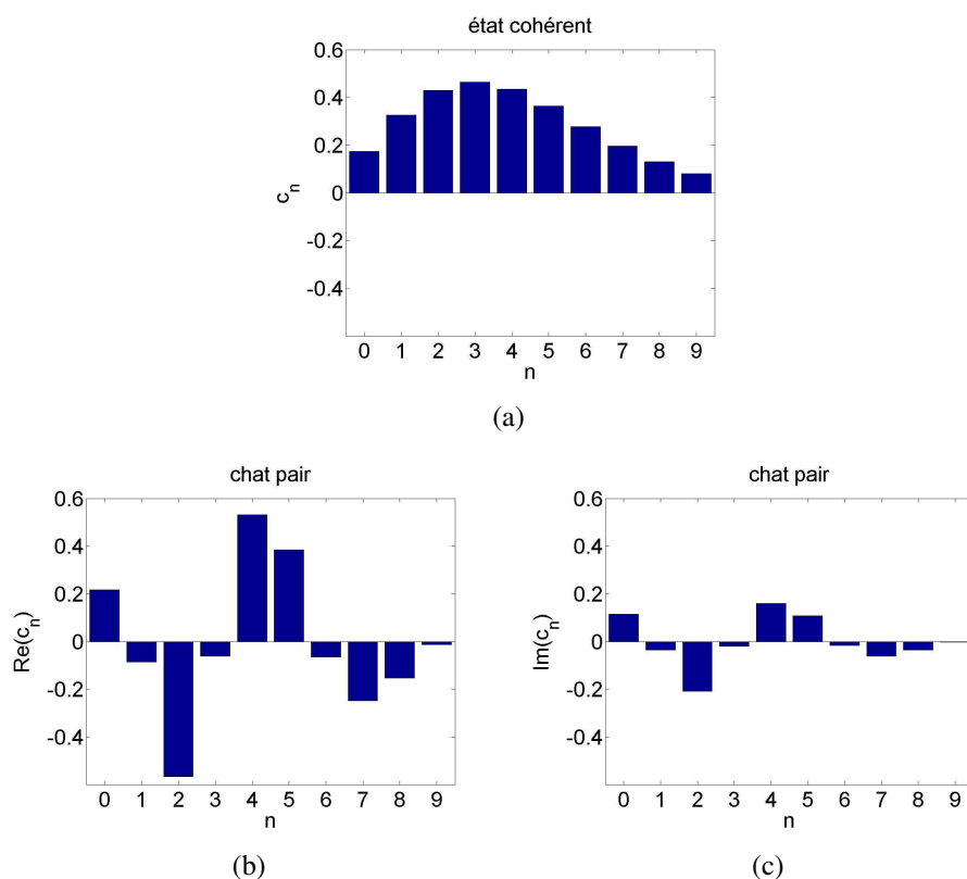
FIG. IV.2 – (a) Coefficients c_n = \langle n|\beta\rangle du champ cohérent avec \beta = \sqrt{3,5} . Parties réelles et imaginaires ((b) et (c)) des coefficients c_n = \langle n|\psi'_+\rangle de l'état chat de Schrödinger pair obtenu par interaction dispersive d'un atome avec un champ cohérent de 3,5 photons. Le désaccord choisi est de 51 kHz.
