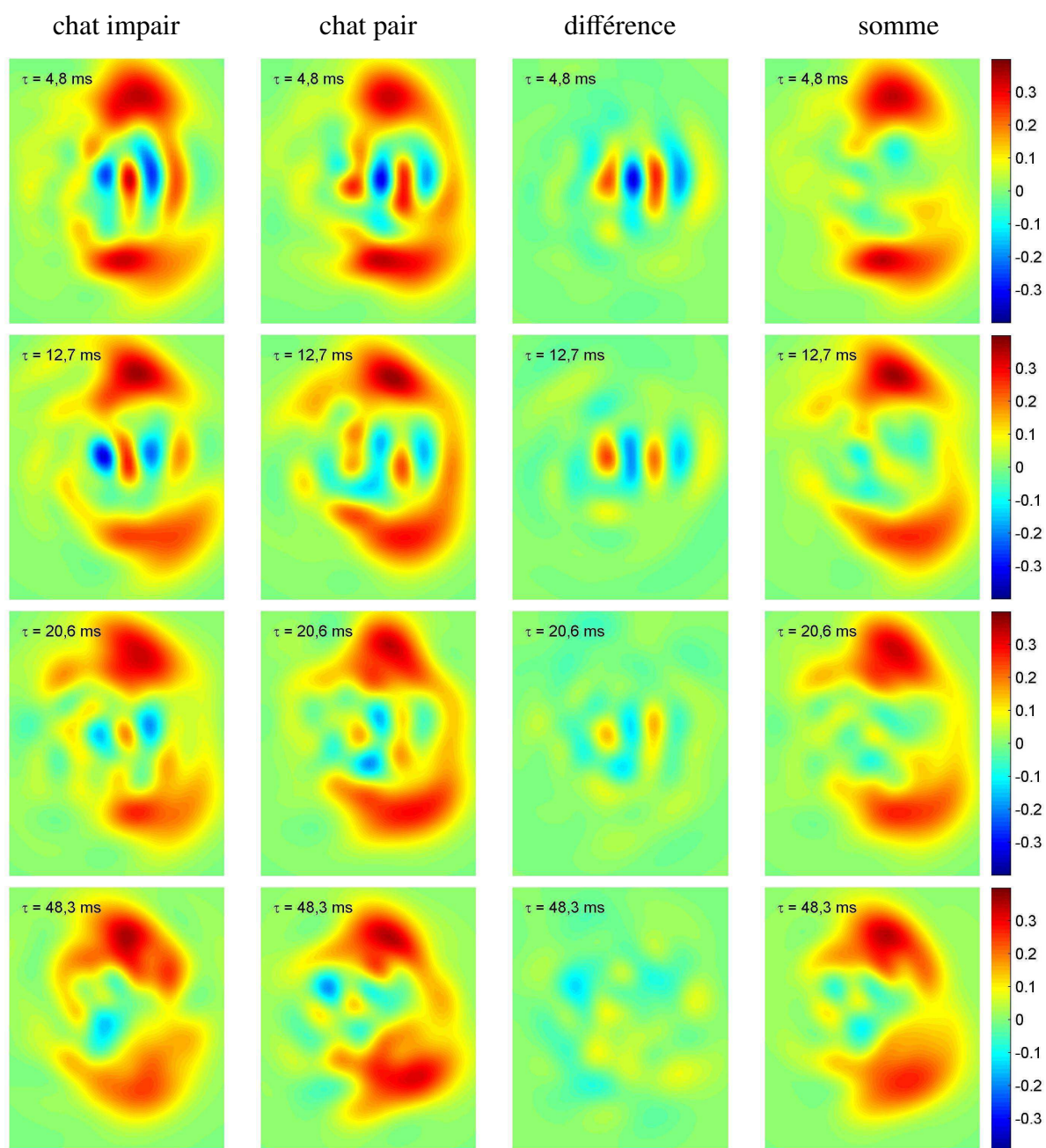
FIG. V.4 – Première et deuxième colonnes : évolution de la fonction de Wigner des chats impair et pair. troisième colonne : différence des fonctions de Wigner du chat pair et impair. Quatrième colonne : somme de ces fonctions.
