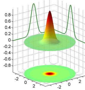
FIG. I.2 – Fonction de Wigner de l'état vide. Les lignes vertes représentent les densités de probabilité des quadratures X et P .
