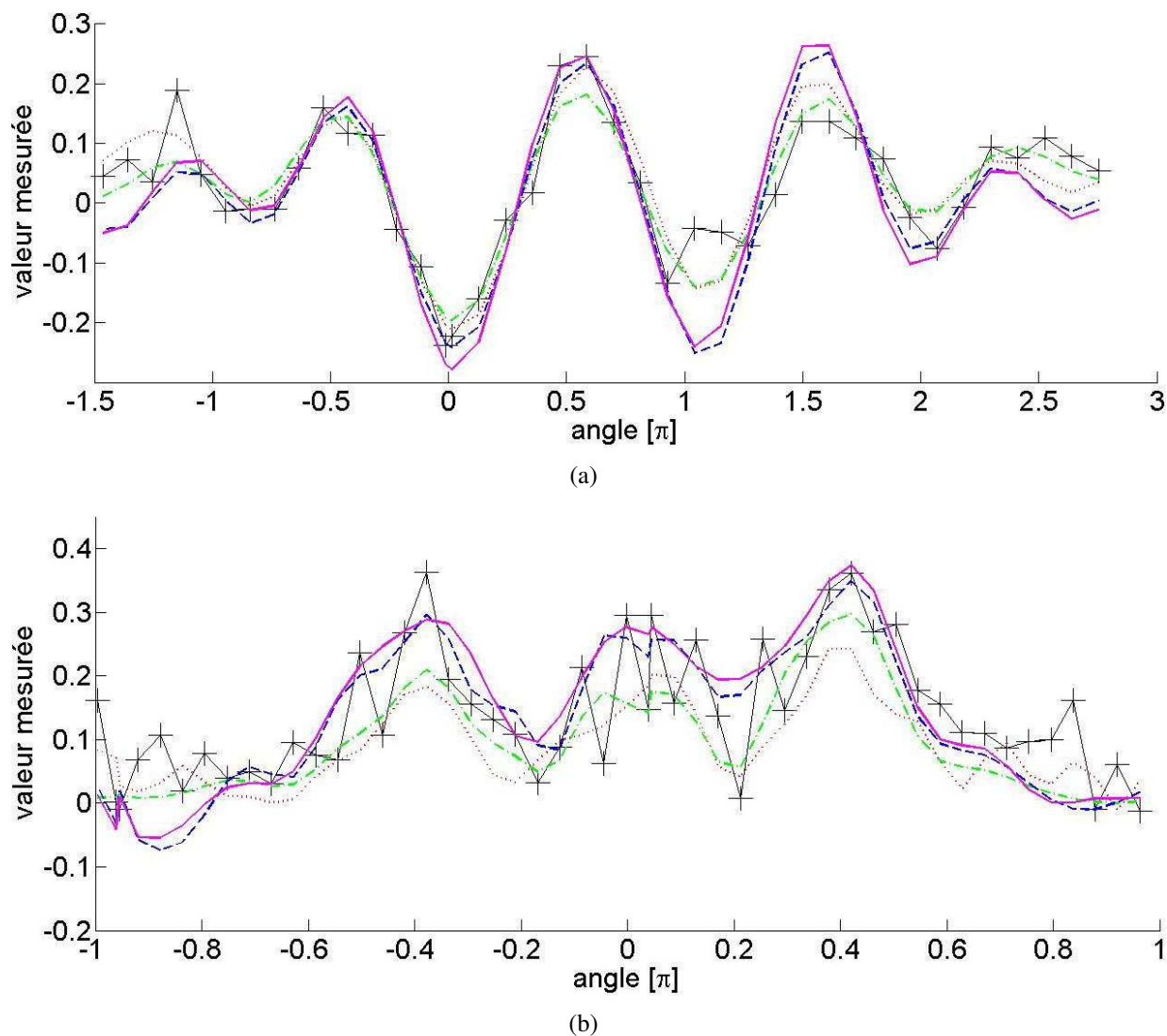
FIG. IV.9 – Les valeurs mesurées pour les points expérimentaux de la figure IV.2.1 dans le cas du chat impair sont représentés par les croix noirs. La ligne en pointillés rouges correspond aux valeurs obtenues dans le cas de la reconstruction directe dans un espace de Hilbert de dimension 20 (voir IV.8(a)). La ligne interrompue verte correspond à la reconstruction dans un espace tronqué de dimension 11 (voir IV.8(b)). Enfin la ligne en tirets bleues représente les points obtenus lorsqu'on pondère l'importance des points expérimentaux suivant la valeur mesurée (voir IV.8(c)).
