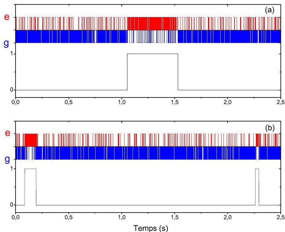
FIG. III.7 – Deux trajectoires quantiques individuelles. Chaque atome détecté est représenté par une barre bleue pour les atomes dans l'état |e\rangle et une barre rouge pour les atomes dans |g\rangle . En dessous de chaque séquence, on a représenté le résultat d'un vote majoritaire à 8 atomes permettant de filtrer les erreurs de détection. (a) Présence exceptionnellement longue d'un photon dans le mode. (b) Trajectoire plus typique.
