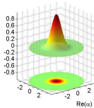
FIG. I.3 – Fonction Q de l'état vide.
