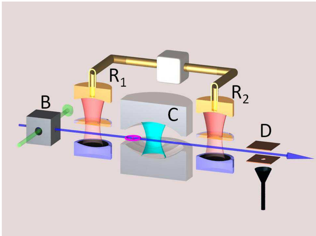
FIG. II.1 – Schéma de principe des expériences d'électrodynamique quantique en cavité avec des atomes de Rydberg circulaires.
