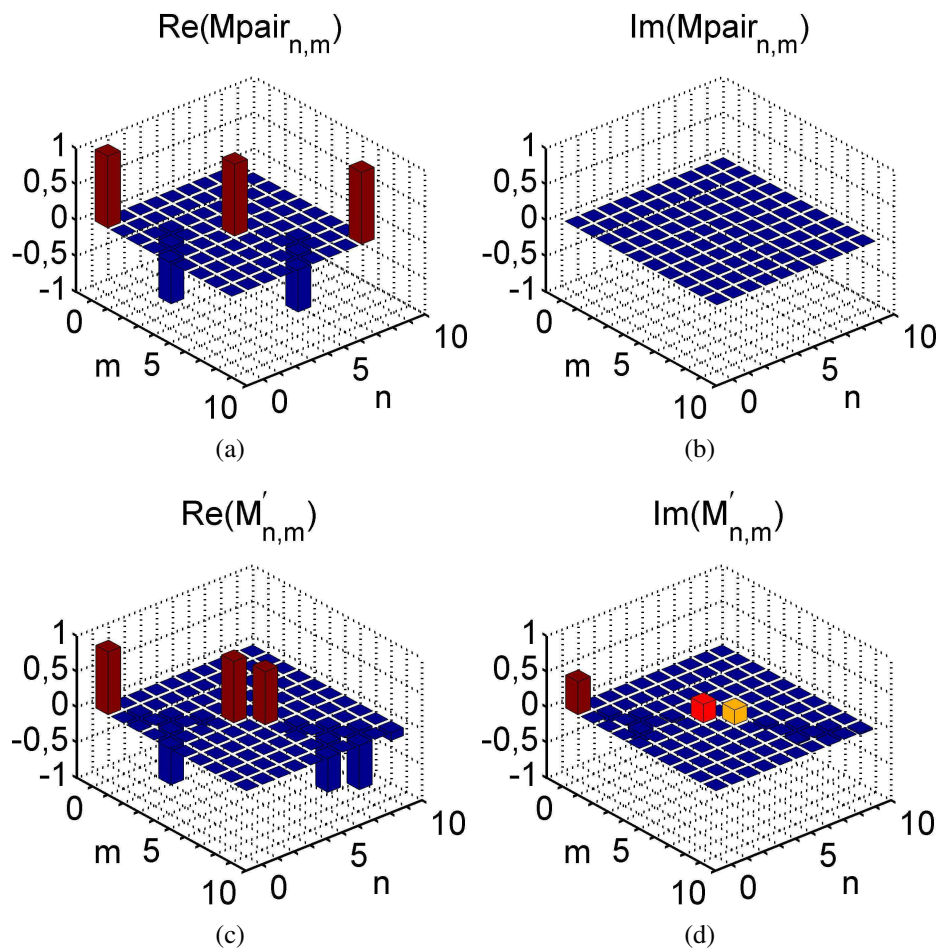
FIG. IV.3 – (a) et (b) : les éléments de l'opérateur de Kraus M_{\text{pair}} correspondant à un déphasage parfaitement linéaire \Phi(n) = \pi(n + 1/2) . (c) et (d) : les éléments de l'opérateur de Kraus M'_+ correspondant à un déphasage non-linéaire calculé pour \delta = 51 kHz.
