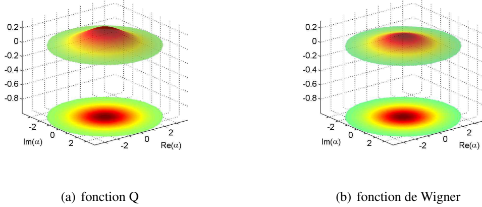
FIG. I.5 – Fonction Q (a) et fonction de Wigner (b) d'un état thermique avec \bar{n} = 3 .
