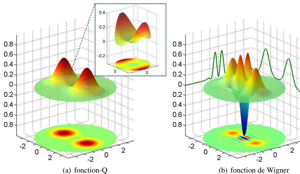
FIG. I.9 – Fonction Q (a) et fonction W (b) de l'état |\psi_{\text{impair}}\rangle = \frac{1}{\mathcal{N}} (|\beta\rangle - |-\beta\rangle) avec \beta = \sqrt{3} . La vignette sur la fonction Q est un agrandissement de la région centrale permettant de distinguer des franges d'oscillations quantiques.
