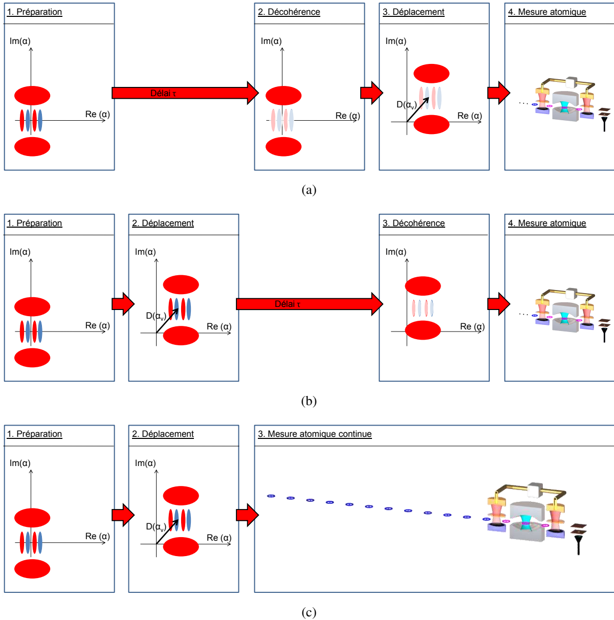
FIG. V.3 – Trois stratégies possibles pour reconstruire l'état \mathcal{L}(\rho, \tau) : (a) Le scénario idéal consiste à préparer l'état \rho , le laisser relaxer pendant un temps \tau , puis mettre en oeuvre la procédure de reconstruction habituelle. (b) Le champ est préparé dans l'état \rho et immédiatement déplacé en un point de mesure \alpha_v . On laisse relaxer l'état déplacé pendant une durée \tau avant de mesurer le signal atomique. (c) Comme précédemment la décohérence a lieu sur l'état déplacé, cependant, la mesure atomique à l'instant \tau est précédée d'une série de « mesures atomiques non-lues ».
