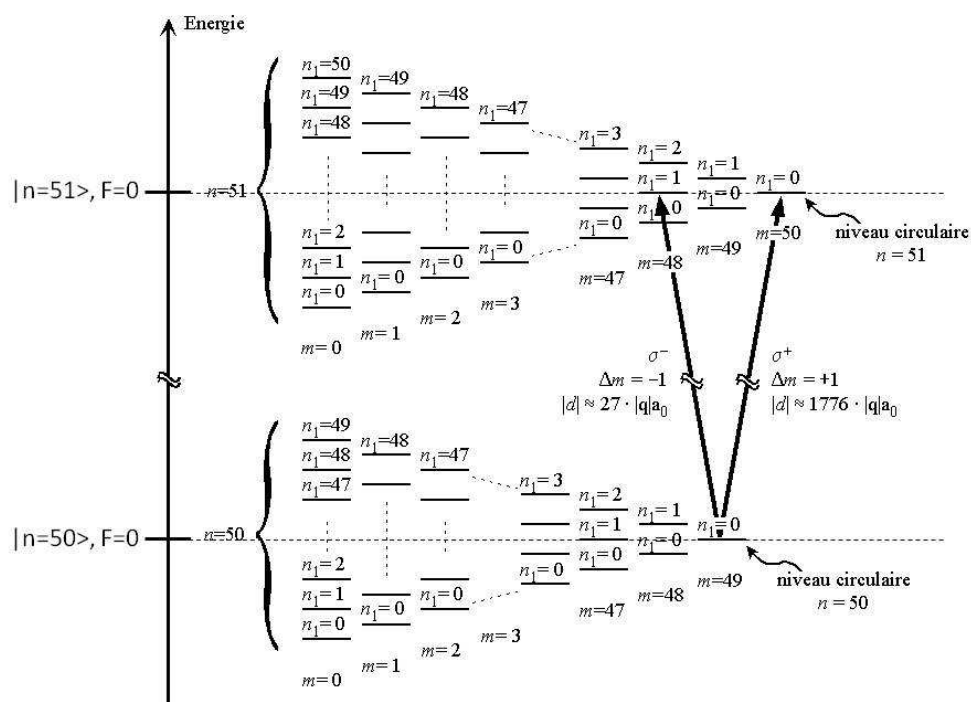
FIG. II.3 – Diagramme d'énergie des niveaux de Rydberg n = 50 et n = 51 en présence d'un champ électrique. Les deux niveaux indiqués sur l'axe vertical correspondent aux énergies des multiplicités n = 50 et n = 51 en champ nul.
