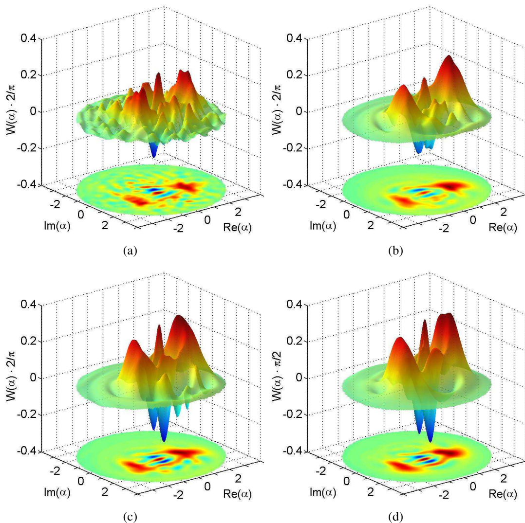
FIG. IV.8 – (a) Fonction de Wigner de l'état chat de Schrödinger pair reconstruit par entropie maximum dans un espace de Hilbert de dimension 20. (b) Le même état reconstruit dans un espace de dimension 11 centré autour de l'amplitude complexe \alpha_{\text{centre}} . (c) A présent, on utilise en plus la loi (IV.31) pour pondérer l'importance des différents points expérimentaux. (d) La dernière étape consiste à tronquer la matrice densité finale en une matrice de dimension 11 (après application du déplacement D(\alpha_{\text{centre}}) ).
