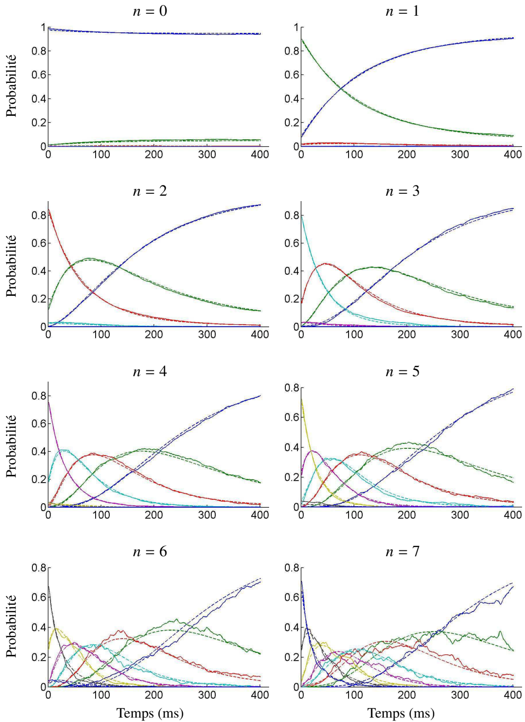
FIG. III.15 – Évolution des populations mesurées P(k, t|n) (traits pleins) et ajustées \mathcal{P}(k, t|n) (tirets). Les valeurs de k allant de 0 à 7 sont respectivement représentées en bleu, vert, rouge, cyan, mauve, jaune, noir et bleu. Les huit séries de courbes correspondent à la sélection des différents états de Fock |n\rangle .
