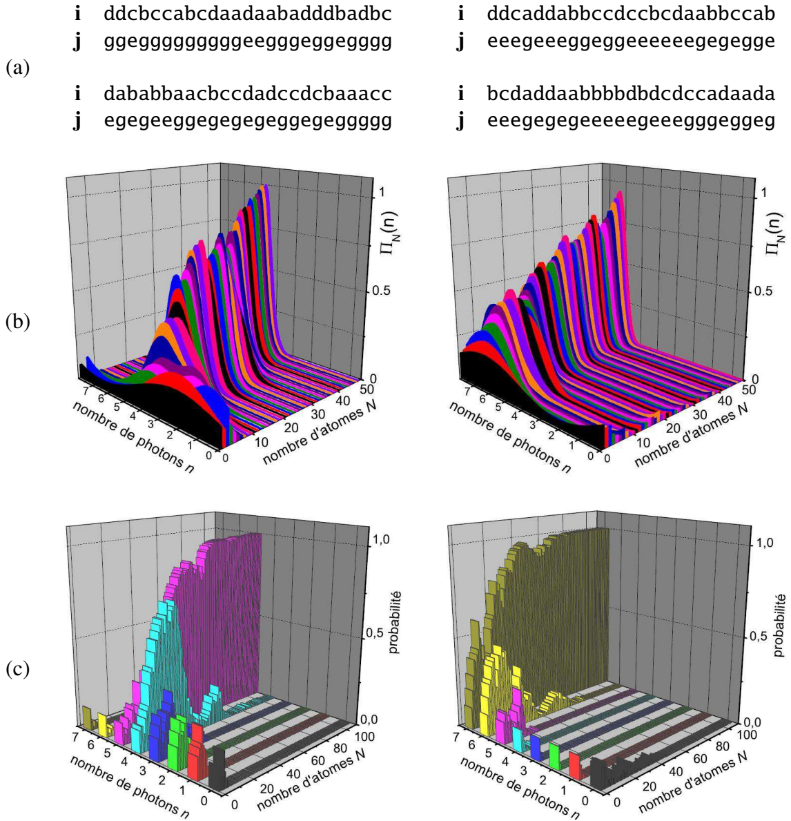
FIG. III.11 – Réduction progressive des probabilités du champ vers un état nombre pour deux réalisations particulières de l'expérience. (a) Résultats des 50 premières détections atomiques ( j, i ) où l'on note j l'état atomique et i la phase de mesure. (b) Evolution de la fonction de détermination \Pi_N(n) en fonction de N au cours des 50 premières détections atomiques. (c) Probabilités des nombres de photons en fonction du nombre N d'atomes détectés variant de 0 à 110.
