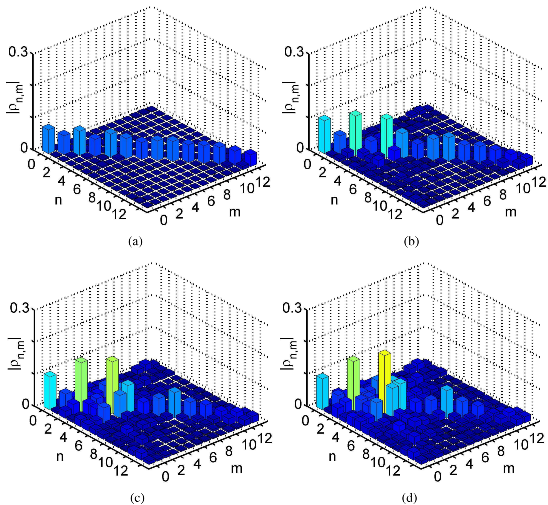
FIG. IV.16 – Modules des 15 premiers éléments de la matrice densité (a) \rho_5 , (b) \rho_{20} , (c) \rho_{50} et (d) \rho_{100} . La matrice densité converge vers le point fixe de la transformation.
