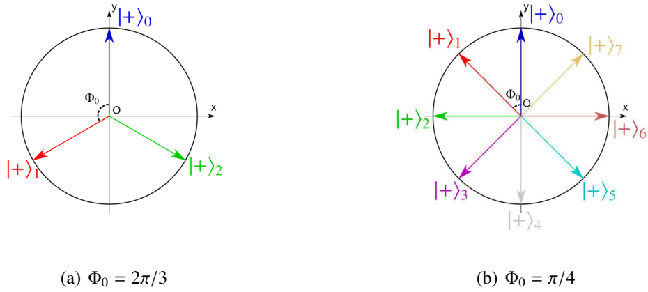
FIG. III.8 – Représentation du pseudo-spin atomique dans le plan équatorial de la sphère de Bloch après interaction dispersive avec un champ contenant n photons. (a) Pour une valeur de \Phi_0 = 2\pi/3 . (b) Pour une valeur de \Phi_0 = \pi/4 .
