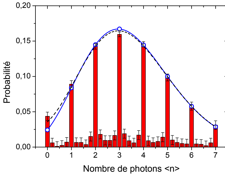
FIG. III.12 – Histogramme des valeurs de \langle n \rangle inférées sur 2000 réalisations et normalisé à 1. Seuls les canaux correspondant à des nombres entiers de photons sont significativement représentés. Ces canaux sont bien ajustés par une distribution poissonnienne (courbe pleine) à l'exception du canal \langle n \rangle = 0 . La prise en compte de notre mesure modulo 8 dans la distribution poissonnienne (tirets) donne un parfait accord pour un nombre moyen de photons de 3,48 \pm 0,04 .
