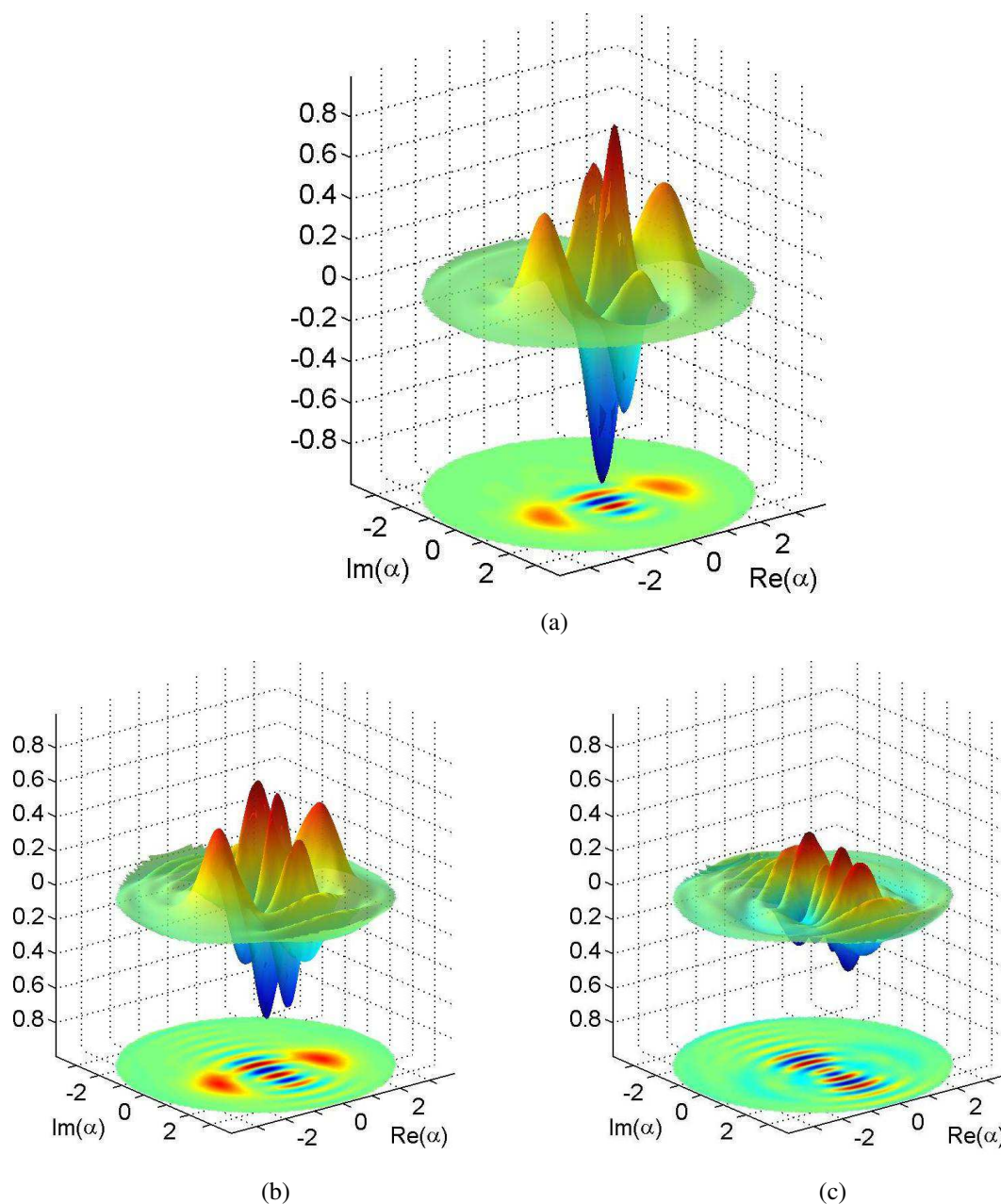
FIG. IV.5 – (a) Fonction de Wigner du chat |\Psi_+\rangle préparé à partir d'un champ cohérent contenant 3,5 photons en moyenne pour un désaccord \delta = 51 kHz, partie réelle (b) et imaginaire (c) de la fonction de Wigner généralisée.
