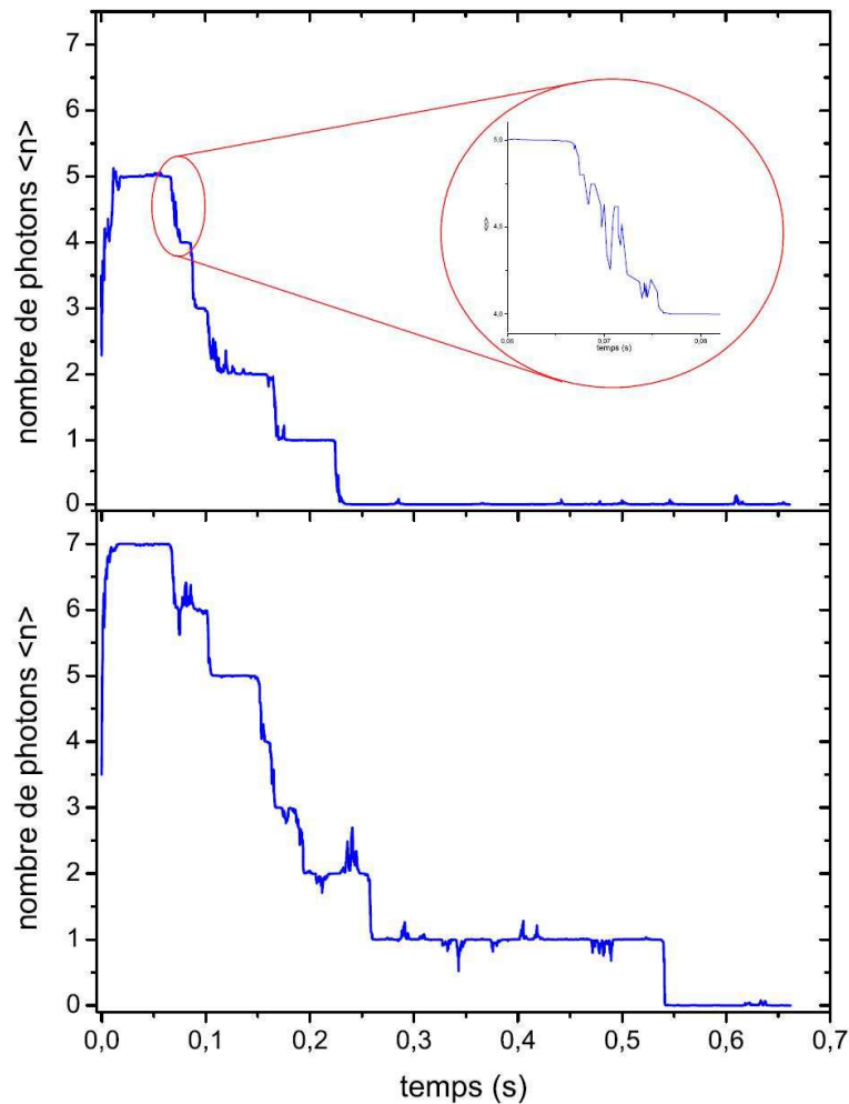
FIG. III.13 – Deux trajectoires quantiques correspondant aux champs dont la mesure initiale est analysée sur la figure III.10. Les deux graphes présentent le nombre de photons moyen \langle n \rangle évalué par une fenêtre de décimation glissante de N = 110 atomes, pendant une durée totale de 0,7 s. L'insert montre un agrandissement de la portion de la première trajectoire entre 0,06 et 0,08 s pendant laquelle le nombre de photons saute de 5 vers 4.
