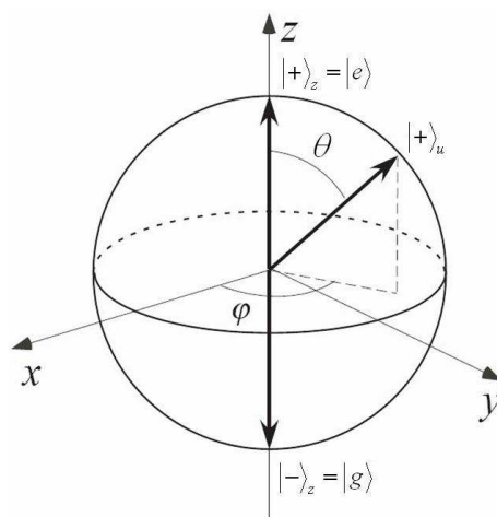
FIG. I.11 – La sphère de Bloch permet de représenter l'état d'un système à deux niveaux
