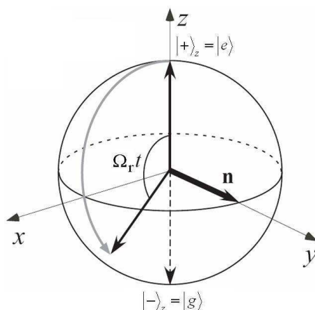
FIG. I.12 – Effet d’une impulsion de micro-onde classique sur le vecteur de Bloch d’un atome initialement préparé dans l’état |e\rangle . Le vecteur unitaire \mathbf{n} autour duquel s’effectue la rotation se trouve dans le plan équatorial. La phase de l’impulsion micro-onde détermine son angle azimutal. Ici, on a choisi \phi = \pi/2 .
