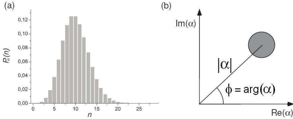
FIG. I.1 – (a) Population des différents nombres de photons dans un état cohérent |\beta\rangle contenant 10 photons en moyenne ( \beta = \sqrt{10} ). (b) représentation du champ cohérent dans l'espace des phases : l'incertitude sur l'amplitude complexe \alpha est représentée par le cercle grisé.
