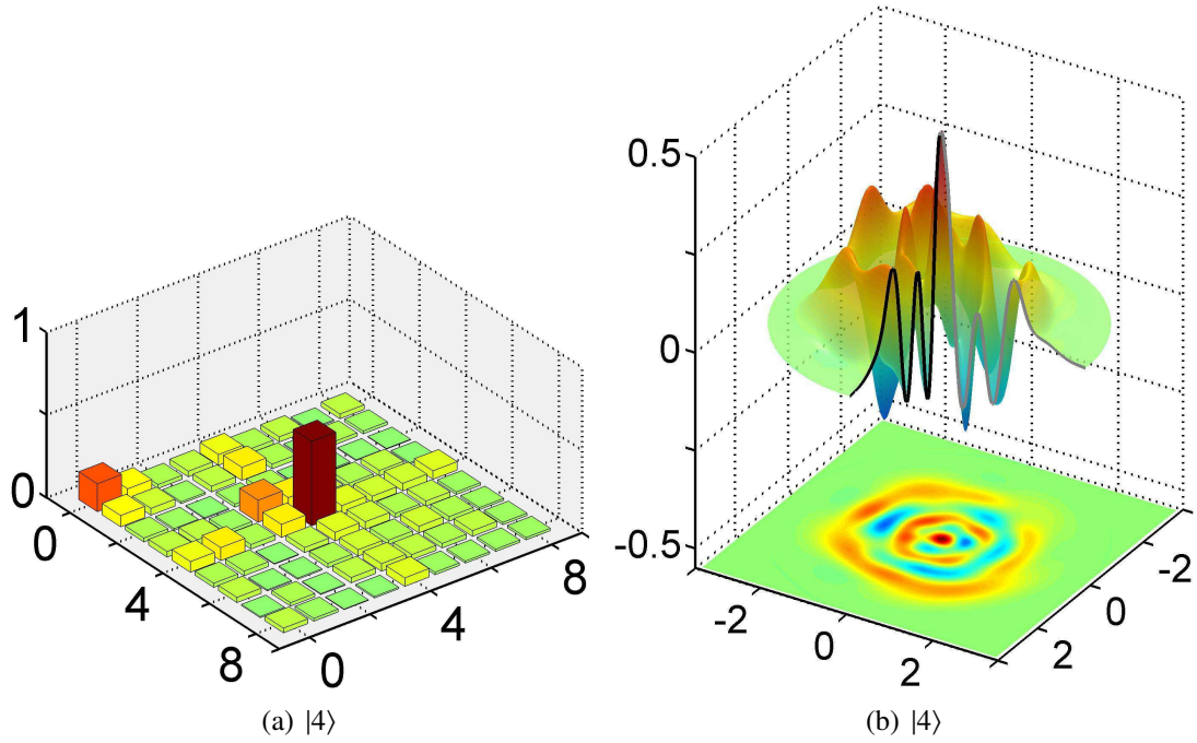
FIG. IV.15 – Modules des éléments de la matrice densité reconstruite (a) et fonction de Wigner correspondante (b) pour l'état de Fock |4\rangle .
