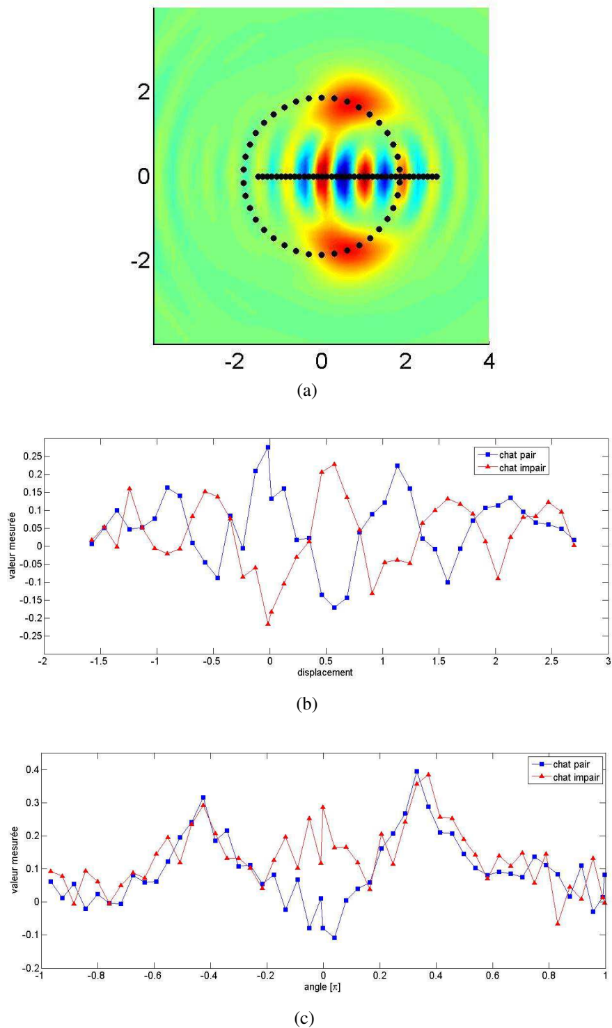
FIG. IV.6 – Deux coupes de la partie réelle de la fonction de Wigner généralisée. La figure (a) montre le résultat attendu théoriquement. Les valeurs mesurées sur la coupe rectiligne et sur la coupe circulaire sont représentées respectivement en (b) et (c) en bleu (carrés) pour le chat pair et en rouge (triangles) pour le chat impair. Les franges d'oscillations sont bien en opposition de phase tandis que les composantes classiques sont identiques. Les fluctuations rapides des signaux mesurés sont dues au bruit statistique.
