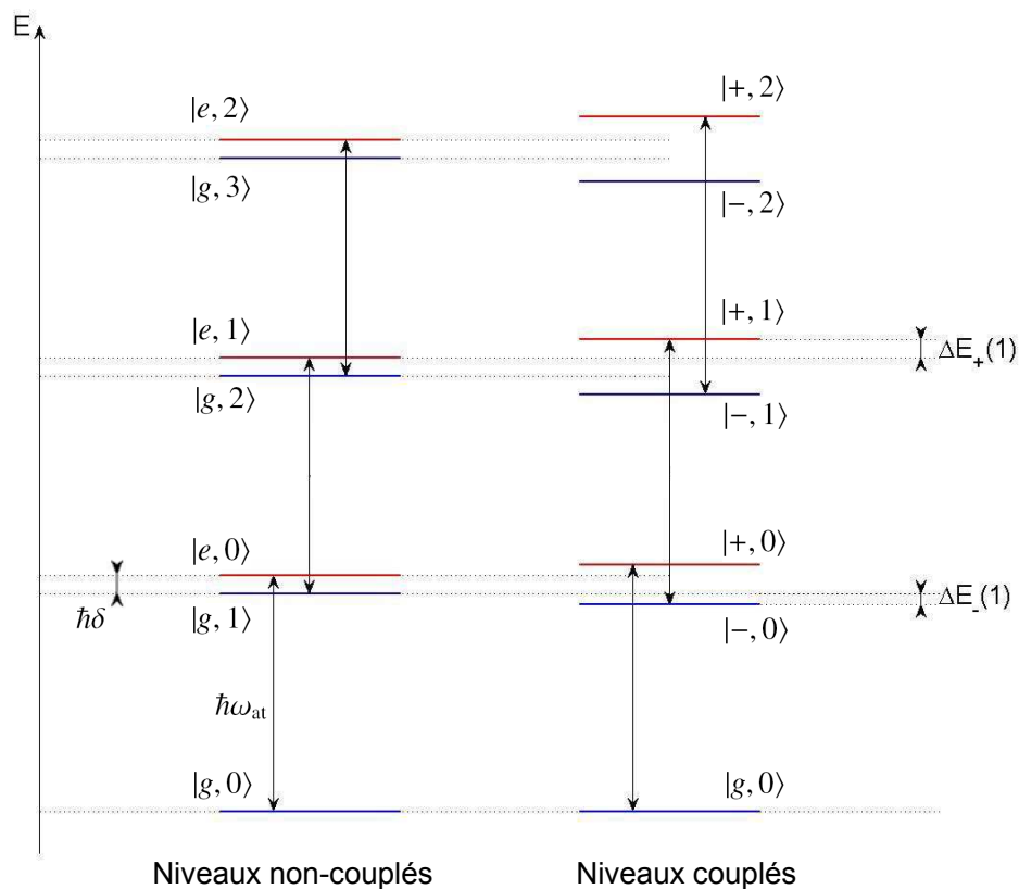
FIG. III.1 – Les énergies propres du Hamiltonien atome-champ dans le cas non-résonant. A gauche : cas d'un couplage nul. A droite, cas d'un couplage fini. Les énergies propres sont déplacées d'une quantité \Delta E_+(n) pour les états |+, n\rangle , et \Delta E_-(n) pour les états |- , n\rangle . La fréquence de la transition entre les niveaux |e, n\rangle et |g, n\rangle est donc déplacée d'une quantité \Delta E(n) = \Delta E_+(n) - \Delta E_-(n) .
