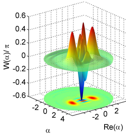
FIG. IV.20 – Fonction de Wigner de l'état à reconstruire.
