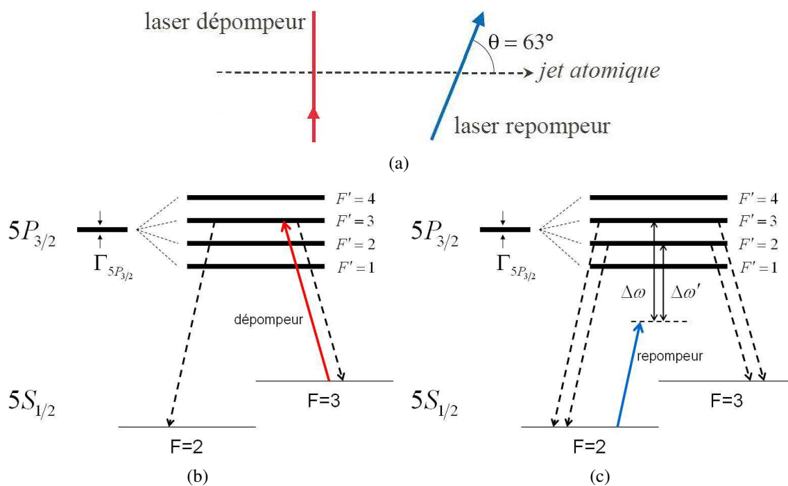
FIG. II.9 – Schéma de principe du dispositif de sélection de vitesse : Le jet atomique rencontre d’abord un laser dépompeur qui pompe tous les atomes dans le sous-niveau F = 2 , puis un Laser repompeur formant un angle de 63^\circ avec ce dernier. Seuls les atomes ayant la vitesse désirée sont repompés dans le sous-niveau F = 3 .
