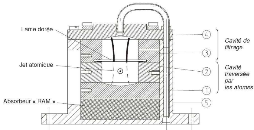
FIG. II.13 – Schéma d'une zone de Ramsey. Le champ micro-onde est d'abord mis en forme spatialement dans une cavité de filtrage. Une partie du champ est transmise à travers la lame dorée dans une cavité de faible Q avant d'être absorbée par le bloc de RAM.
