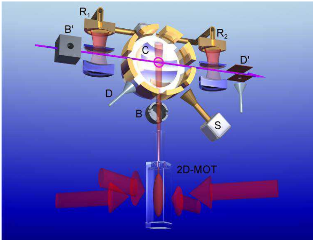
FIG. V.10 – Schéma de principe du futur montage expérimental. En plus des possibilités du montage actuel, un jet atomique vertical permettra de faire interagir des atomes lents avec la cavité.
