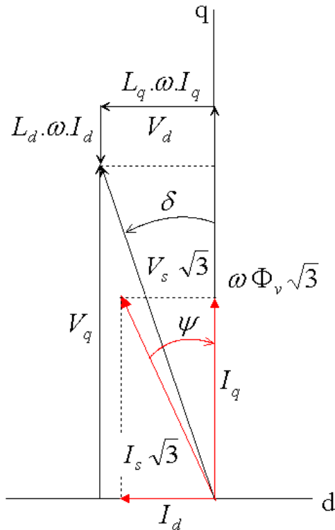
Figure 1.9: Diagramme de Fresnel du modèle sans pertes
