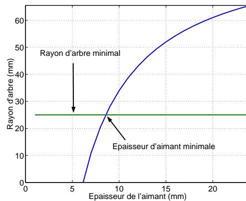
Figure 2.14: Epaisseur des aimants minimale
