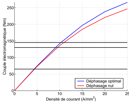
a. Couple en fonction de la densité de courant
