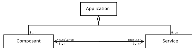
FIG. 3.14 – Représentation UML d'une application
