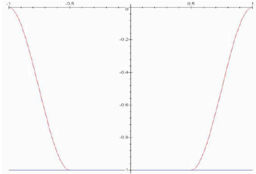
FIG. 4.3 – flexion d’une poutre encastree : contact suivant un intervalle
