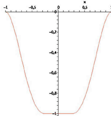
FIG. 4.7 – plaque circulaire encastrée sous un chargement uniforme au dessus d’un obstacle \psi : r \mapsto -1 : la zone de contact \mathcal{I}(F_{24}) = \{(0, 0)\} est un point alors que la réaction est nulle ; puis en augmentant le chargement la zone de contact devient un disque et la réaction est non-nulle.
