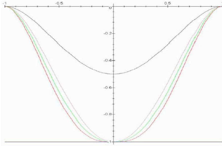
FIG. 4.2 – flexion d'une poutre encastree (par ordre décroissant) : sans contact, contact affleurant, contact tangent avec réaction ponctuelle, contact avec étalement imminent et réaction ponctuelle
