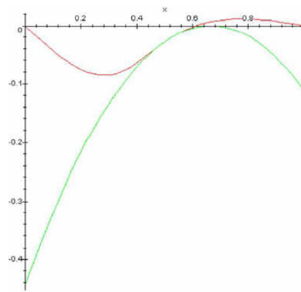
FIG. 4.1 – Graphes de la solution de la poutre en flexion soumise à une force ponctuelle variable
