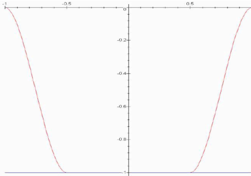
FIG. 4.3 – flexion d’une poutre encastree : contact suivant un intervalle
