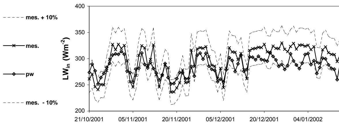
Figure 2.6. Moyennes quotidiennes des rayonnements grandes longueurs d'ondes incidents LW_{in} mesurés ( mes. ) et estimés par la méthode pw ( pw ), et enveloppes LW_{in+10} ( mes. + 10\% ) et LW_{in-10} ( mes. - 10\% ) d'incertitude de la mesure, au cours de la première période de bon fonctionnement du pyrgéomètre (87 jours)
