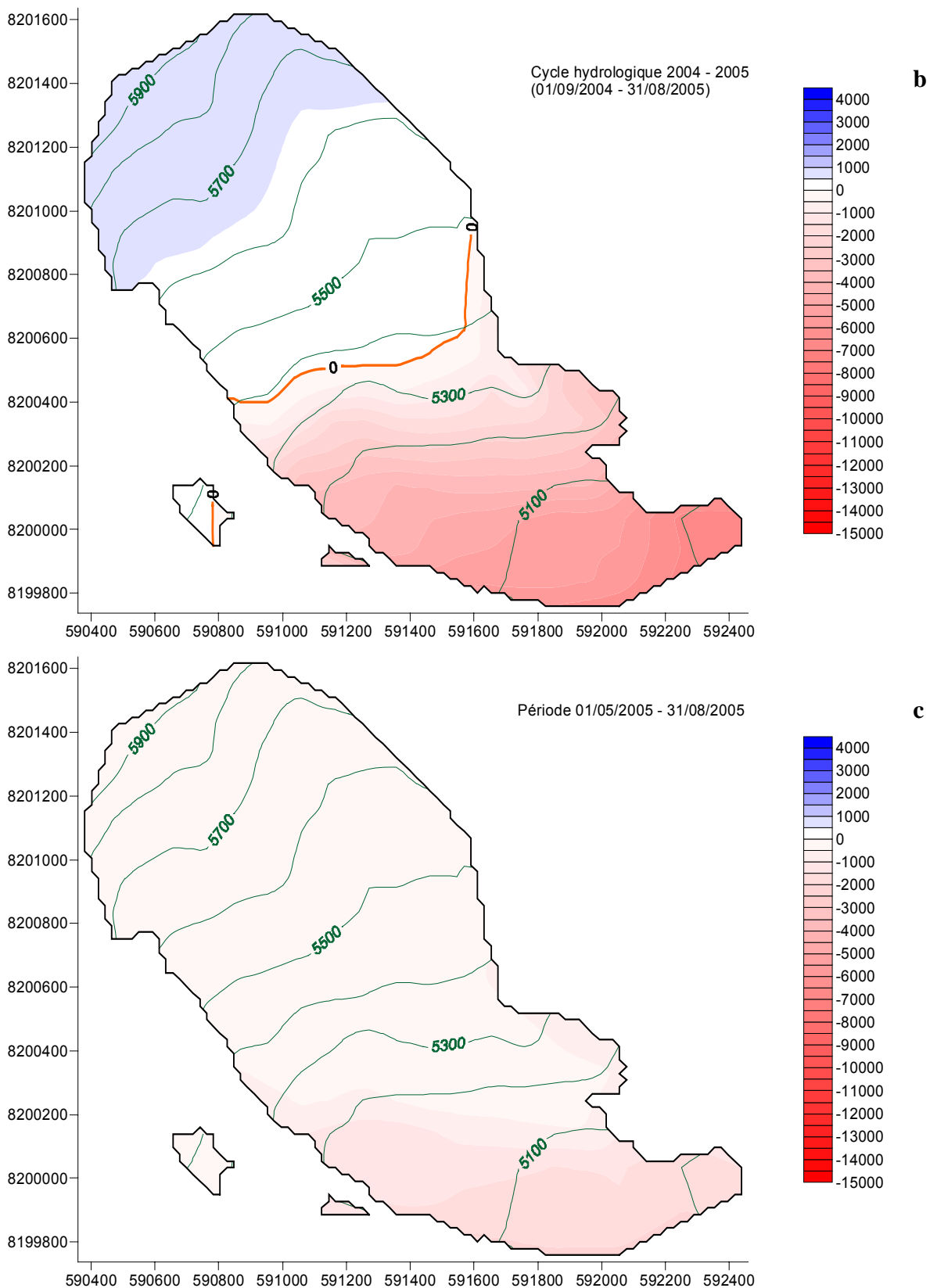
Figures 5.3.b et 5.3.c. Variation spatiale sur la grille RT100WGS du bilan de masse ( mm_{eq.eau} ) du glacier Zongo simulé par le modèle CROCUS (b) pour le cycle hydrologique 2004-2005 (1 er septembre 2004 – 31 août 2005) et (c) la saison sèche de ce cycle (1 er mai 2005 – 31 août 2005).
