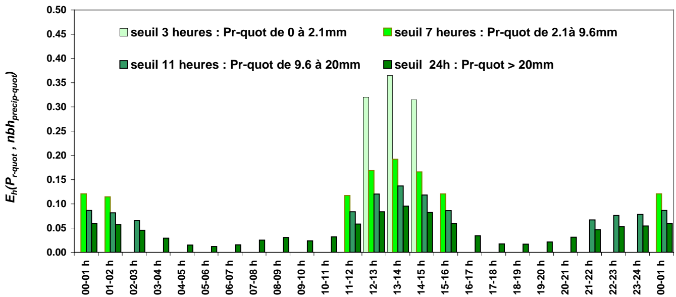
Figure 2.15. Heures et coefficient de répartition E_h(P_{r\text{-quot}}, nbh_{precip\text{-quot}}) des lames d'eau quotidiennes de précipitations P_{r\text{-quot}} en fonction de leurs montants
