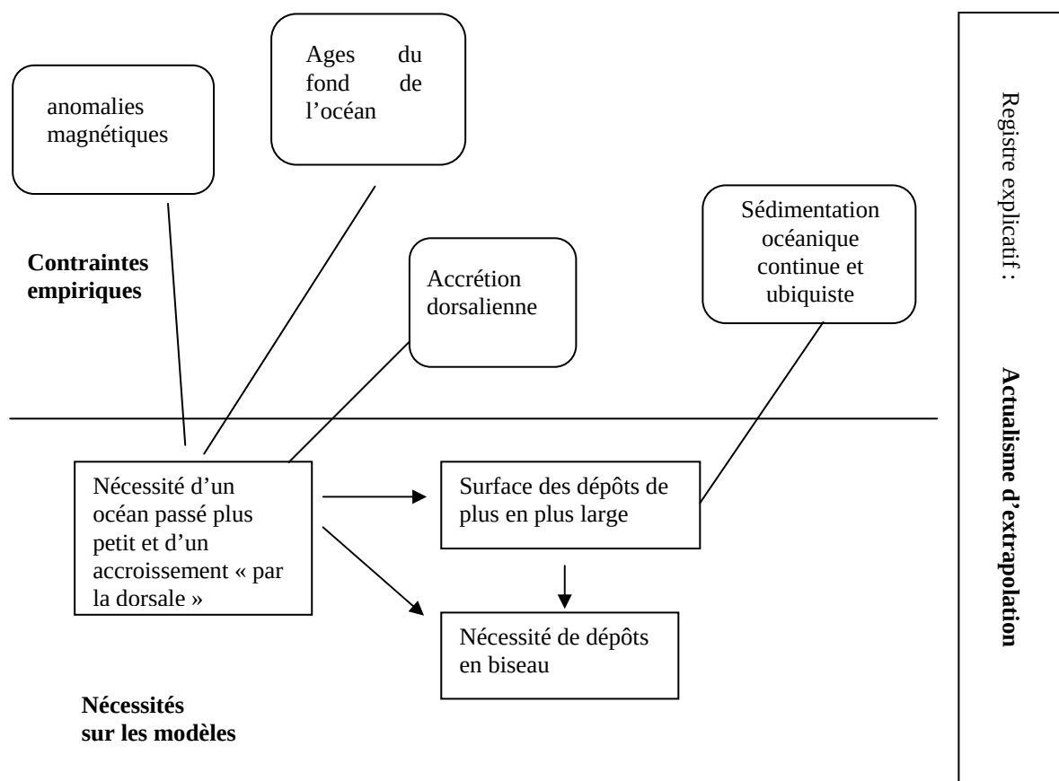
Figure 6.5 : L'espace des contraintes en jeu dans la reconstitution du passé d'un fond océanique
