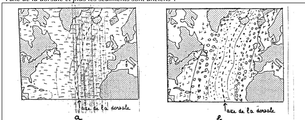
Figure 7.13 : Sédimentation océanique (de dessus) : deux types de réponse
