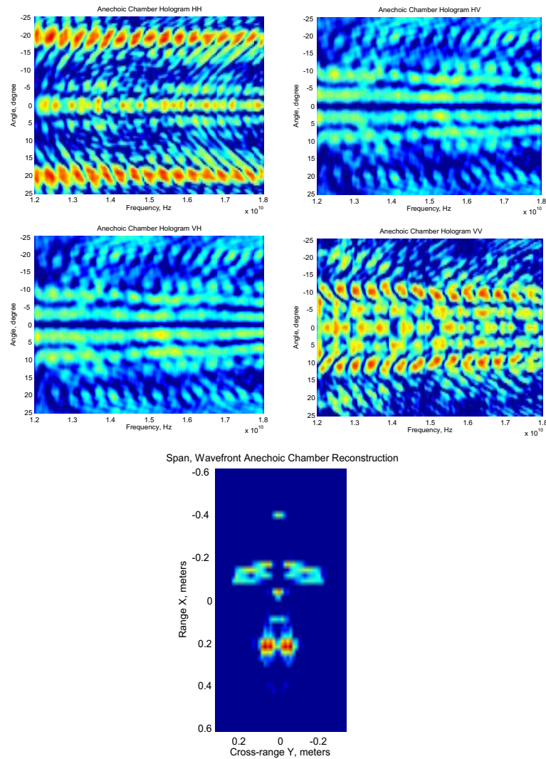
FIG. 5.4 – Données de chambre anechoïque et image du missile "Cyrano".
