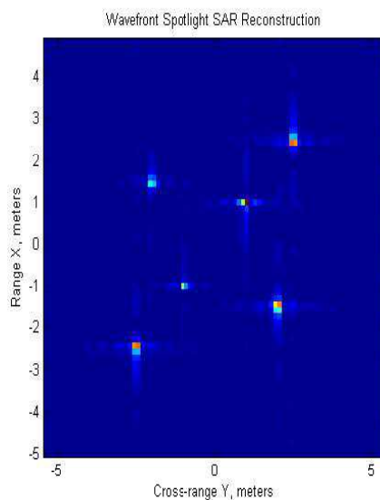
FIG. 1.14 – Résultat de la simulation de l'algorithme RMA.
