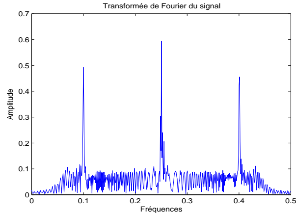
FIG. 2.2 – Spectre du signal non-stationnaire.
