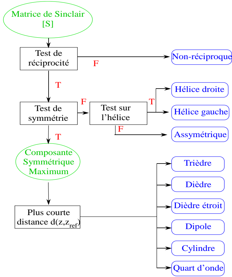
FIG. 3.5 – Technique de classification basée sur la décomposition de Cameron
