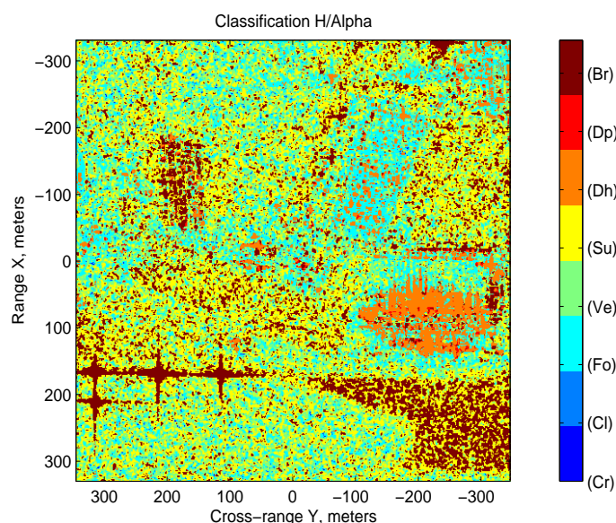
FIG. 3.18 – Résultat de la classification selon les paramètres H/alpha de l'image SAR de la région de Brétigny.
