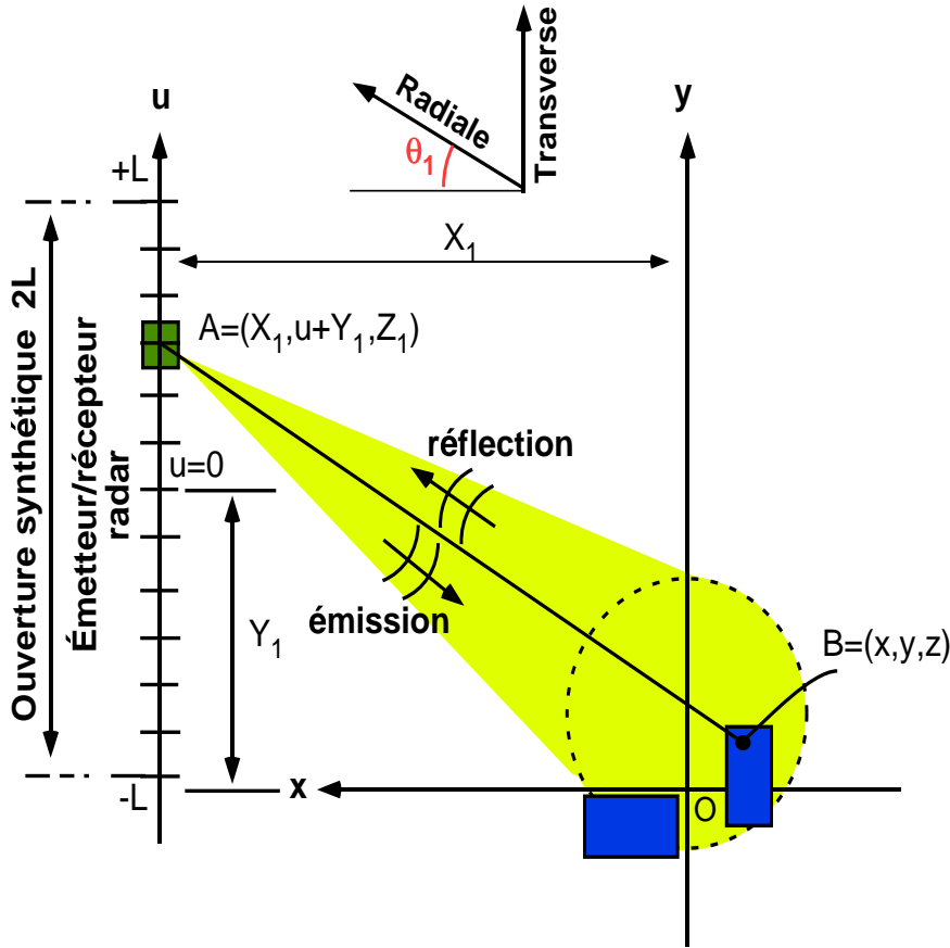
FIG. 1.9 – Géométrie du modèle de mesure en azimuth.
