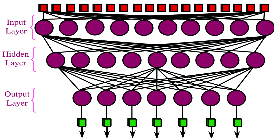
FIG. A.4 – Structure du multi-layer perceptron à trois couches.
