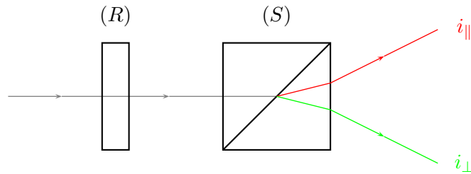
FIGURE 2.6 – Principe de base du polarimètre. Le séparateur ( S ) (prisme de Wollaston) génère deux faisceaux d'états de polarisation orthogonaux d'intensités i_{\parallel} et i_{\perp} . Le réglage des angles entre l'axe de la lame à retard ( R ) (lame quart d'onde) par rapport à l'axe de ( S ) d'une part, et de l'axe de l'ensemble ( R ) + ( S ) par rapport à l'axe Nord–Sud d'autre part, permet de sélectionner le paramètre de Stokes mesuré. Stokes V est mesuré en positionnant les axes lent et rapide de la lame quart d'onde à \pm 45^\circ par rapport aux axes du séparateur de faisceaux. Q et U sont obtenus en alignant les axes de la lame quart d'onde avec ceux du séparateur.
