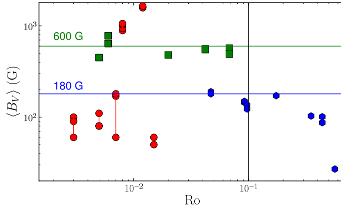
(a) Flux magnétique mesuré à partir de Stokes V
