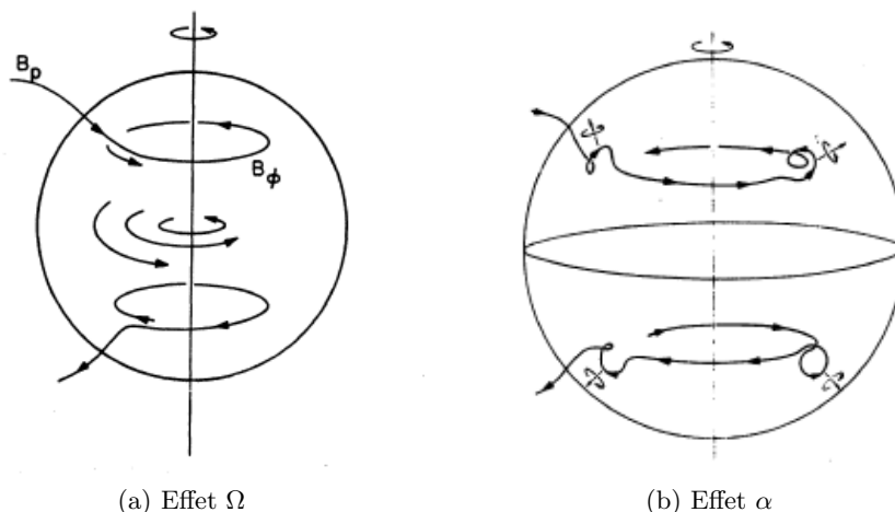
FIGURE 1.5 – Schéma de la dynamo \alpha\Omega . (a) Un champ initialement poloidal est soumis au cisaillement dû à la rotation différentielle, générant un champ toroïdal. (b) La convection rendue hélicitaire par la force de Coriolis régénère un champ poloidal à partir de la composante toroïdale. D’après Parker (1970) .
