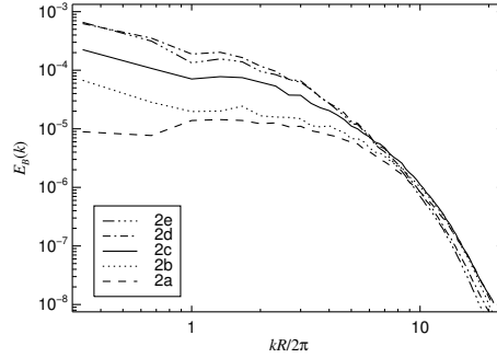
FIGURE 4.2 – Dobler et al. (2006) : évolution du spectre d'énergie magnétique dans la phase saturée en fonction du taux de rotation. La numérotation des simulations fait référence à la table 4.3.
