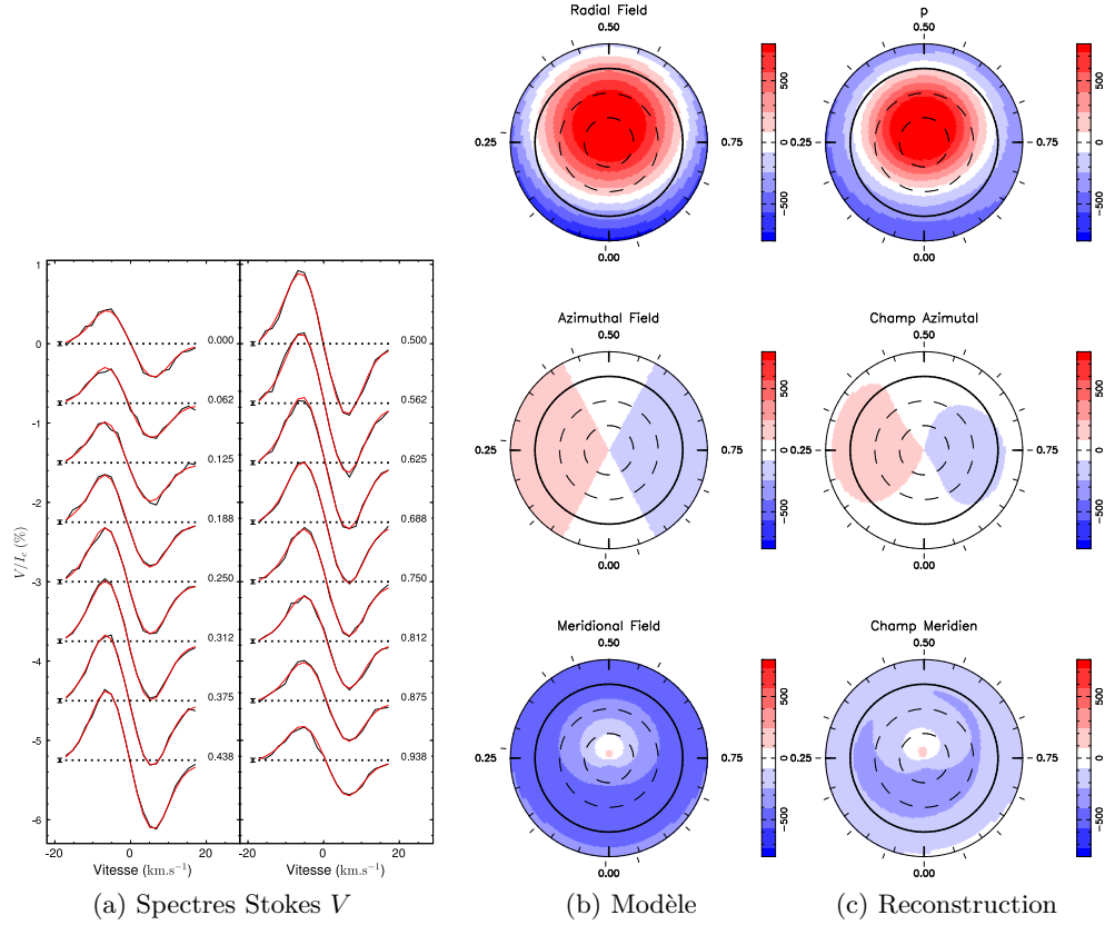
FIGURE 2.9 – Reconstruction d’une topologie simple. (b) Modèle de topologie magnétique à grande échelle représentée en projection polaire aplatie. Le pôle est au centre de l’image et les cercles concentriques représentent (de l’intérieur vers l’extérieur) les latitudes de 60^\circ , 30^\circ , 0^\circ et -30^\circ . Les tirets radiaux indiquent les 16 phases d’observations. Les paramètres stellaires sont i = 45^\circ , v \sin i = 3 \text{ km.s}^{-1} . Les paramètres de raie correspondent au profil LSD d’une étoile de type spectral M4. La topologie magnétique est un dipôle incliné de 20^\circ par rapport à l’axe de rotation, le champ au pôle vaut 1 kG. (a) Série de spectres polarisés, en noir les spectres calculés à partir du modèle de champ magnétique et bruités avec un rapport signal à bruit égal à 4000. Le trait rouge représente l’ajustement par le code ZDI avec \chi_r^2 = 1.0 , et \ell_{\max} = 2 . À gauche de chaque spectre est représentée une barre d’erreur \pm 1\sigma , et à droite la phase rotationnelle est mentionnée. (c) Topologie reconstruite par imagerie Zeeman-Doppler.
