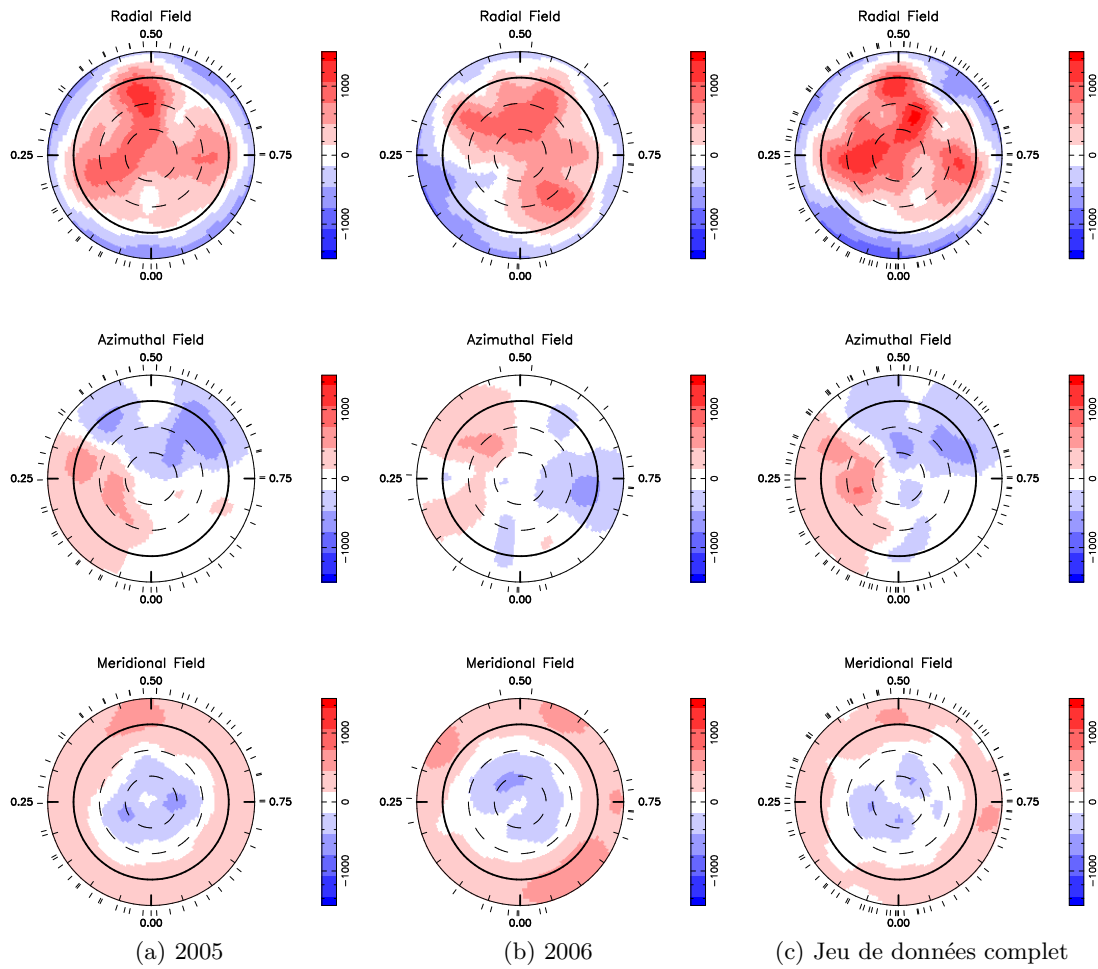
FIGURE 3.5 – Champ magnétique de surface de V374 Peg en projection polaire aplatie. Le cercle en gras représente l'équateur, le cercle extérieur et ceux en pointillés représentent (de l'extérieur vers le centre) les latitudes de -30^\circ , +30^\circ et +60^\circ . Chaque trait radial indique la position du méridien central au moment d'une observation. La figure de droite a été obtenue à partir de l'ensemble des données 2005 et 2006 en tenant compte de la rotation différentielle ( cf. 3.4.2). Elle représente la topologie magnétique à une époque intermédiaire.
