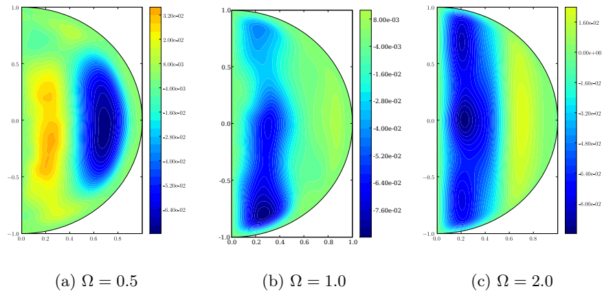
FIGURE 4.12 – Évolution de \langle U_\phi \rangle avec le taux de rotation.
