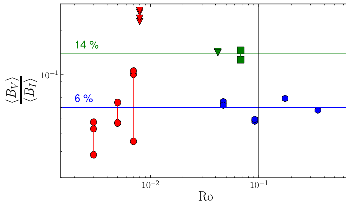
(b) Rapport des flux magnétiques mesurés à partir de Stokes V et I
