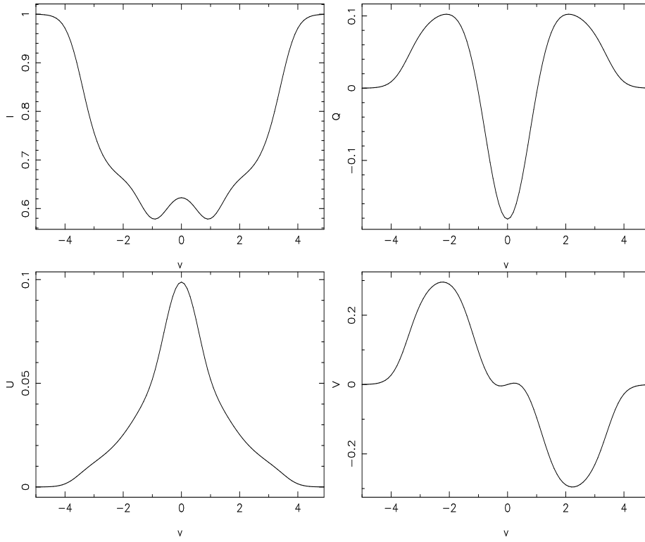
FIGURE A.1 – Paramètres de Stokes calculés avec la solution d’Unno-Rachkovsky, normalisés au continu et tracés en fonction de la fréquence réduite. Les paramètres utilisés sont \beta = \frac{B_1}{B_0} = 4 , \mu = 1 , \eta_0 = 10 , a = 0 , v_B = 2 , \theta = \frac{\pi}{4} et \chi = 0 .
