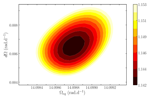
FIGURE 3.7 – Variation du \chi^2 en fonction des paramètres de rotation différentielle \Omega_{\text{eq}} et d\Omega . Le contour extérieur correspond à un accroissement de \chi^2 de 1%, i.e. une barre d'erreur de 7\sigma (pour chaque paramètre pris séparément).
