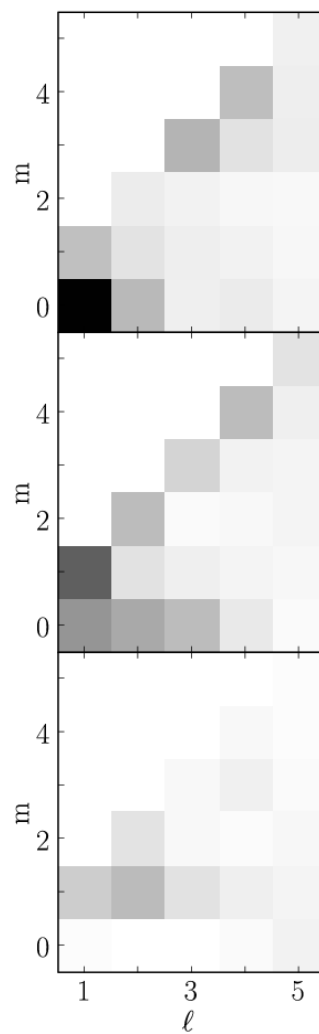
FIGURE 3.6 – Spectre d'énergie magnétique de V374 Peg, pour les données 2005, tronqué à \ell = 5 . Les trois panneaux représentent, de haut en bas, les modes \alpha_{\ell,m} , \beta_{\ell,m} et \gamma_{\ell,m} .
