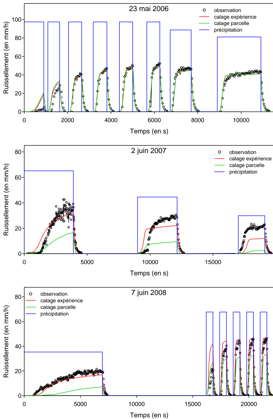
FIGURE 7.15 – Comparaison du modèle avec les observations pour la parcelle A désherbée avec les paramètres re-calés pour l'expérience ("calage expérience") et avec les paramètres globaux de la parcelle ("calage parcelle").
