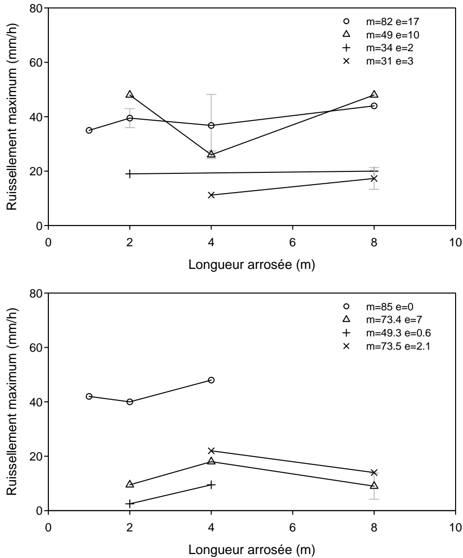
FIGURE 3.10 – Ruissellement en régime permanent en fonction de la longueur de versant arrosée pour la parcelle désherbée (en haut) et enherbée (en bas). Les barres d'erreur correspondent à l'écart-type des mesures et le point à la moyenne dans les cas où on a plusieurs mesures. Dans la légende, m et e correspondent respectivement à la moyenne et à l'écart-type de l'intensité de pluie.
