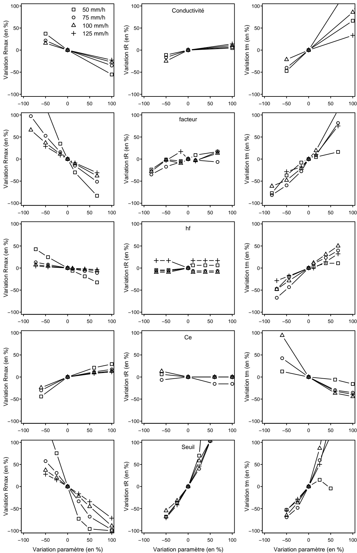
FIGURE 7.5 – Sensibilité de la conductivité, du facteur d’augmentation, le potentiel de front (hf), le coefficient de débit (Ce) et la hauteur du seuil sur le ruissellement maximal (Rmax), le temps d’apparition du ruissellement (tr) et le temps de montée (tm). Les différentes courbes correspondent à différentes intensités de pluie.
