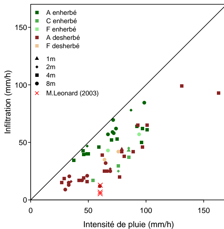
FIGURE 3.11 – Infiltration en régime permanent en fonction de l'intensité de pluie pour différentes parcelles et différentes longueurs arrosées. Les résultats des simulations de pluie effectuées par Leonard (2003) ont également été rajoutés.
