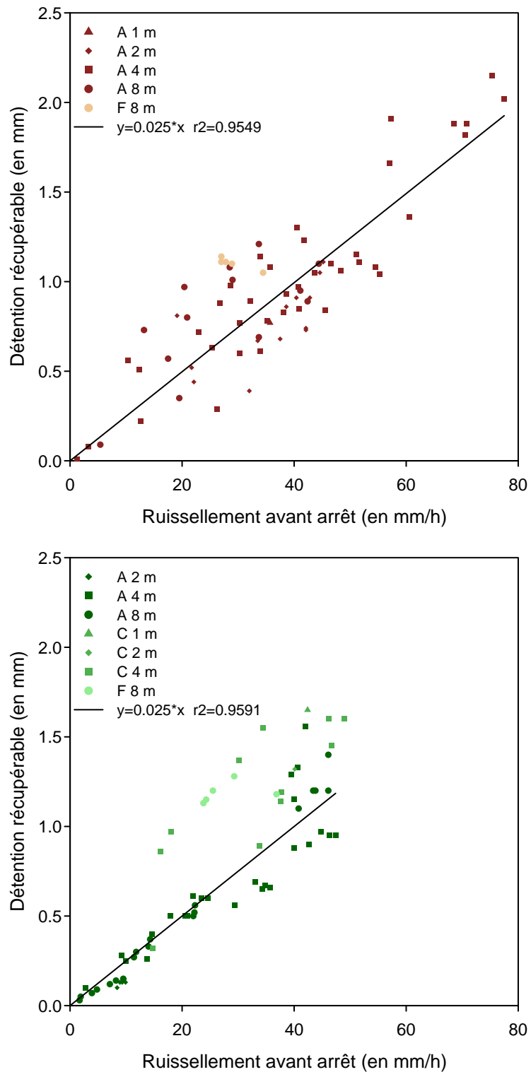
FIGURE 3.9 – Détection récupérable après arrêt de la pluie en fonction du ruissellement pour l'interrang dés herbé (en haut) et en herbé (en bas). Les droites de régression sont calculées uniquement sur les parcelles A de chaque interrang.
