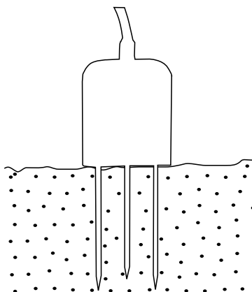
FIGURE 3.4 – Schéma d'un capteur diélectrique
