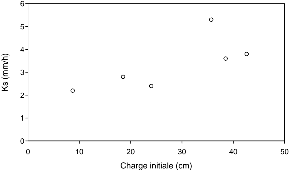
FIGURE 5.2 – Conductivité hydraulique à saturation de la céramique pour différentes charges (entre 8 et 43 cm).
