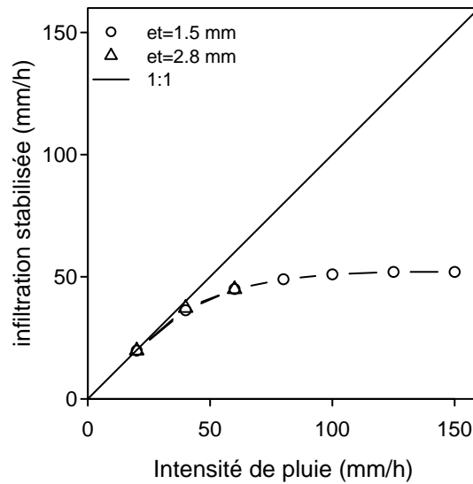
FIGURE 6.5 – Effet d’une répartition de K_s fonction de l’altitude de la microtopographie sur l’infiltration en régime quasi-permanent en fonction de l’intensité de pluie pour deux écart-types de microtopographie (1.5 et 2.8 mm).
