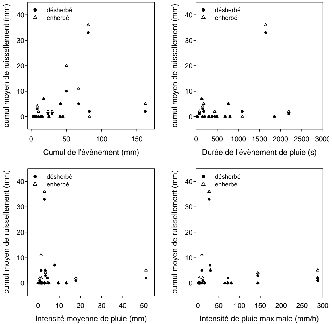
FIGURE 4.11 – Cumul de ruissellement moyen en fonction du cumul, de la durée, de l'intensité moyenne et de l'intensité maximale sur 5 s.
