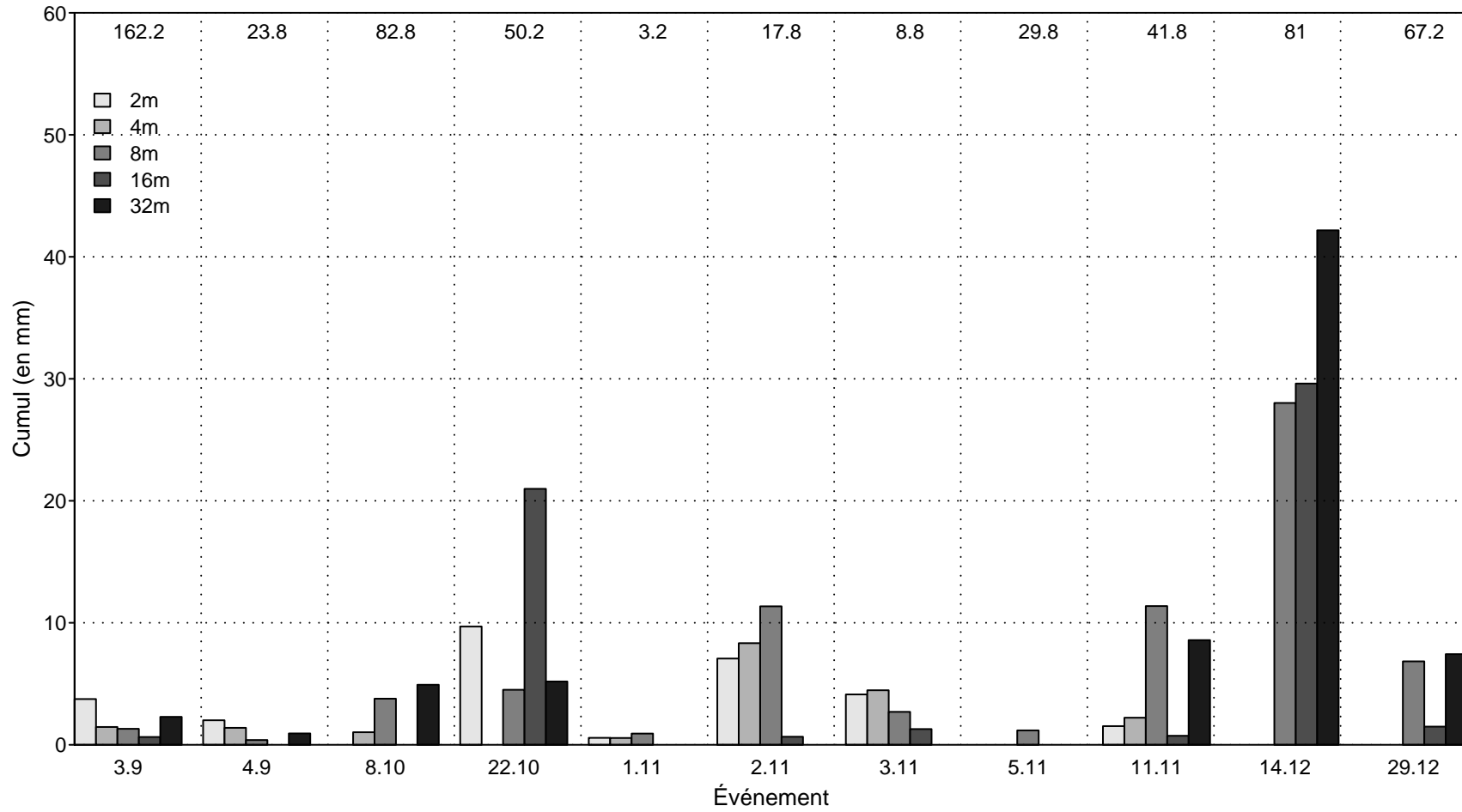
FIGURE 4.7 – Cumul de ruissellement pour chaque événement ruisselant pour la parcelle désherbée. Les nombres placés en haut correspondent aux cumuls de pluie de chaque évènement dont la date est notée en bas.
