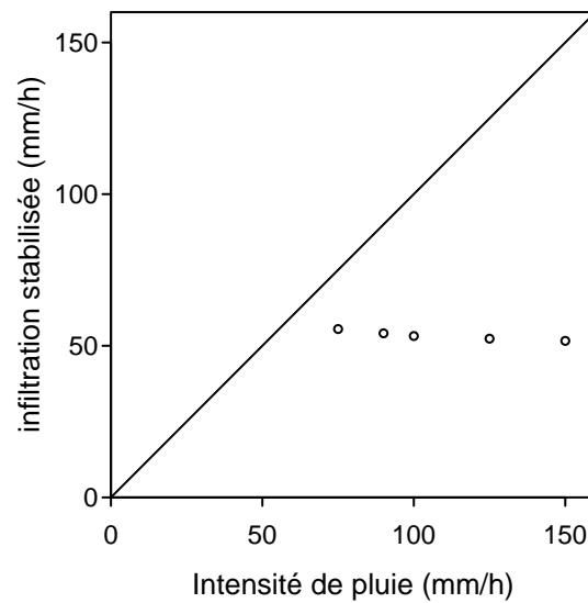
FIGURE 6.3 – Infiltration en régime pseudo-permanent en fonction de l'intensité de pluie pour un plan incliné et une conductivité à saturation uniforme.
