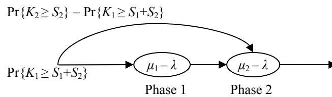
Figure 4.6. Représentation de D_2 par une loi de type phase
