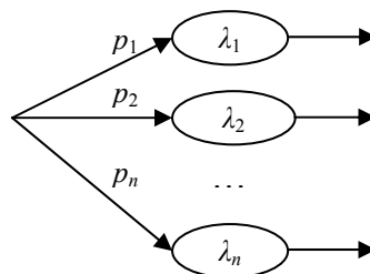
Figure C.2. Représentation de la distribution hyper-exponentielle
