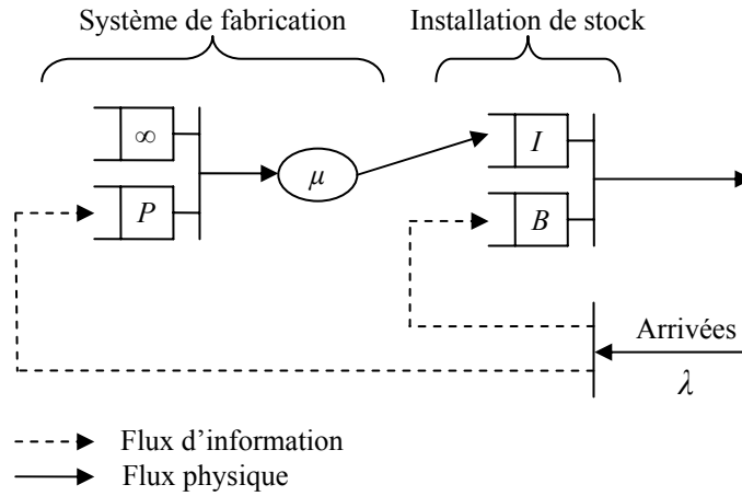
Figure 1.15. Représentation du système par les files d'attente
