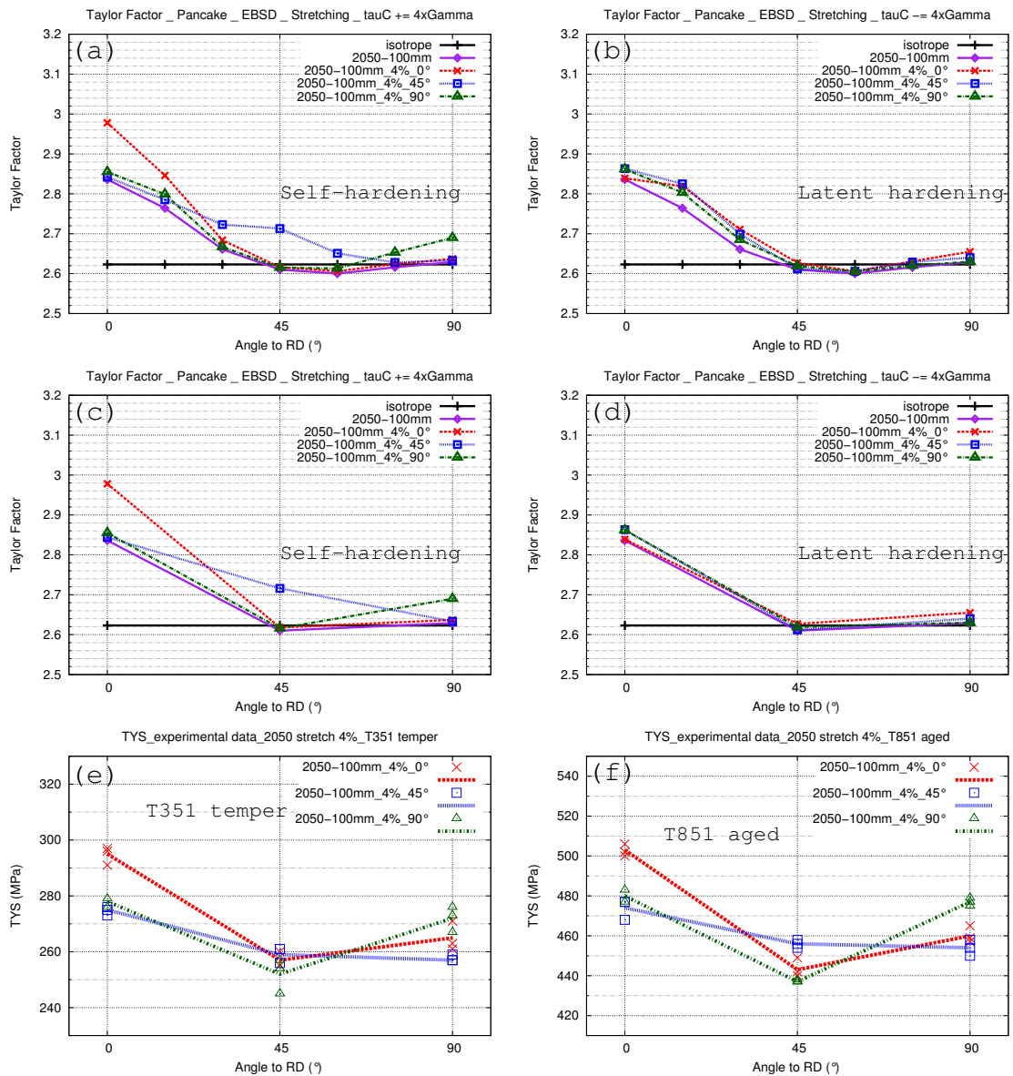
FIG. V.3: Modélisation de l'anisotropie par le calcul du facteur de Taylor après des détensionnements en traction à 0°, 45° et 90° d'après le modèle Taylor Pancake : (a) Durcissement des systèmes actifs durant le détensionnement (b) Durcissement des systèmes non actifs durant le détensionnement (c) idem a (d) idem b (e) Résultats expérimentaux 2050 100mm état T351 (f) Résultats expérimentaux 2050 100mm état T851.
