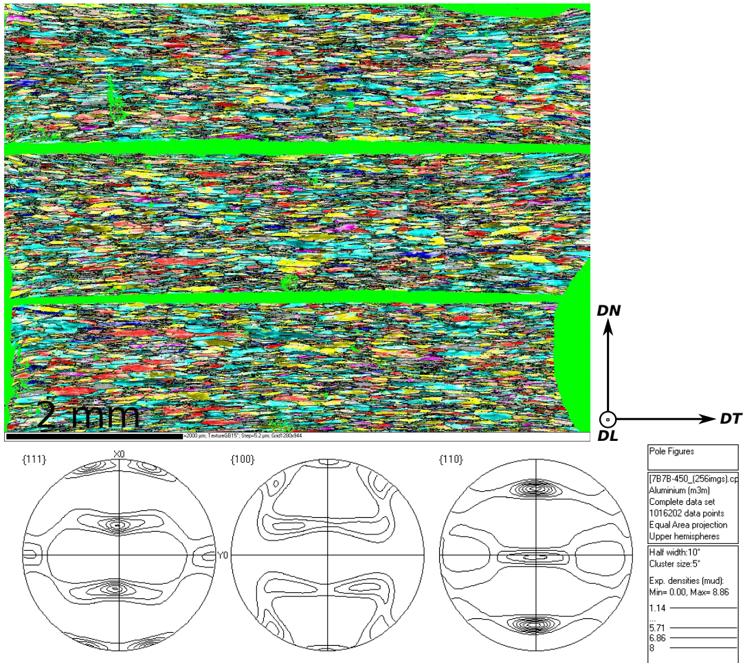
FIG. II.13: Cartographie EBSD de trois sections dans le plan DN-DT de l'alliage 7050 après compression plane encastree : \varepsilon = 2.25 , \dot{\varepsilon} = 1s^{-1} , T = 450^{\circ}C . Et les figures de pôle.
