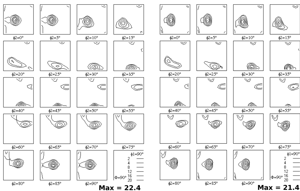
FIG. II.20: FDOC (EBSD) de tôles brut de laminage à mi-épaisseur, 2050 \varepsilon = 2.1 et 2050 \varepsilon = 2.9 . Logiciel Channel5, Lmax=22
