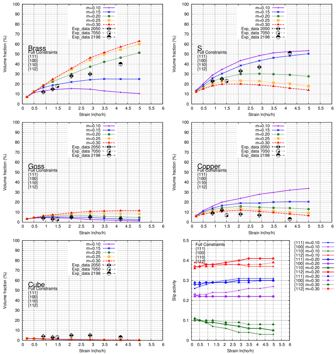
FIG. II.28: Evolution des principales composantes de texture de laminage d'après le modèle de Taylor "Full Constraints" incluant les plans de glissement \{111\} , \{100\} , \{110\} et \{112\} , pour différentes valeurs de m :
