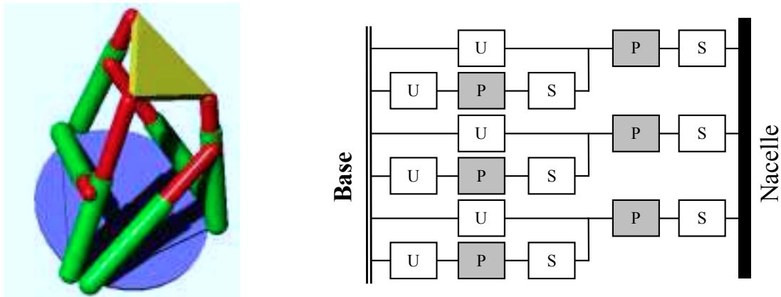
Figure I-15 : Plate-forme de Stewart.
