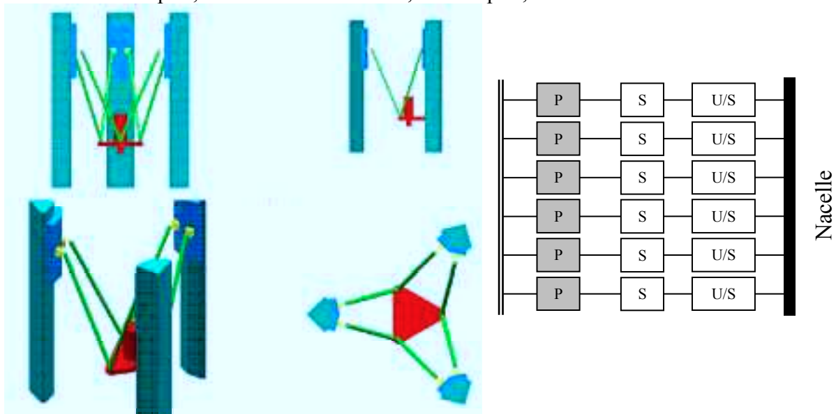
Figure IV-11 : Partie micro – Fraiseuse parallèle 5 axes.
