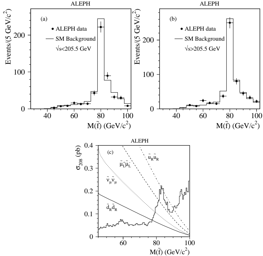
FIG. 3.10 – La masse invariante reconstruite des paire de jets pour les événements à quatre jets. L’histogramme en trait plein représente la prédiction du modèle standard. Les points correspondent au données mesurées. en c, les section efficaces maximum pour les sleptons et les sneutrinos (LQD) et les squark (UDD) se désintégrant directement sont montrées. Les sections efficaces de sneutrinos, smuons et squarks sont superposées [30].
