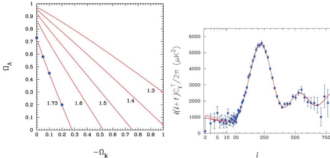
FIG. 4.12 – Les dégénérescences entre paramètres de courbure et de constante cosmologique avec une mesure du CMB isolée. Les quatres points de couples (\Omega_k, \Omega_\Lambda) différents présentés sur la figure de gauche correspondent aux courbes présentées sur la figure de droite qui se trouvent quasiment superposées et indiscernables avec les points de mesure actuels [55].
