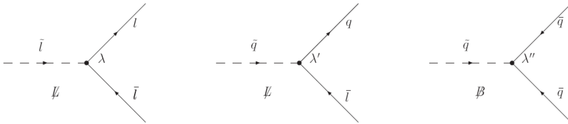
FIG. 3.2 – Les trois couplages associés aux couplages de Yukawa brisant les nombres leptoniques ou baryoniques
