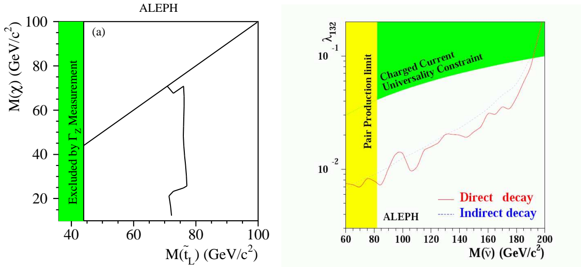
FIG. 3.9 – A gauche, la limite à 95% de niveau de confiance dans le plan (m_\chi, m_{\tilde{t}_L}) pour une désintégration indirecte avec le couplage UDD dominant [30]. A droite, les limites sur le couplage \lambda_{132} en fonction de la masse du sneutrino produit en mode singlet [31].
