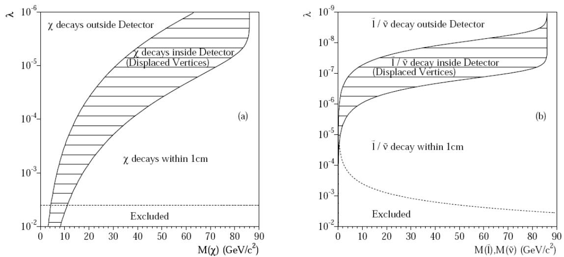
FIG. 3.5 – Région, dans le plan masse de la particule/couplage \lambda , où la particule a une longueur de désintégration L_j \approx 1\text{cm} , 1_j L_j \approx 3\text{m} (grand vertex déplacé) et L_j \approx 3\text{m} (en dehors du détecteur). Pour un neutralino ( m_f=100\text{ GeV} ) a) et un slepton ou neutrino b) [28]
