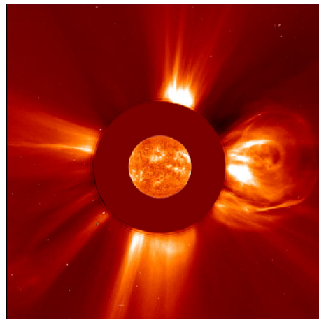
FIGURE 1.7 – Éruption solaire intervenue le 2 avril 2001
