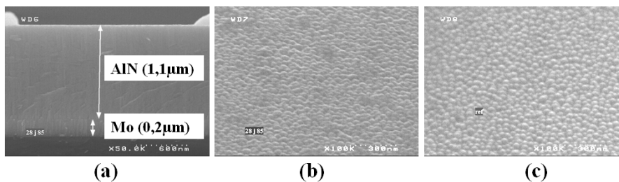
FIG.3-33: (a) Vue section MEB du dépôt d'AlN après 672 heures (28 jours), (b) Surface AlN vieillie, (c) Surface AlN référence
