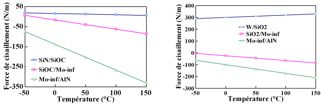
FIG.3-46: Force de cisaillement en fonction de la température pour les interfaces Bragg3/Bragg4 , Bragg4/Mo-inf et Mo-inf/AlN pour (a) SMR1 et (b) SMR2
