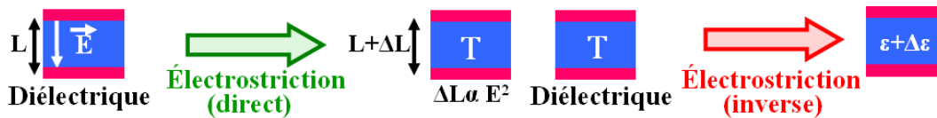
FIG.2-35 : Effet électrostrictif direct et inverse dans un diélectrique
