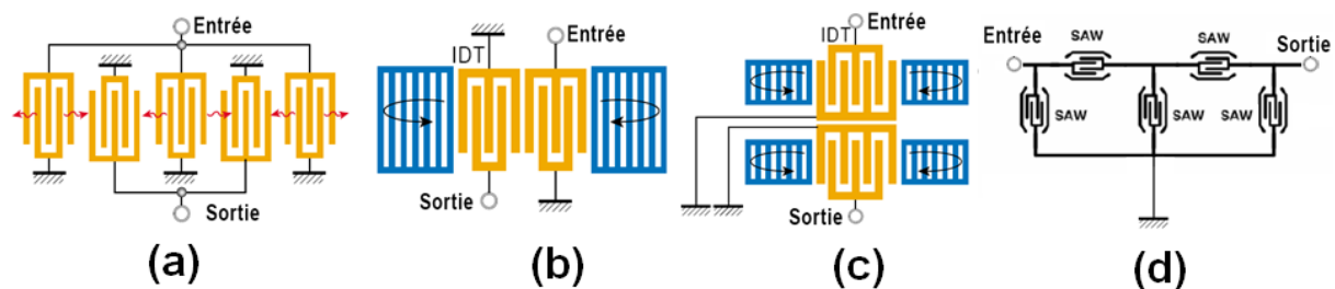
FIG.1-9: Vue supérieure de quelques structures de base des filtres SAW [R.1.31-R.1.72] :(a) IIDT (b) DMS à Couplage longitudinal (c) DMS à Couplage transverse et (d) filtre SAW à résonateurs en échelle d'ordre 5 (en jaune les transducteurs, en bleu les parois réfléchissantes)
