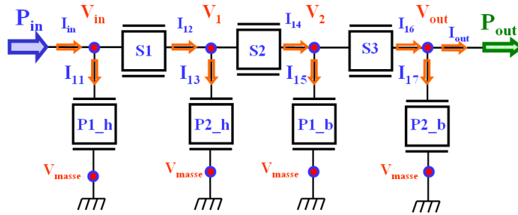
FIG.4-6: Méthode de calcul de la puissance dissipée dans chaque résonateur par extraction des couples courant I et tension V dans chaque nœud du circuit équivalent
