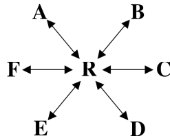
Figure 9. Plan en référence et en « dye swap » à six conditions (12 lames). Les six lames sont systématiquement comparées à la même référence. Les doubles flèches indiquent que chaque hybridation est répétée sur une autre lame en inversant les fluorochromes « dye swap ».
