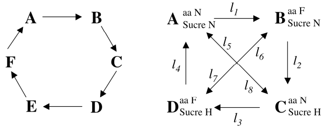
Figure 10. Deux types de plans en boucle. A gauche, un plan en boucle classique avec six conditions et six lames ; à droite, le plan de l'expérience AAS (quatre conditions, huit lames), incluant des croisements supplémentaires entre les quatre conditions qui représentent deux facteurs de l'expérience (acides aminés et sucre) à deux niveaux (N - F et N - H).
