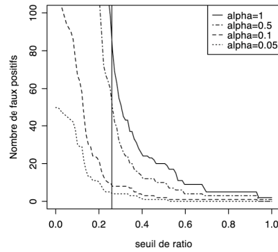
Figure 12. Nombres de faux positifs de l'expérience AAS pour différentes valeurs de \alpha et différentes valeurs de seuil de rapports d'expression (exprimé en valeur absolue du \log_2 ).
