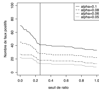
Figure 13. Nombres de faux positifs de l'expérience YF pour différentes valeurs de \alpha et différentes valeurs de seuil de rapport d'expression (exprimé en valeur absolue du \log_2 ).
