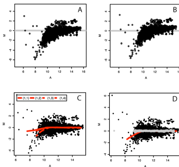
Figure 16. Illustration de différentes méthodes de normalisation. A : données non normalisées (lame 1 de l'expérience AAS), B : normalisation par la médiane, C : normalisation loess par aiguille, D : normalisation loess sur un jeu de gènes invariants (en gris).
