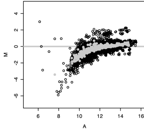
Figure 15. Détection des gènes invariants par la méthode de Tseng et al. (2001). Lame 1 du jeu de données AAS. Les gènes invariants sont en gris.
