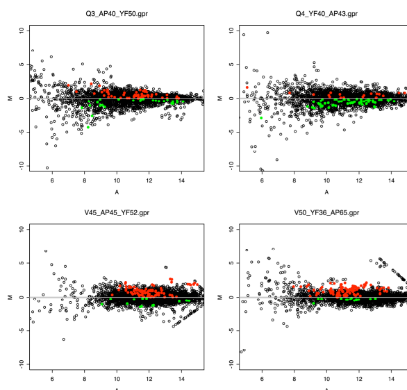
Figure 20. Graphes des \log_2 des rapports d'expression normalisés (M) en fonction de l'intensité du marquage (A) dans une expérience en « dye swap ». En rouge sont représentés les ARNt caractérisés par des valeurs positives, en vert sont pointées les valeurs négatives. Le « dye swap » est bien visible pour l'hybridation manuelle (en haut) alors qu'un biais systématique rouge est observé avec l'hybridation automatique (en bas).
