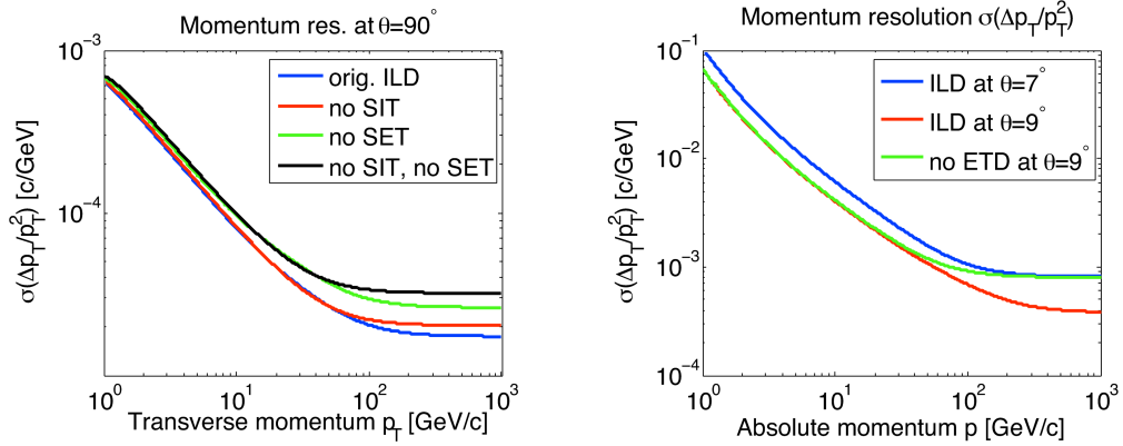
FIG. 3.4 – Résolution du moment transverse (à gauche) et résolution du moment absolu du trajectographe (à droite).
