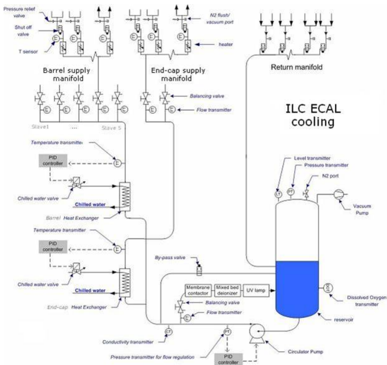
FIG. 3.15 – Système de thermalisation 1- en haut : détecteur ILD ; 2- en bas : système global de thermalisation
