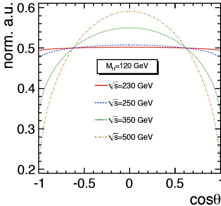
FIG. A.4 – Distribution angulaire de production du boson de Higgs, voir texte.
