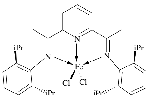
Figure 8 : Structure du précatalyseur bis(arylimino)pyridine-FeCl 2 actif, après traitement par le cocatalyseur MAO, en polymérisation de l'éthylène.
