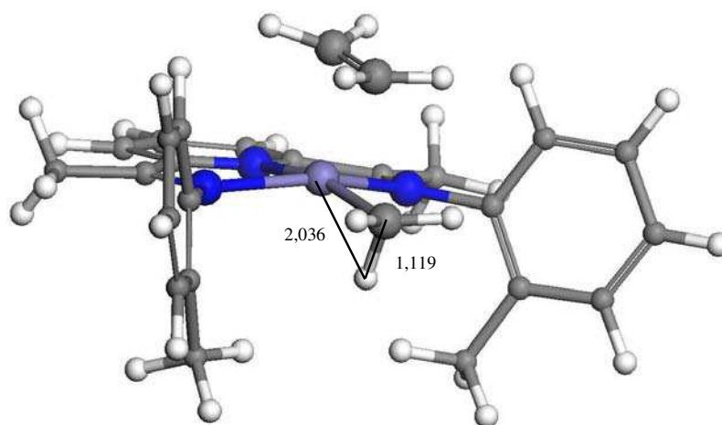
Figure 10 : Vue de l'interaction Fe-H \alpha agostique pour l'état doublet [1-2(III)Me] 2+ (approche anti ) (les distances interatomiques sont en angströms) (en blanc = atomes d'hydrogène ; en gris = atomes de carbone ; en bleu = atomes d'azote ; en violet = atome de fer).
