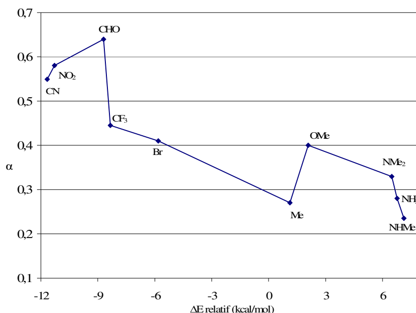
Figure 17 : Évolution du coefficient \alpha , extrait de la relation (6.7), en fonction des substituants X classés selon leur valeur \Delta E relative issue de la méthode de calculs de Hammett (Tableau 6); noter que les connections entre les différents points n'ont pas de sens physique mais servent à montrer une tendance.
