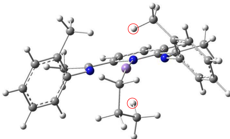
14. Structure optimisée de Mn_{II}^{\gamma\delta} : charge = +1, multiplicité = 2.
