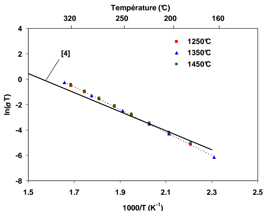
Figure III.A. 7 : Variation de la conductivité de grain de l'électrolyte CGO en fonction de la température obtenue pour les trois protocoles de frittage, et comparé à un résultat obtenu par Cheng et co. [4]
