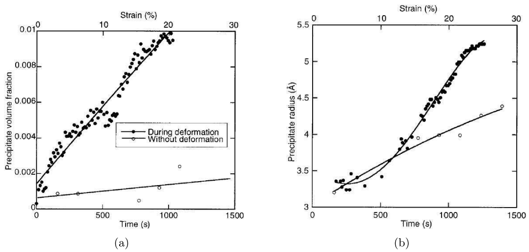
FIG. 2.4: (a) Évolution de la fraction volumique précipitée et (b) du rayon moyen des précipités à température ambiante, en précipitation statique (points blancs) et dynamique ( \dot{\epsilon} = 10^{-4} ) (points noirs) [Deschamps et al., 2003].
