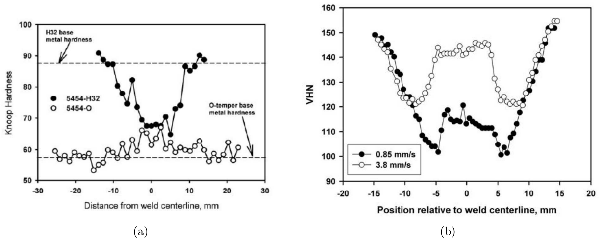
FIG. 5.5: (a) Profils de dureté d'un joint soudé par FSW d'un alliage AA5454 soit dans un état écroui (symbole H) soit dans un état recuit (symbole O) [Reynolds, 2007]. (b) Profil de dureté d'un joint soudé par FSW à deux vitesses de soudage différentes pour un AA7050-T74 [Reynolds, 2007].
