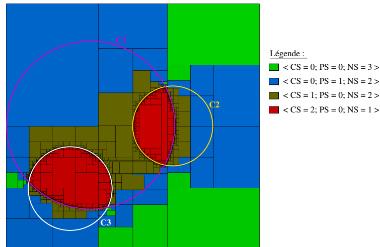
Figure 3.13 – Application de l'algorithme d'extension intérieure présenté en table 3.6 à un problème d'intersection de trois cercles C1 , C2 , C3 . La méthode recupèreConfiguration est instanciée par un choix de point médian. Le temps de résolution est de 0.87 secondes. L'algorithme a effectué 4261 itérations et une boîte maximale ( c.-à-d. satisfaisant 2 contraintes) a été trouvée au bout de 3 itérations. Le domaine de recherche est de \{[-3, 3], [-3, 3]\} pour les variables X et Y mises en jeu; la précision de bisection est de 0.01.
