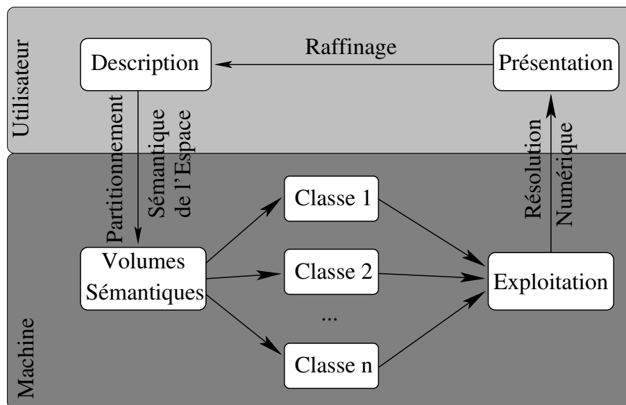
Figure 4.4 – Schéma global de l'approche des volumes sémantiques.
