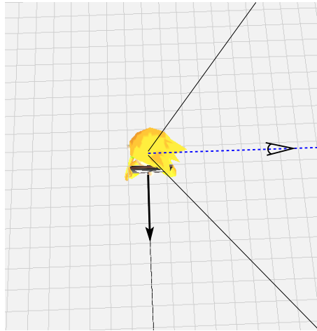
Figure 4.17 – Illustration d'une position de caméra maximisant la propriété « Voir Calvin de profil gauche ».
