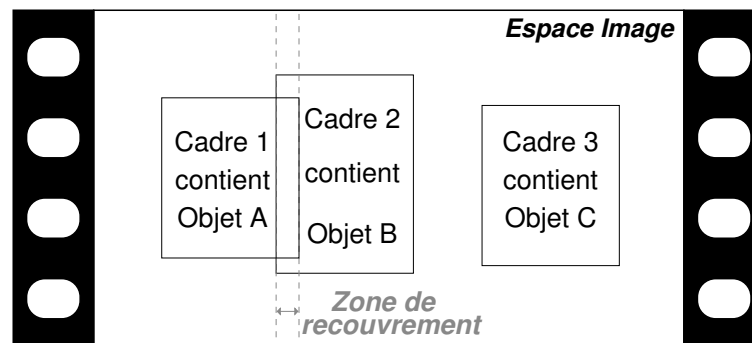
Figure 4.15 – Une description utilisateur comportant des propriétés de framing avec chevauchements des cadres.
