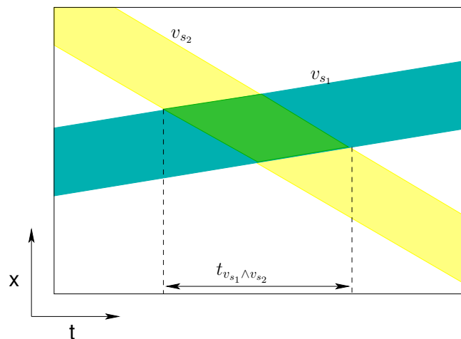
Figure 4.39 – Intersection volumes sémantiques temporels, la représentation des volumes est abstraite à la composante X dans un souci de clarté de la représentation.
