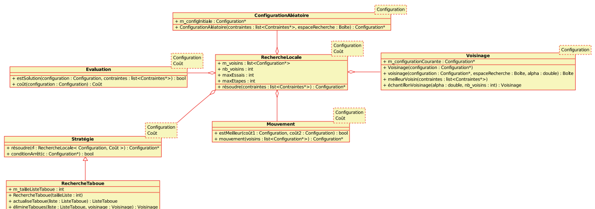
Figure C.1 – Diagramme de classes de l'implémentation de l'extension de la recherche locale avec recherche taboue aux domaines continus.
