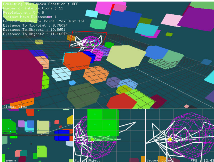
Figure 5.29 – Illustration d'une scène composée de 98 objets occultants ayant des trajectoires cycliques aléatoires.
