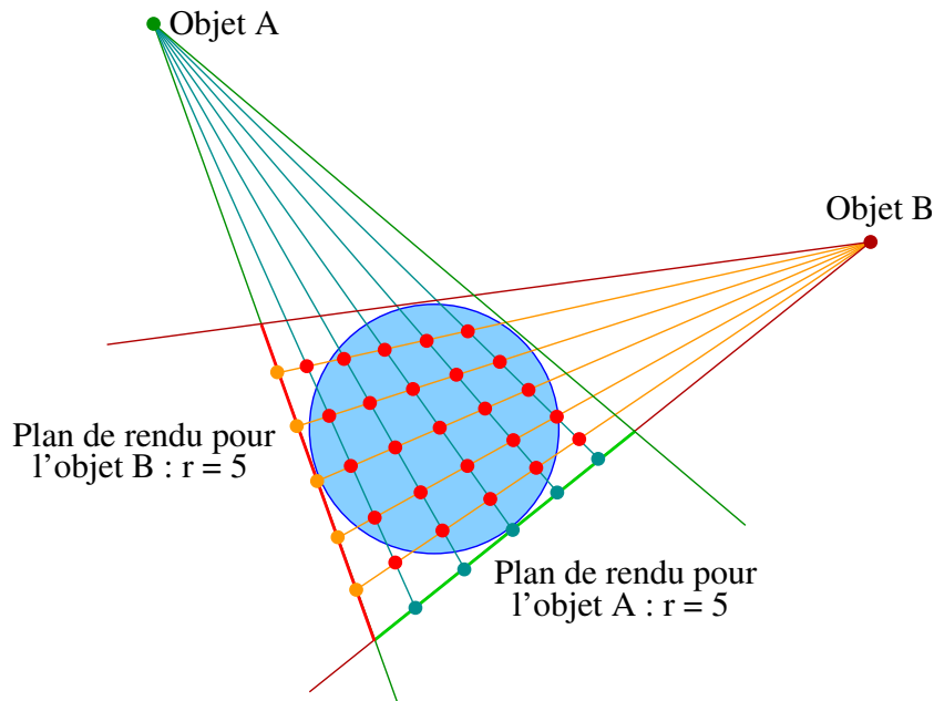
Figure 5.14 – Calcul du nombre d'intersections générées en fonction de la résolution (c.-à-d. d'un nombre de rayons) du plan de rendu.
