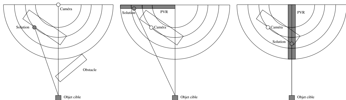
(a) Recherche non contrainte d'un bon point de vue grâce à la méthode PVR . (b) Recherche sous contrainte : l'utilisateur a spécifié un PVR favorisant l'obtention d'un profil gauche de l'objet ciblé. (c) Recherche sous contrainte : l'utilisateur a spécifié un PVR favorisant l'obtention d'une vue de face de l'objet d'intérêt
