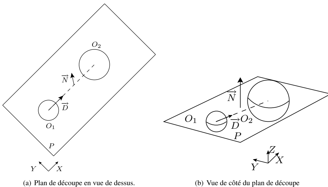
Figure 4.24 – Plan de découpe lié à la propriété de positionnement relatif gauche/droite à l'écran.
