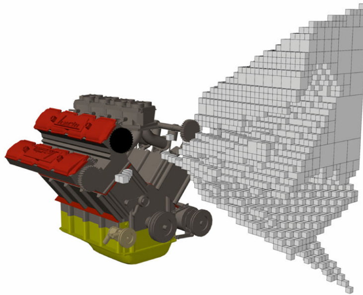
Figure 2.15 – Modélisation des régions potentiellement intéressantes de l'espace de recherche à l'aide d'arbres octaux d'après Pickering [Pic02].
