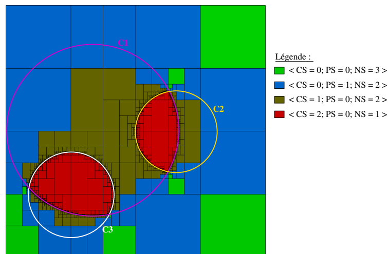
Figure 3.11 – Application de l'algorithme d'extension intérieure présenté en table 3.6 à un problème d'intersection de trois cercles C1 , C2 , C3 . Le temps de résolution est de 1,19 secondes. L'algorithme a effectué 5431 itérations et une boîte maximale ( c.-à-d. satisfaisant 2 contraintes) a été trouvée au bout de 41 itérations. Le domaine de recherche est de \{[-3, 3], [-3, 3]\} pour les variables X et Y mises en jeu; la précision de bissection est de 0.01.
