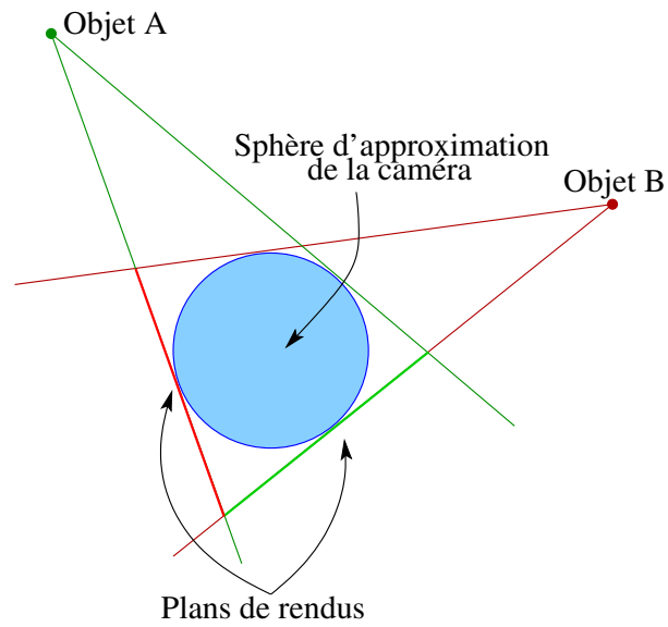
Figure 5.10 – Pyramides de vue tangentes à la sphère d'approximation de la caméra.
