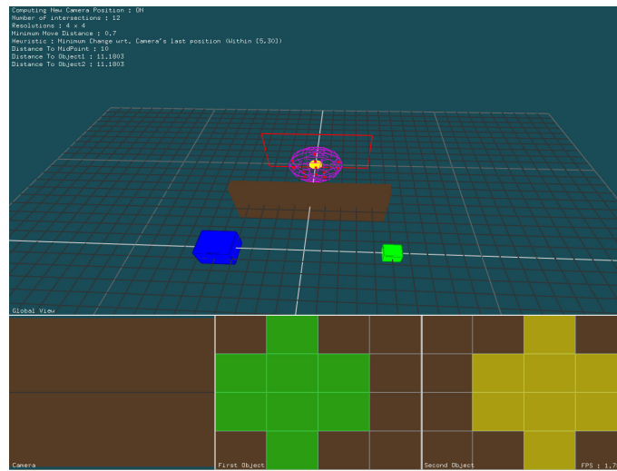
Figure 5.24 – Illustration d’une occultation des deux objets d’intérêt O_1 et O_2 dans le prototype OCCLUSION AVOIDER. Les points d’intersection appartenant à la sphère d’approximation sont affichés en rouge pour signaler que les deux objets d’intérêt sont occultés.
