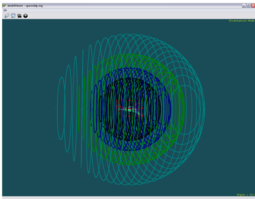
Figure 5.30 – Points de vue générés par le MODELVIEWER autour d'un modèle 3D à partir desquels une structure de données est créée afin d'ajouter des informations lors de l'évitement d'occlusions par l'application OCCLUSION AVOIDER.
