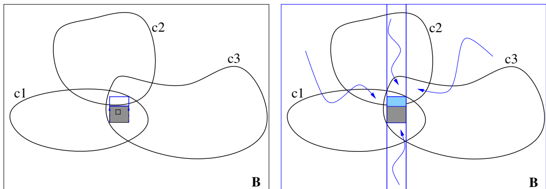
(c) Réduction autour de la région prometteuse par propagation des contraintes potentiellement satisfaites : c2 . (d) Itération sur les domaines restants, rajout de la zone propagée à la liste des boîtes à traiter et abandon de la boîte grisée.
