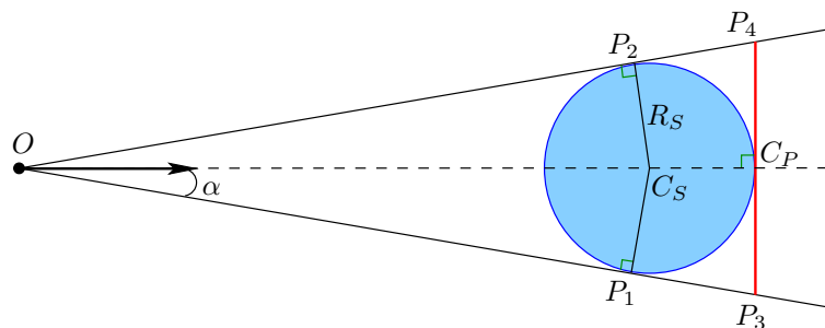
Figure 5.11 – Illustration de la construction d'une pyramide tangente à une sphère S .
