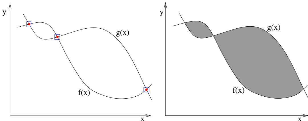
(a) Relation à solutions ponctuelles : f(x) = g(x) . Elle est représentée par les points rouges entourés de carrés bleus. (b) Relation présentant deux continums de solutions est représentée par les régions grisées : y \leq g(x) \wedge y \geq f(x) .
