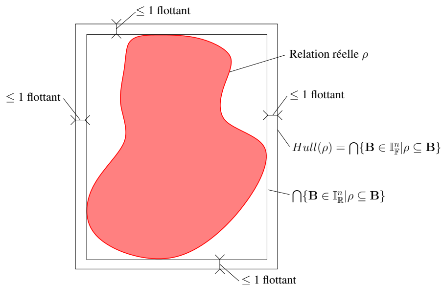
Figure 3.6 – Illustration de l'opérateur Hull qui calcule la plus petite boîte à bornes flottantes englobant une relation réelle \rho .
