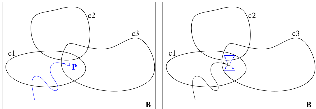
(a) À la recherche d'un « bon » point de départ, le pavé P . (b) Extension intérieure de P par rapport aux contraintes certainement satisfaites c1 et c3 .
