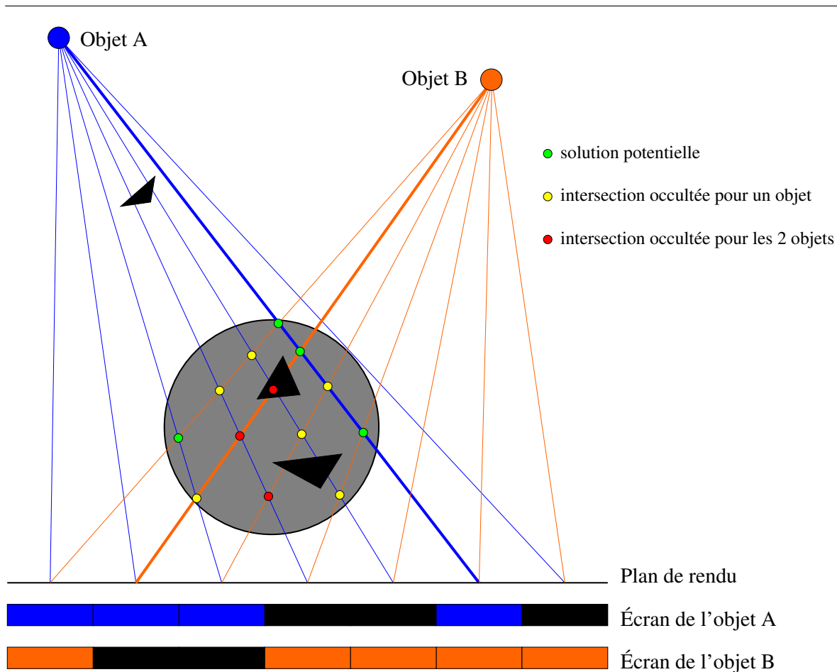
Figure 5.20 – Création des « rayons » issus des objets pour le rendu de la scène vers la sphère des positions futures de caméra. Les statuts d'occlusion des intersections sont gérés en prenant en compte les informations de profondeur des depth buffers afin de déterminer s'ils sont ou non situés devant les occultants et correspondent à une solution potentielle.
