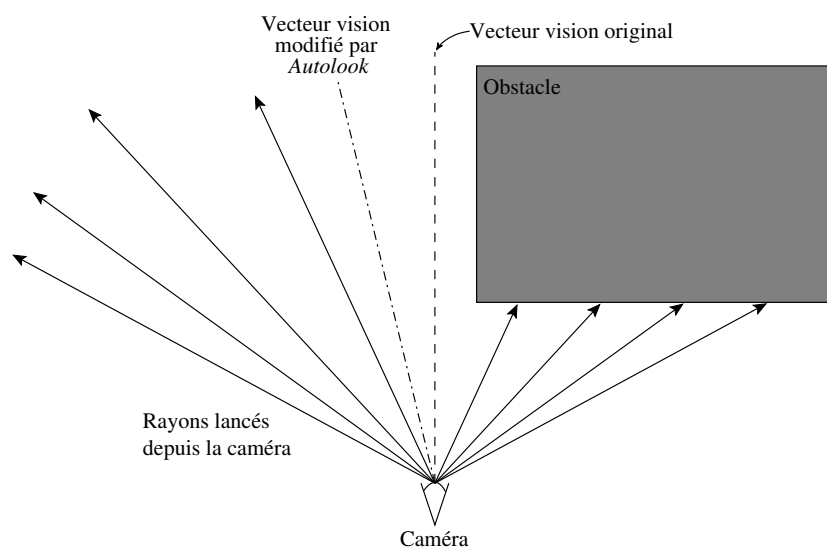
Figure 5.1 – Illustration du système Autolook [Gio04] en vue de dessus. Le système lance des rayons à droite et à gauche de la position courante de caméra. En fonction des intersections, le vecteur vision est modifié afin de limiter la place des obstacles à l'écran. Ici les rayons gauches ne rencontrent aucune intersection alors que ceux de droite rencontrent un obstacle. Le vecteur vision est donc décalé sur la gauche afin de limiter l'affichage de l'obstacle à l'écran ( Autolook ne modifie que l'orientation de la caméra, pas sa position).
