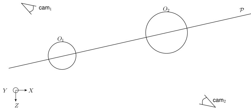
Figure 4.11 – Vue de dessus d'un plan de coupe défini pour la propriété de positionnement relatif « Gauche/Droite » des objets O_1 et O_2 à l'écran.
