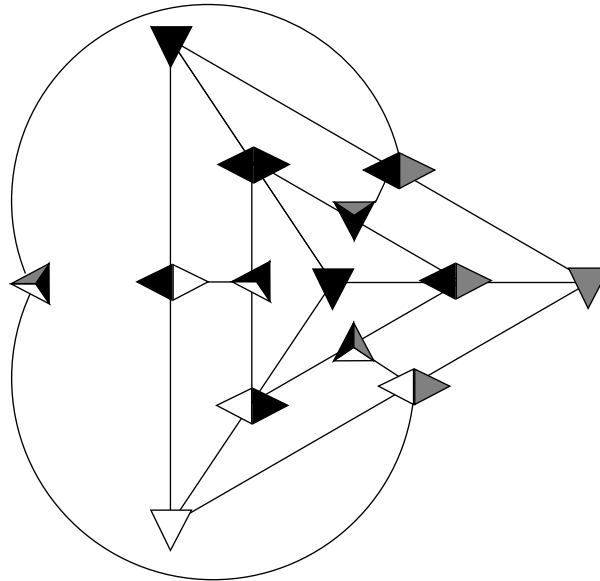
Figure 4.2 – Graphe d’aspects d’un tétraèdre, d’après Koenderink et van Doorn [KvD79]. On distingue trois types d’aspects suivant le nombre de faces visibles à partir d’un point de vue.
