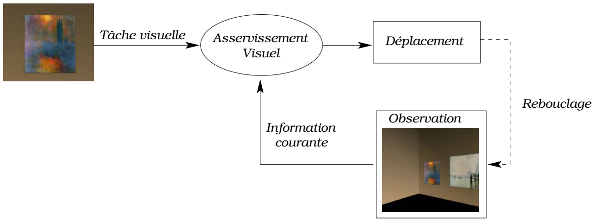
Figure 2.8 – Boucle fermée de l'asservissement visuel, d'après Courty [Cou02].
