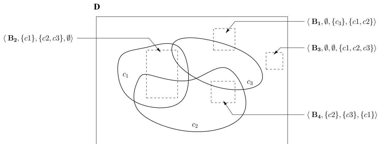
Figure 3.9 – Caractérisation \mathcal{CPN} des pavés \mathbf{B}_1, \mathbf{B}_2, \mathbf{B}_3 et \mathbf{B}_4 d'un espace de recherche D en fonction de trois contraintes numériques c_1, c_2, c_3 .
