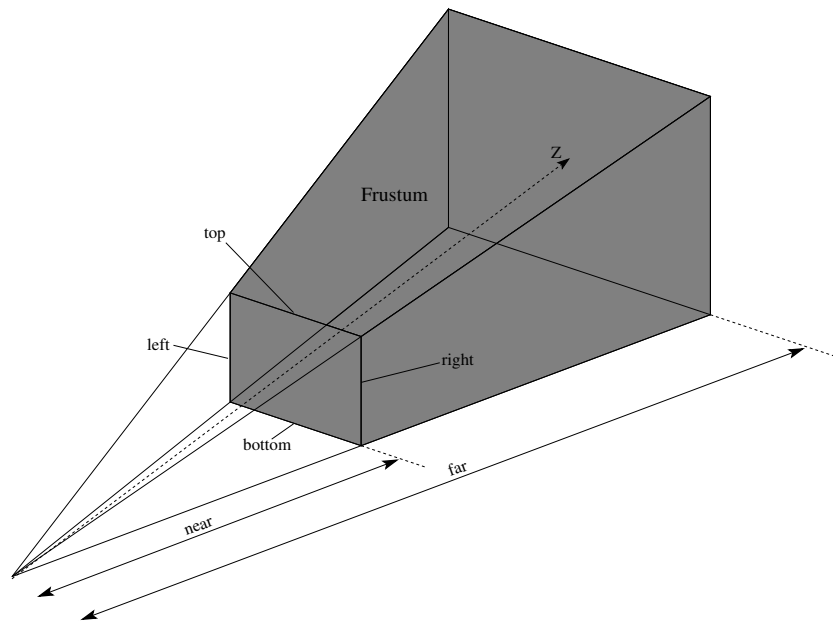
Figure 5.18 – Pyramide de vue OpenGL créée par un appel à la fonction glFrustum avec les paramètres left , right , bottom , top , near et far , d'après Shreiner et al. [SWND05].
