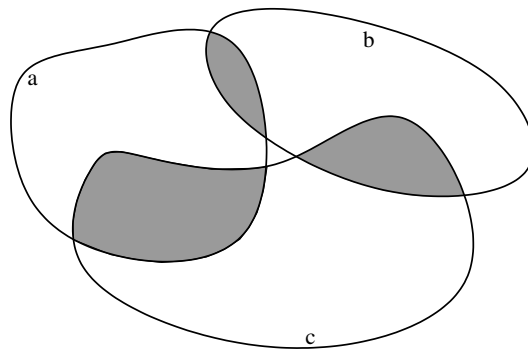
Figure 3.2 – Illustration de l'approche MAX-NCSP appliquée à trois relations a , b et c . Les zones maximisant le nombre de contraintes satisfaites apparaissent en grisé.
