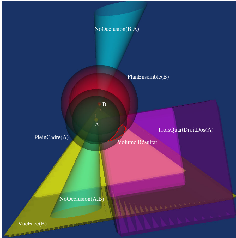
Figure 4.27 – Volumes sémantiques générés par le processus de partitionnement sémantique de l’espace de recherche et affichés par la librairie VTK. L’intersection de ces volumes correspond aux positions de caméra solutions de l’ over-the-shoulder .
