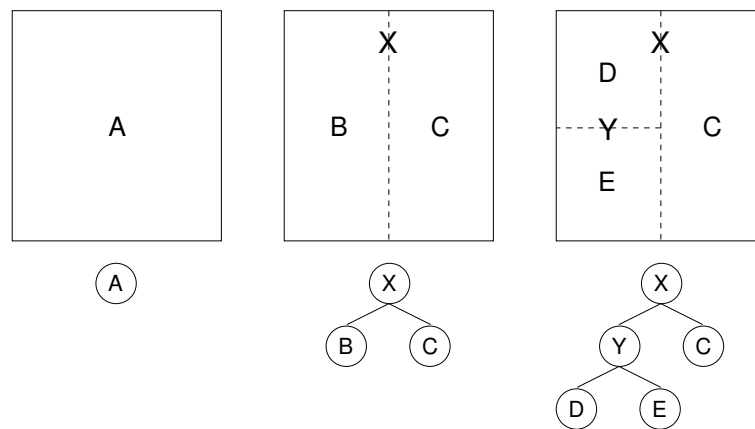
Figure 4.1 – Arbre BSP de découpe d’un polygone suivant l’axe X puis l’axe Y.
