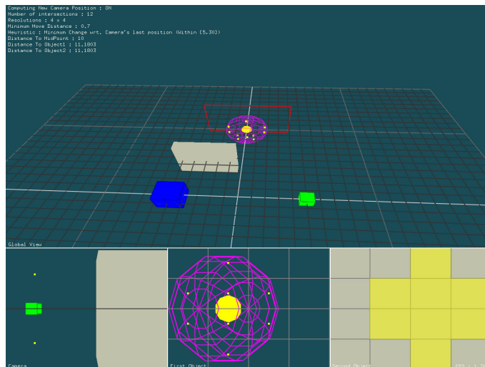
Figure 5.23 – Illustration d’une occultation de l’objet O_2 , représenté par un cube bleu, dans le prototype OCCLUSION AVOIDER. Les points d’intersection appartenant à la sphère d’approximation sont affichés en jaune pour signaler que l’objet O_2 est occulté.
