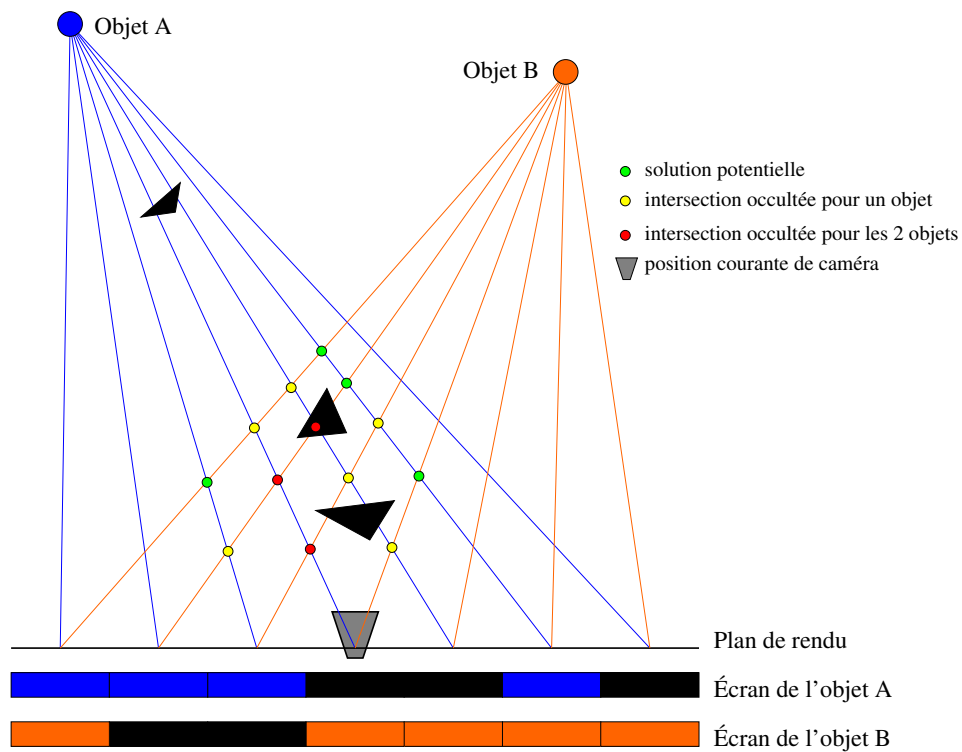
Figure 5.7 – Illustration de notre approche d'évitement de l'occlusion. Des rendus de la scène sont effectués depuis les objets dans des tampons de profondeur (les écrans) afin de déterminer si les points d'intersection correspondent à des positions non occultées de caméra (points vert), occultées pour un des objets (points jaune) ou pour les deux objets d'intérêt (points rouge). Les occlusions sont détectées grâce aux distances entre les points candidats, les objets occultants (triangles noirs) et les objets d'intérêt.
