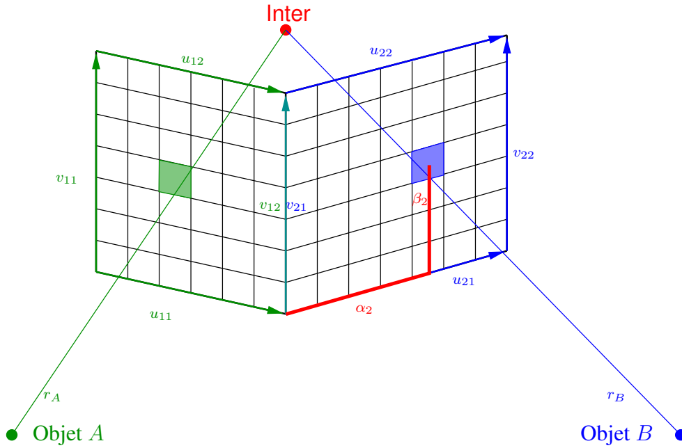
Figure 5.17 – Détermination des coordonnées des rayons r_A et r_B dans les systèmes multi-linéaires à partir des coordonnées globales du point d'intersection Inter de ces deux rayons.
