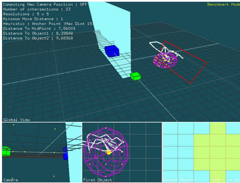
Figure 5.28 – Illustration de l'aller-retour d'un objet occultant devant les objets d'intérêt.
