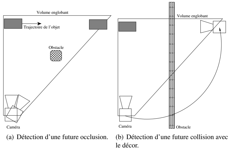
Figure 5.3 – Prévision d'occlusion et/ou de collision grâce à des volumes prédictifs, d'après [Cou02].
