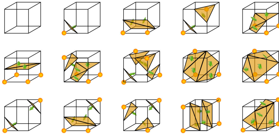
Figure 4.20 – Principe de l’algorithme du Marching Cubes . Le maillage est calculé en fonction des positions d’un cube unitaire par rapport à la surface que l’on souhaite reconstruire.
