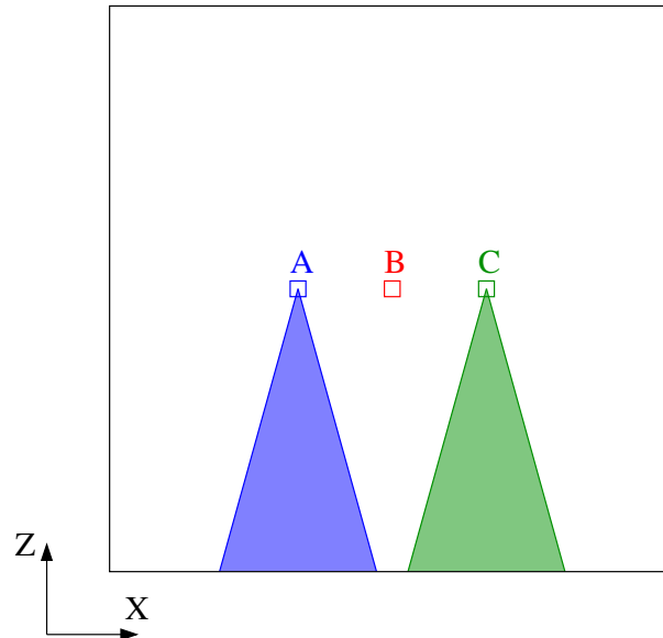
Figure 3.18 – Vue de dessus de l’espace de recherche associé au problème de composition visuelle. Les zones bleues et vertes correspondent aux positions de caméra pouvant amener à voir les objets A et C de face. L’espace de recherche représenté a une taille de [-3, 3] sur les deux dimensions X et Z .
