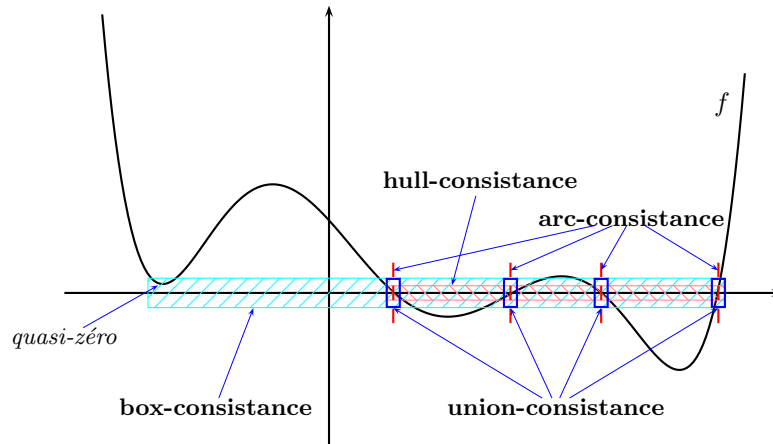
Figure 3.7 – Illustration de différentes consistances locales, d’après Goualard [Gou00].
