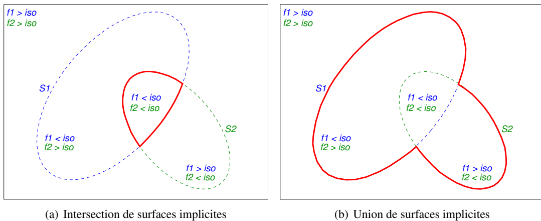
Figure 4.19 – Illustration de l’union et de l’intersection de deux surfaces ( S_1 et S_2 ) définies par les fonctions de potentiel f_1 et f_2 . Les équations des surfaces résultats des opérations Booléennes sont : \min(f_1, f_2) = iso (a), qui représente l’intersection des deux champs de potentiels; et \max(f_1, f_2) = iso (b) qui représente leur union.
