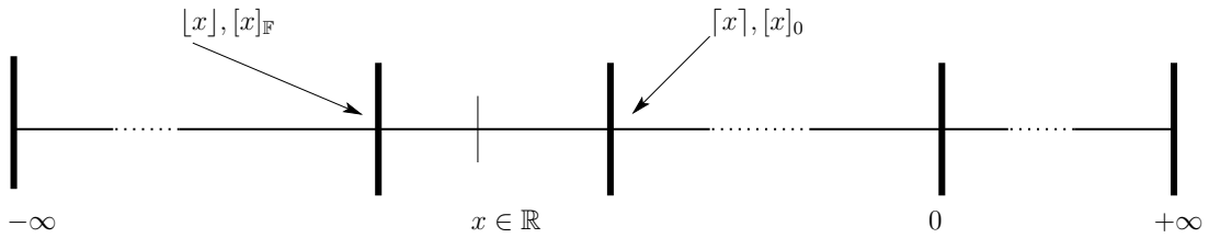
Figure 3.5 – Les différents modes d’arrondis d’un nombre réel x définis par la norme IEEE 754, d’après Goualard [Gou00].
