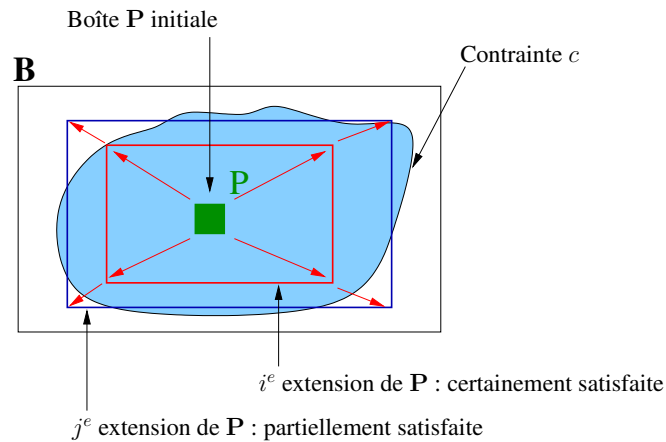
Figure 3.8 – Illustration de l’opérateur OEI (cf. table 3.3) d’extension intérieure appliqué à une contrainte bidimensionnelle.
