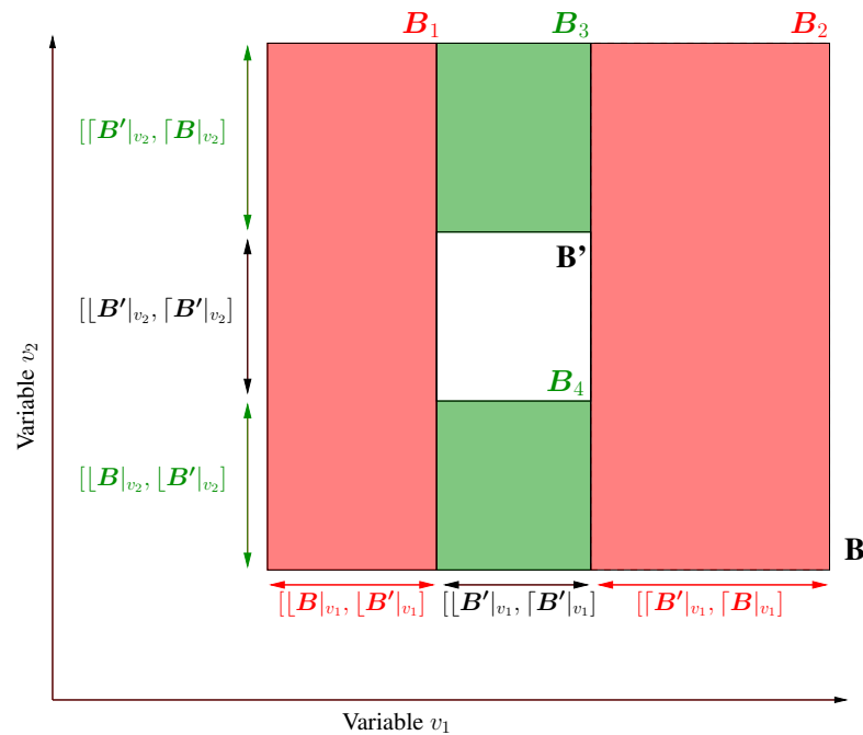
Figure 3.14 – Différence entre deux boîtes \mathbf{B} et \mathbf{B}' en deux dimensions.
