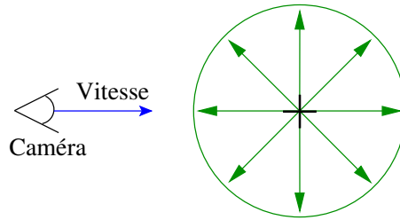
Figure 5.9 – Approximation des positions futures d'une caméra en mouvement par une sphère dont le rayon représente une accélération maximale uniforme : la sphère d'approximation.
