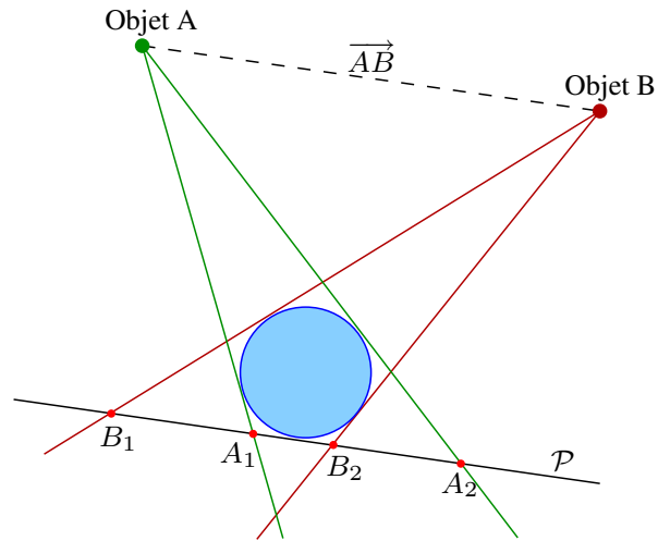
Figure 5.12 – Création de deux plans de rendu appartenant à un plan commun \mathcal{P} .
