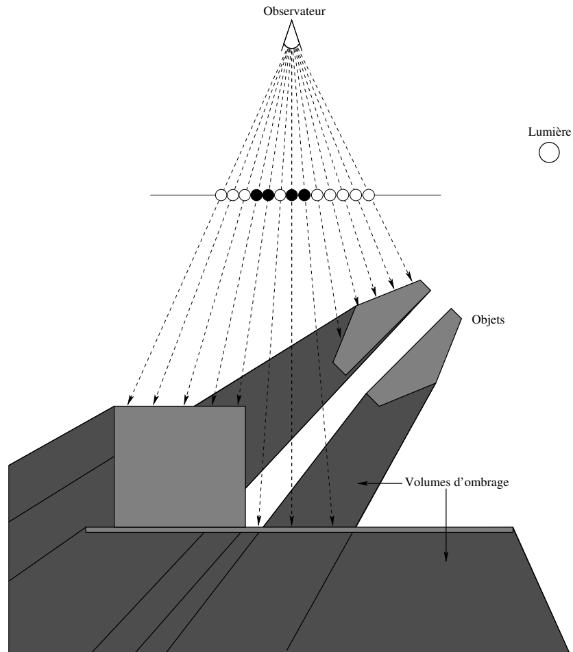
Figure 5.5 – Algorithme de calcul des volumes d'ombrage. La source lumineuse permet de définir les zones d'ombrage en fonction de la position des objets dans la scène. Afin de déterminer si un pixel est à l'ombre, il faut tester l'appartenance à un volume d'ombrage de l'intersection entre le rayon correspondant à ce pixel et la scène 3D. Si l'intersection appartient à un shadow volume , le point est à l'ombre, sinon il est éclairé.
