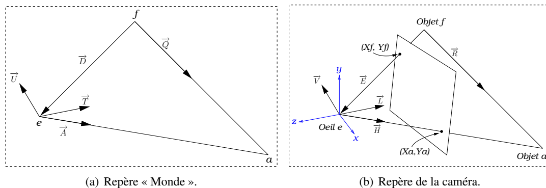
Figure 2.12 – Approche algébrique développée par Blinn pour le placement de caméra.
