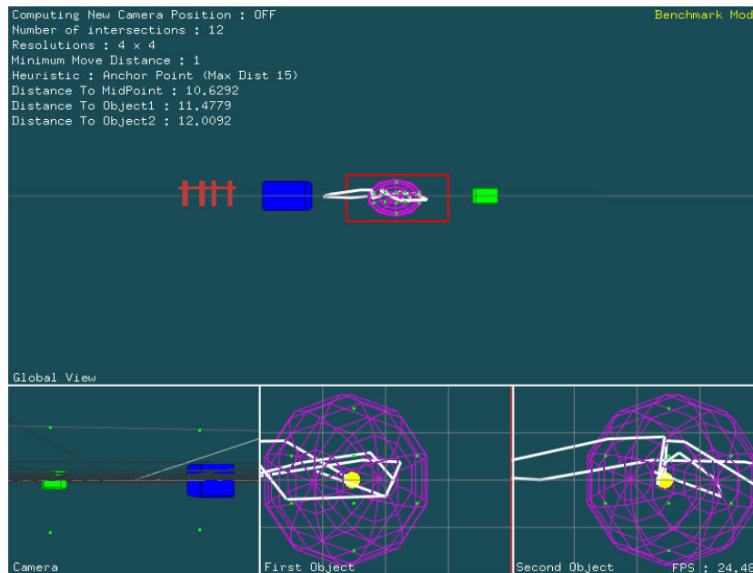
Figure 5.26 – Illustration de l'aller-retour d'un objet occultant devant les objets d'intérêt.
