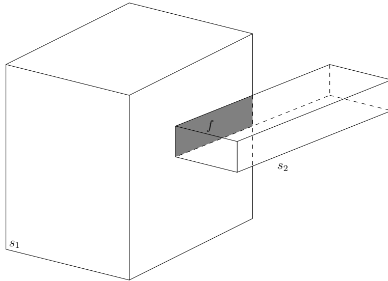
Figure 4.18 – Singularité résultant de l'application d'une opération booléenne à deux solides s_1 et s_2 représentés paramétriquement.
