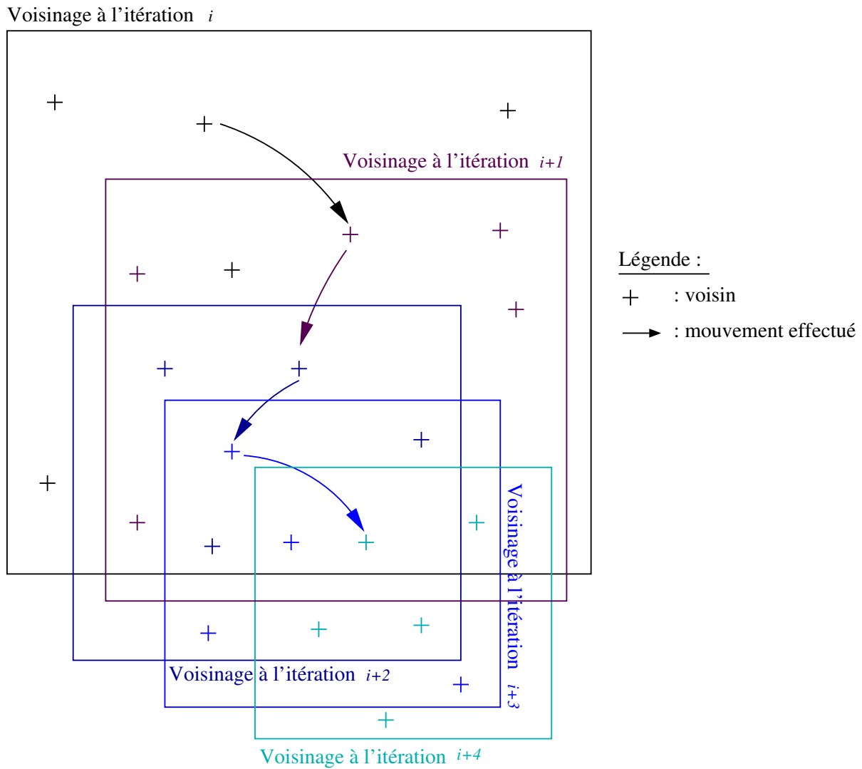
Figure 3.15 – Notions de voisinage, de génération de voisins, d' \alpha -réduction du voisinage et de mouvement d'une recherche locale adaptée aux intervalles à bornes flottantes.
