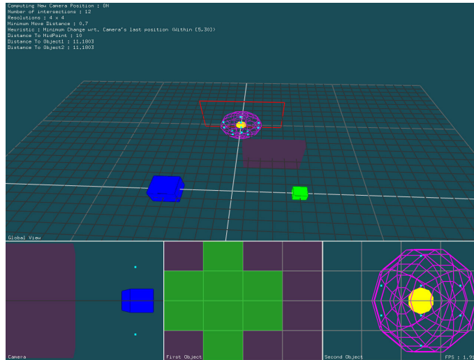
Figure 5.22 – Illustration d’une occultation de l’objet O_1 , représenté par un cube vert, dans le prototype OCCLUSION AVOIDER. Les points d’intersection appartenant à la sphère d’approximation sont affichés en bleu turquoise pour signaler que l’objet O_1 est occulté.
