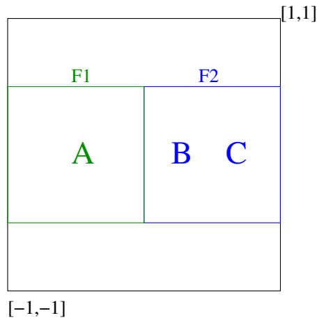
Figure 3.17 – Cadres mis en jeu dans le jeu de test de composition visuelle. Le cadre F1 doit contenir l'objet A , alors que B et C doivent appartenir à F2.
