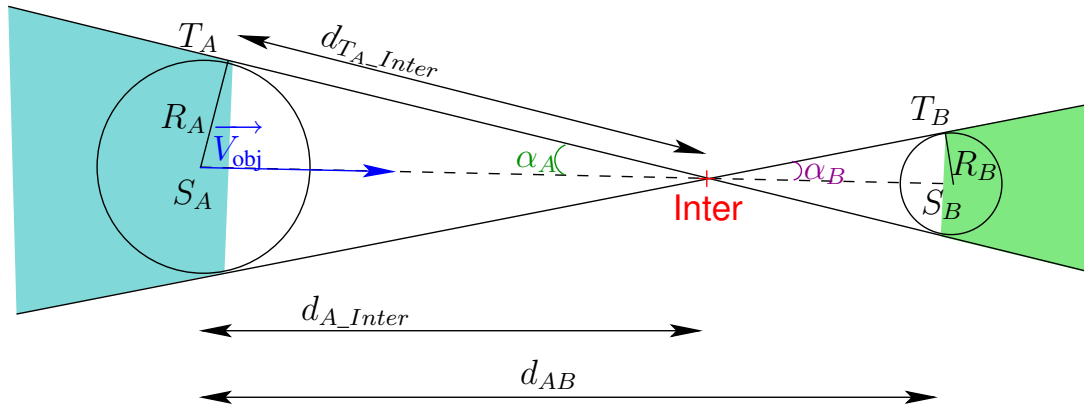
Figure 4.22 – Cônes d’occlusion partielle : les zones mises en évidence correspondent aux régions d’occlusion partielle d’un objet par un autre.
