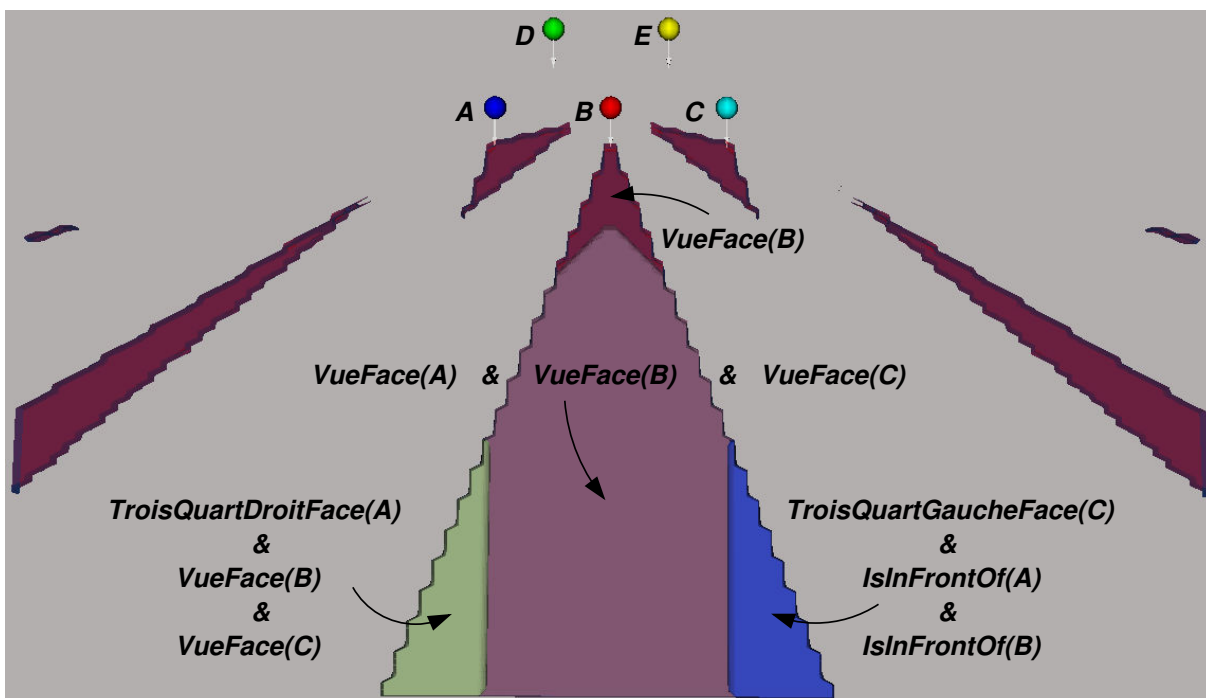
Figure 4.34 – Raffinements possibles d'une première description utilisateur.
