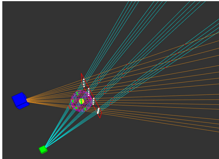
Figure 5.8 – Illustration du principe de l'OCCLUSION AVOIDER présentant les objets, le plan de rendu commun, les pixels de cet écran ainsi que les intersections calculées.
