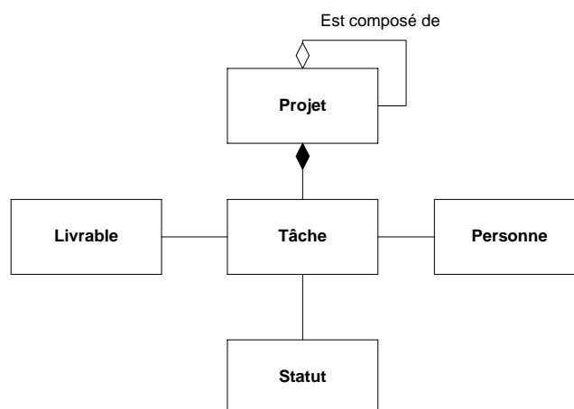
Figure 3-10: Modèle de données projet SMP
