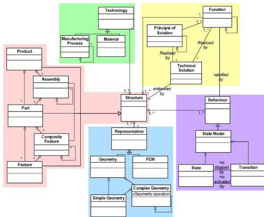
Figure 2-8: Modèle de produit de MOKA [MML 00]
