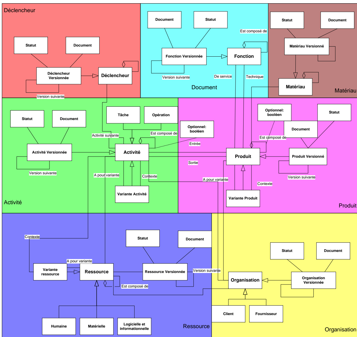
Figure 4-14: Diagramme de classes UML du modèle générique
