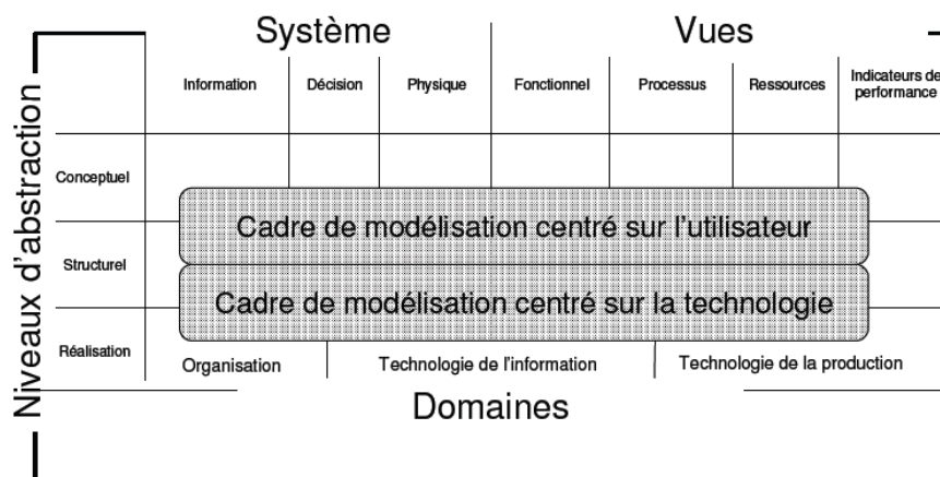
Figure 2-14: Cadre de modélisation de GIM [DOU 98]
