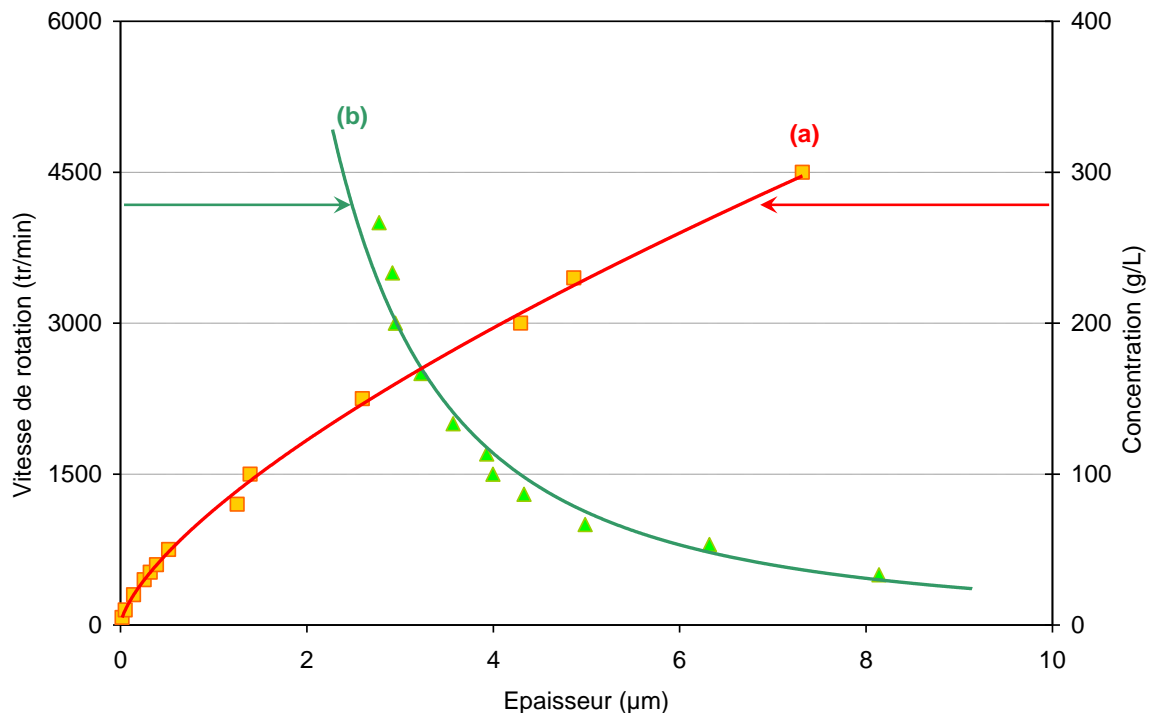
Figure 25 : Etude, sur l'épaisseur des films de PVCi, de : a) l'effet de la concentration de la solution à vitesse constante ( V = 1500 tr/min) ; b) l'effet de la vitesse de rotation de la tournette à concentration constante ( C = 230 g/L)
