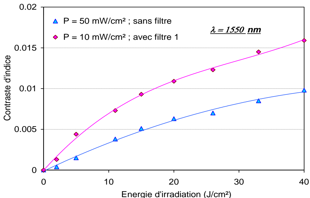
Figure 46 : Etude de la variation d'indice de réfraction, dans des films de PVCi de 5 µm, insolés avec et sans filtre
