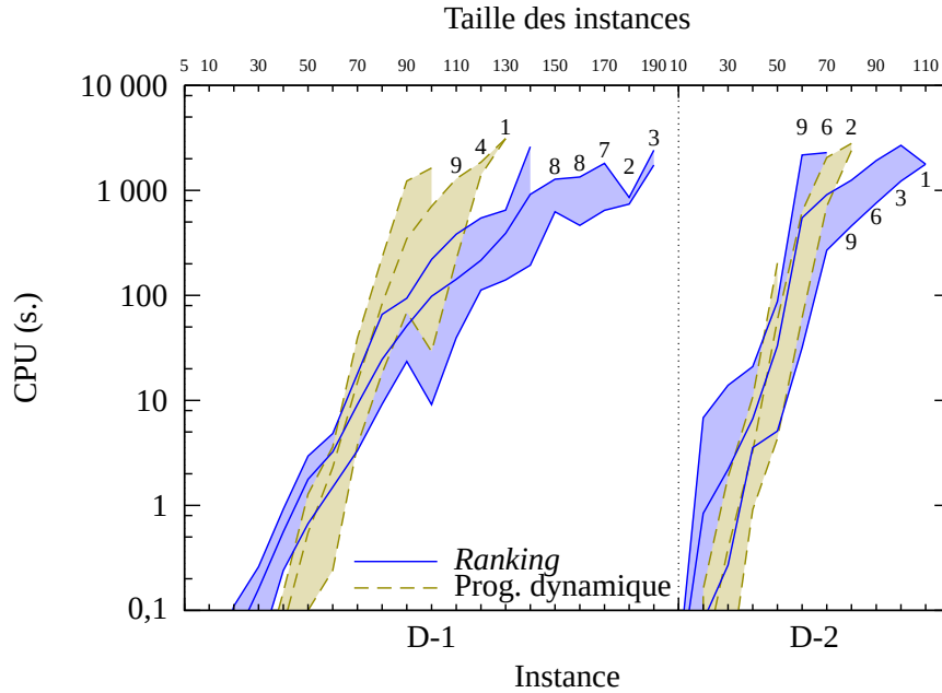
Figure 5.11 – Comparaison des temps de résolution minimaux, moyens et maximaux pour les instances du groupe D, obtenus avec la programmation dynamique de [10] et avec la procédure en deux phases utilisant un ranking . Le nombre d’instances résolues est indiqué lorsque certaines instances n’ont pas été résolues dans le délai d’une heure, pour une taille donnée. Les chiffres 9, 6 et 2 en haut à droite concernent la programmation dynamique.
