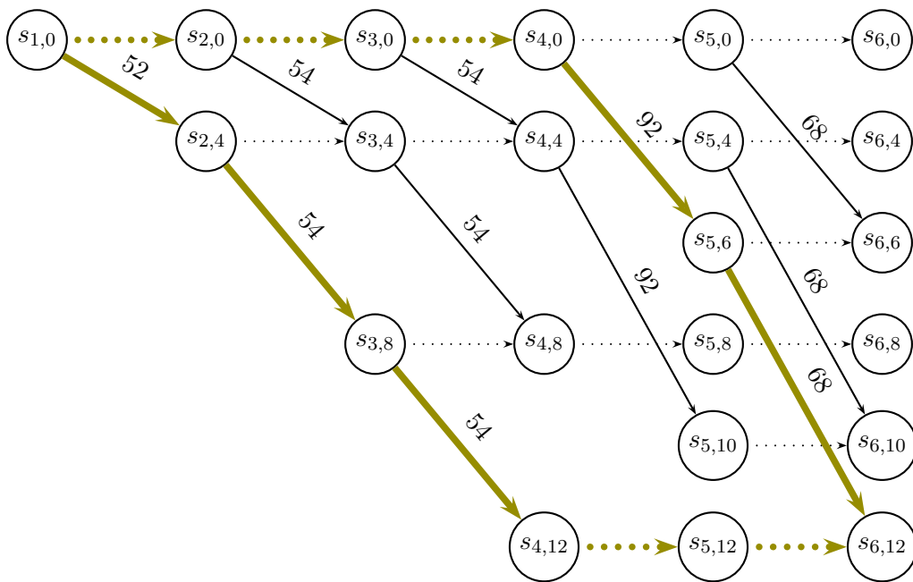
Figure 4.5 – Graphe associé à l’instance de l’exemple 4.14. La valeur indiquée au dessus des arcs est leur poids. Les arcs en pointillés ont un poids nul, non indiqué pour plus de lisibilité. Les chemins de l’ensemble \varphi(s_{6,12}) sont mis en évidence.
