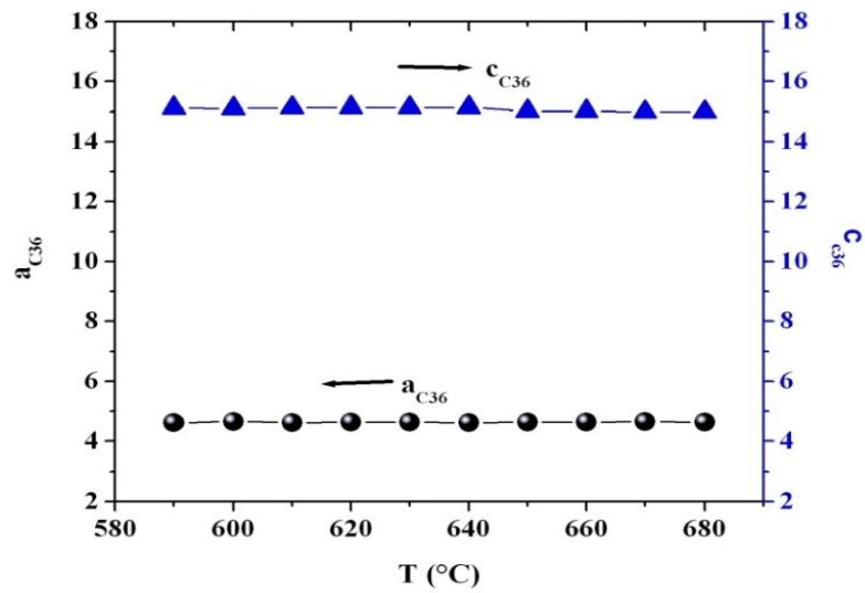
Figure III.24: Variation des paramètres de la maille hexagonale de Mg_2Sn C36 ( T > 590^\circ C )
