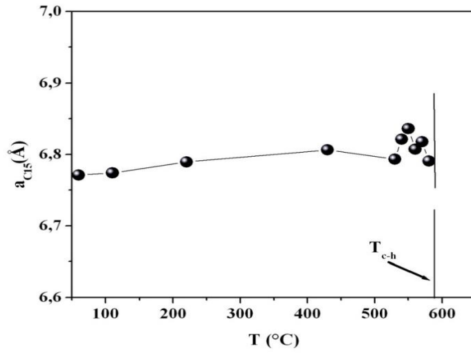
Figure III.23: Variation des paramètres de la maille cubique de Mg_2Sn C15 ( T < 590^\circ C )
