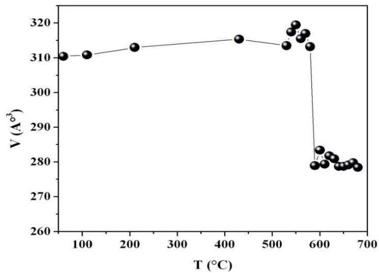
Figure III.25: Variation du volume de la maille de Mg_2Sn en fonction de la température
